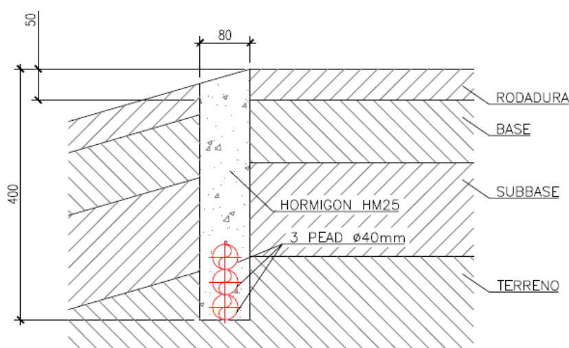
SECCION MICROZANJA EN BERMA COTAS EN mm.
