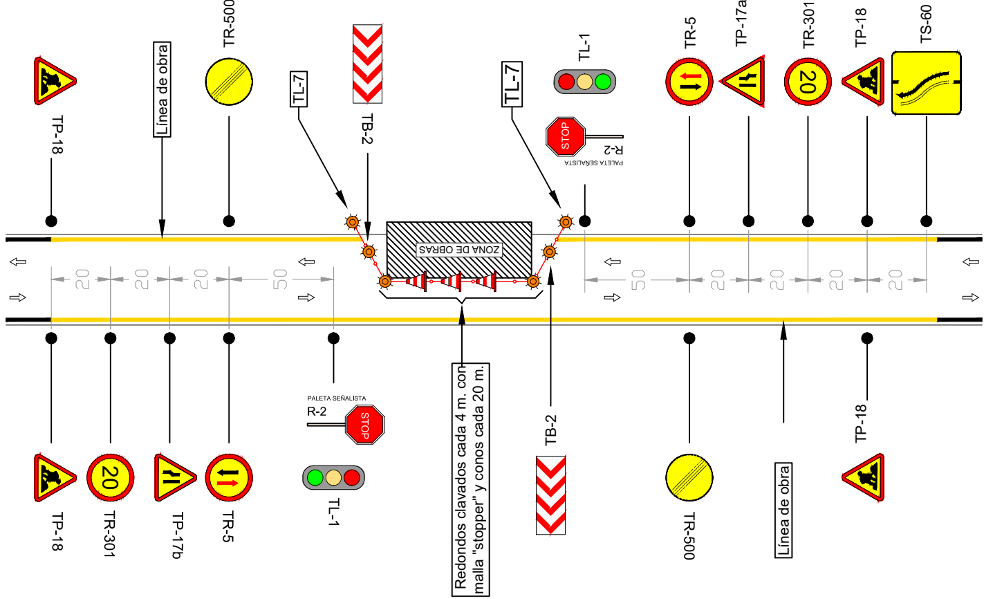
DETALLE DE CRUCE DE CARRETERA PRIVADA CON INTERRUPCIÓN TEMPORAL DE UN CARRIL.
