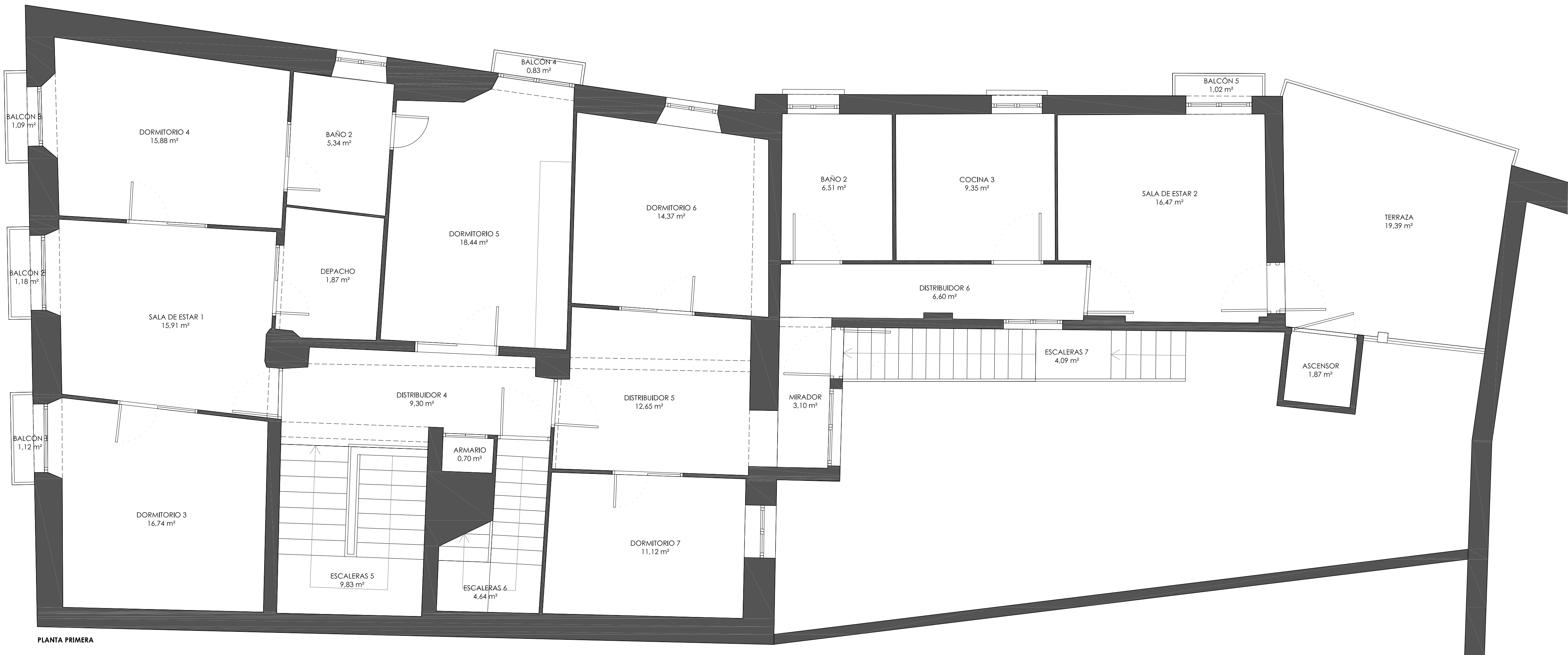
PLANTA PRIMERA
