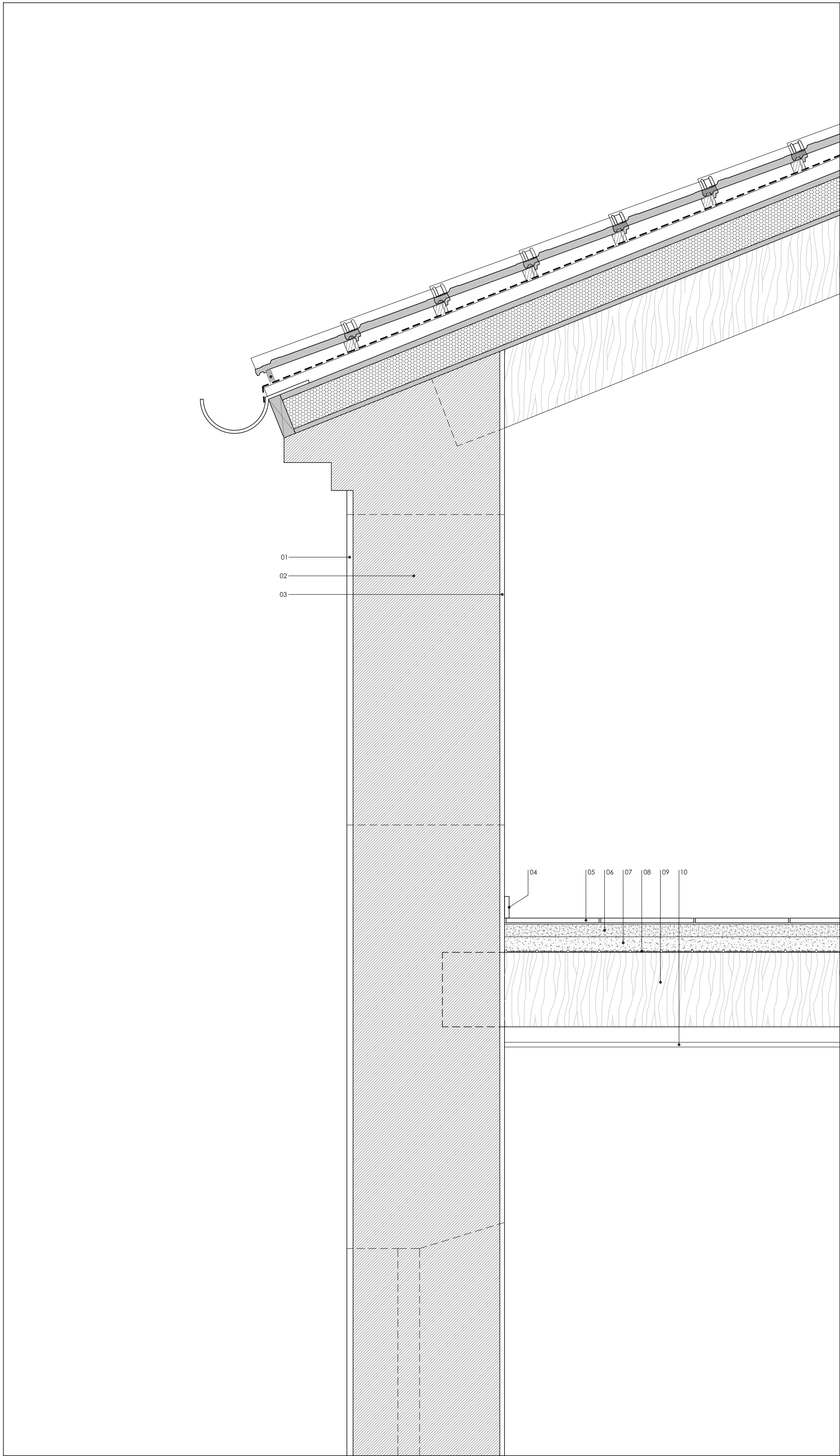
DETALLE CONSTRUCTIVO 1
