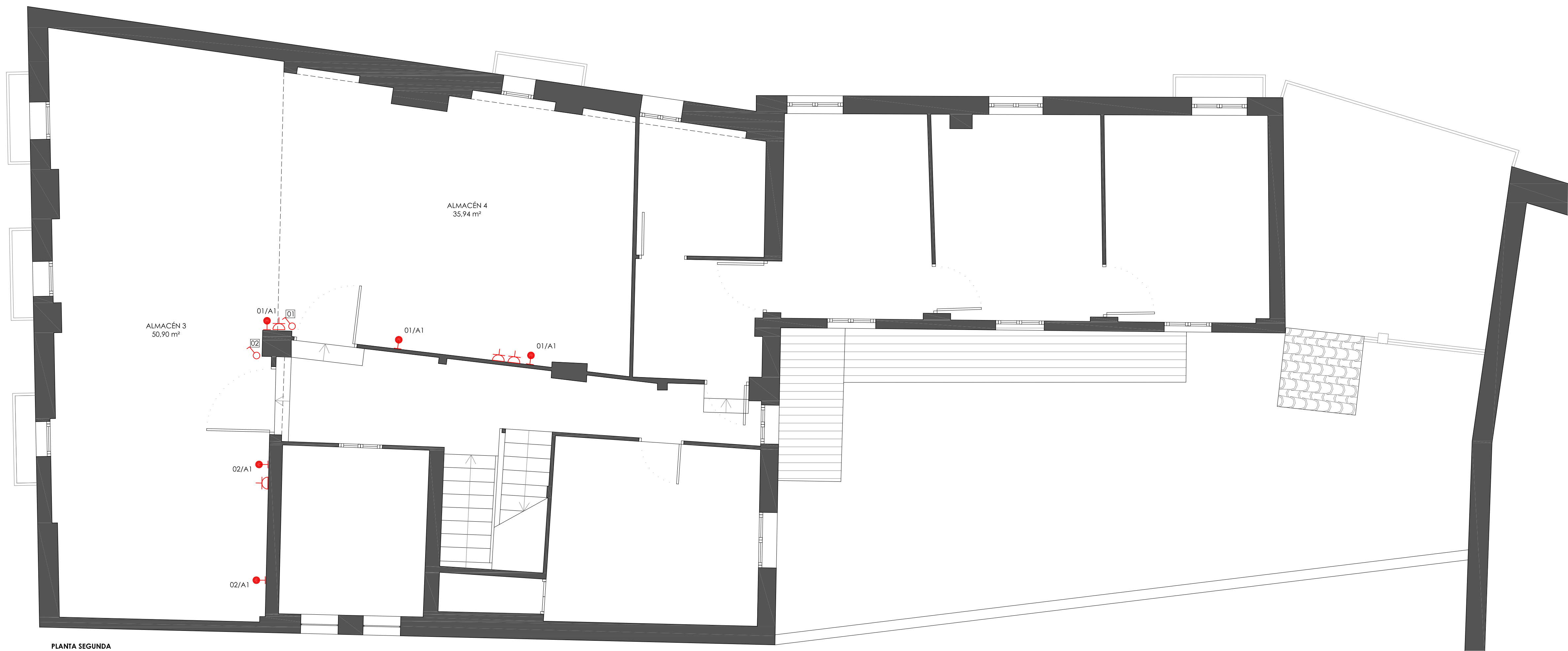
PLANTA SEGUNDA
