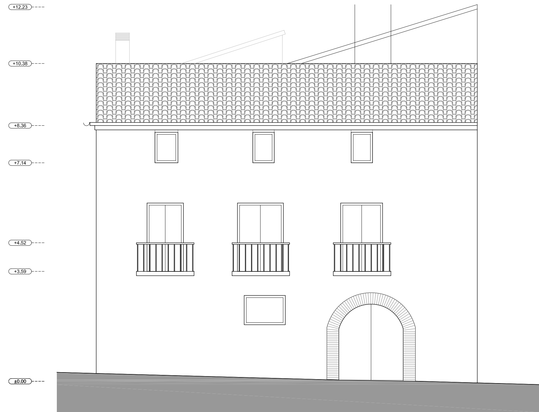
ALZADO OESTE
