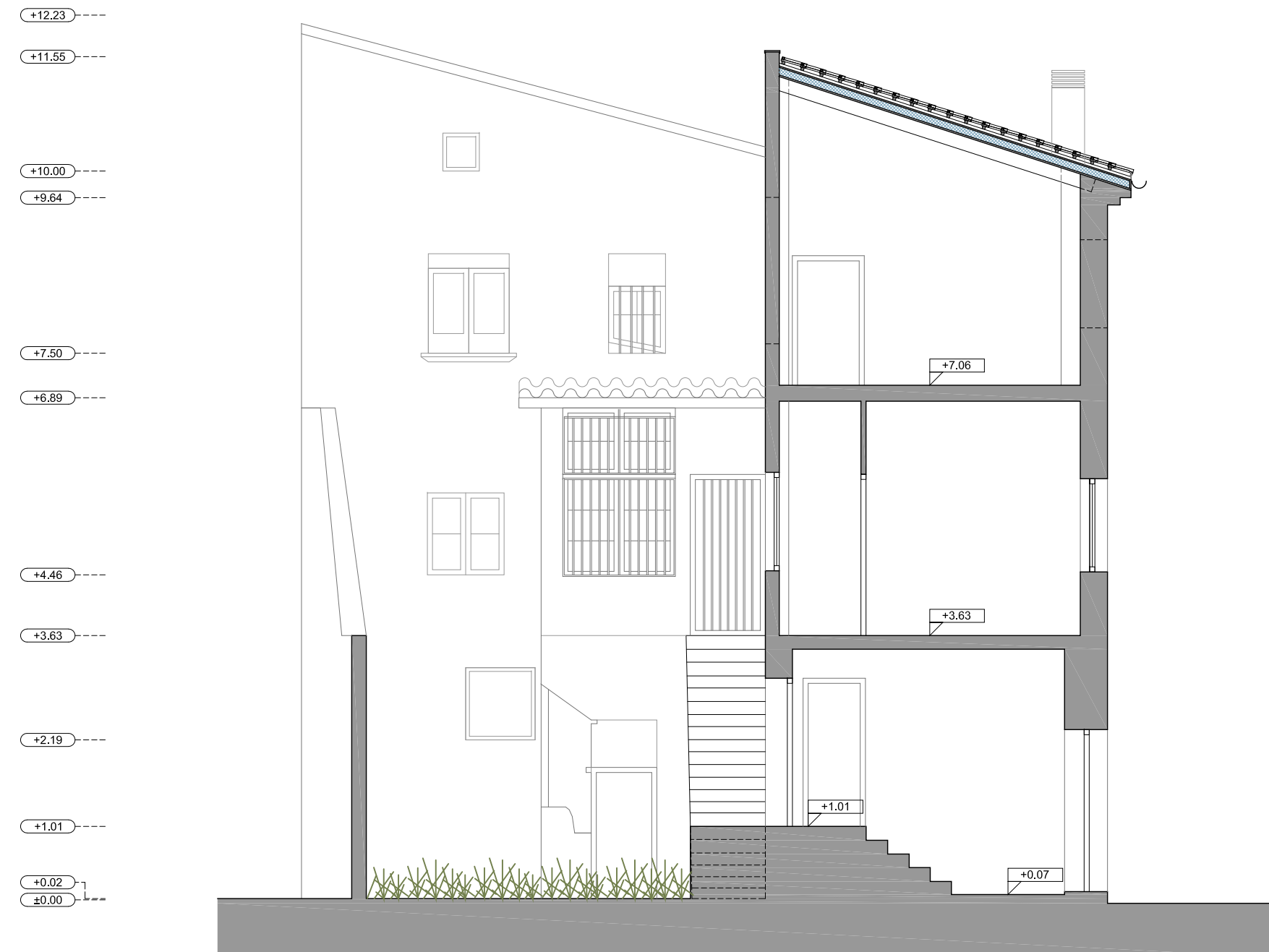
SECCIÓN B
