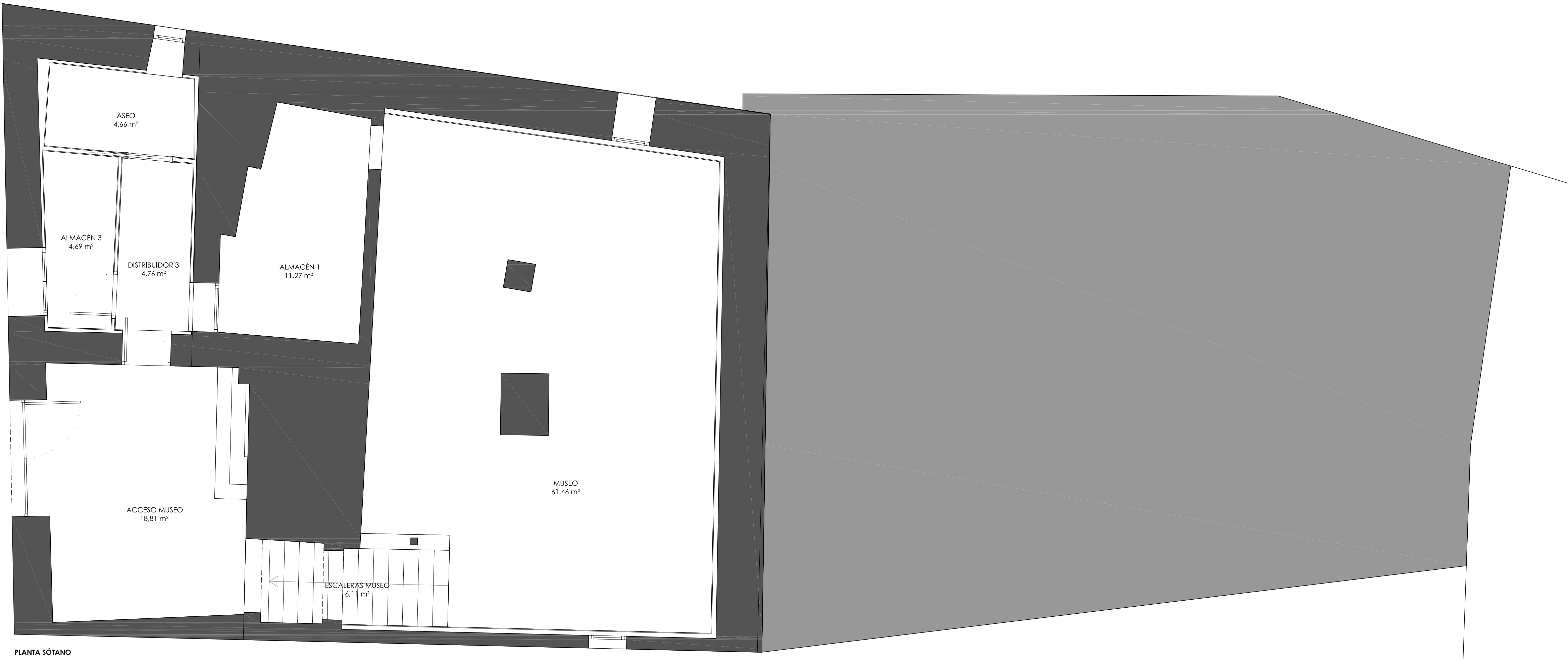
PLANTA SÓTANO
