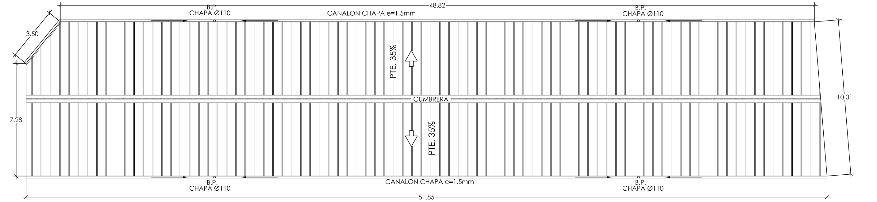
PLANTA CUBIERTA PANEL SANDWICH GRECADO 60mm REMATES PERIMETRALES e=0,7mm
