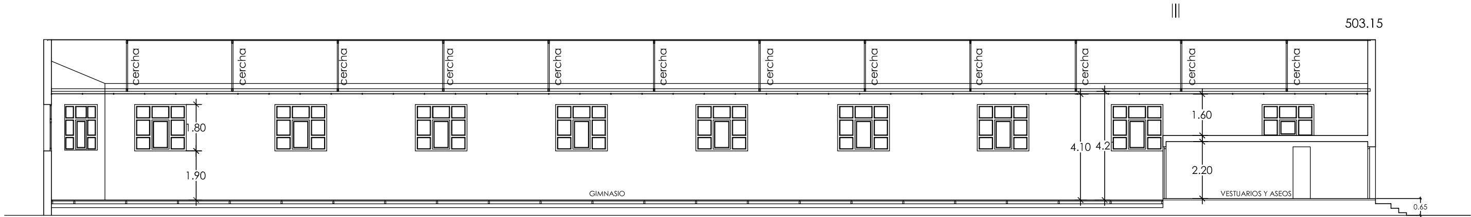
SECCION A-A' 1/150
