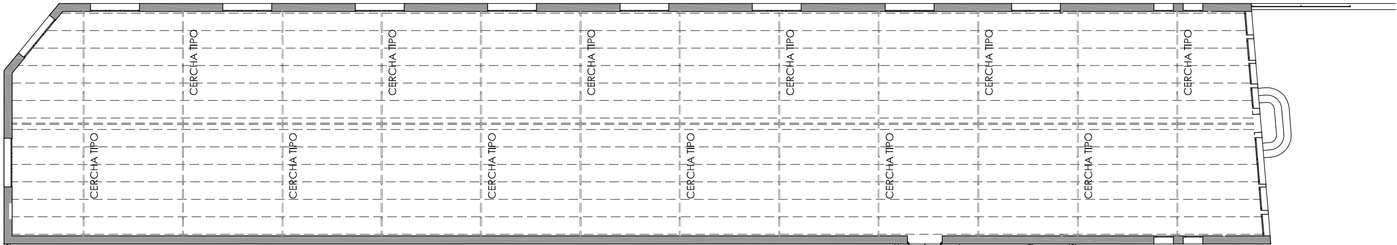
PLANTA ESTRUCTURA CERCHAS Y CORREAS 1/150
