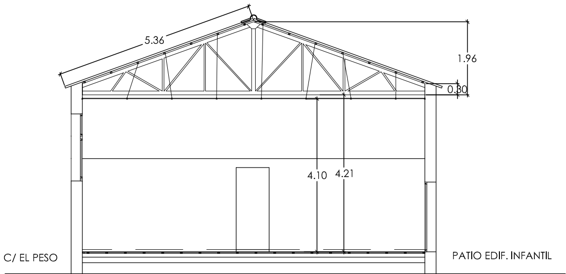
SECCION B-B' 1/100
