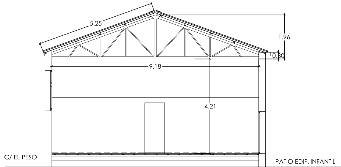
SECCION B-B' 1/100
