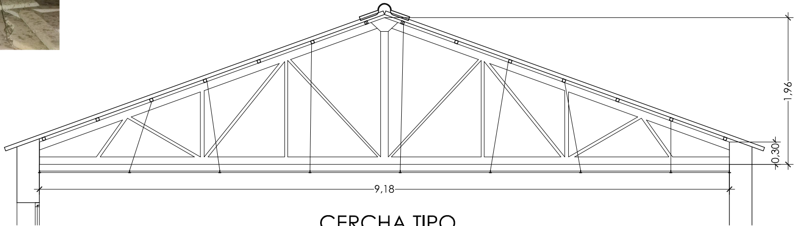
CERCHA TIPO 1/50
