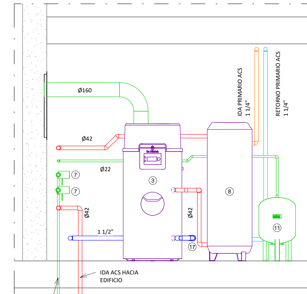
SECCIÓN ACS 1 : 25
