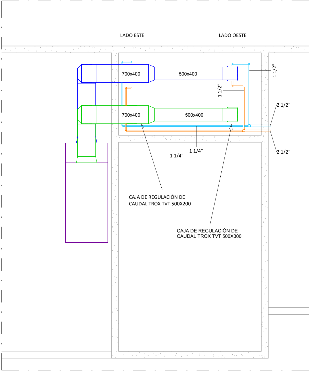
1 CUBIERTA 1 : 75
