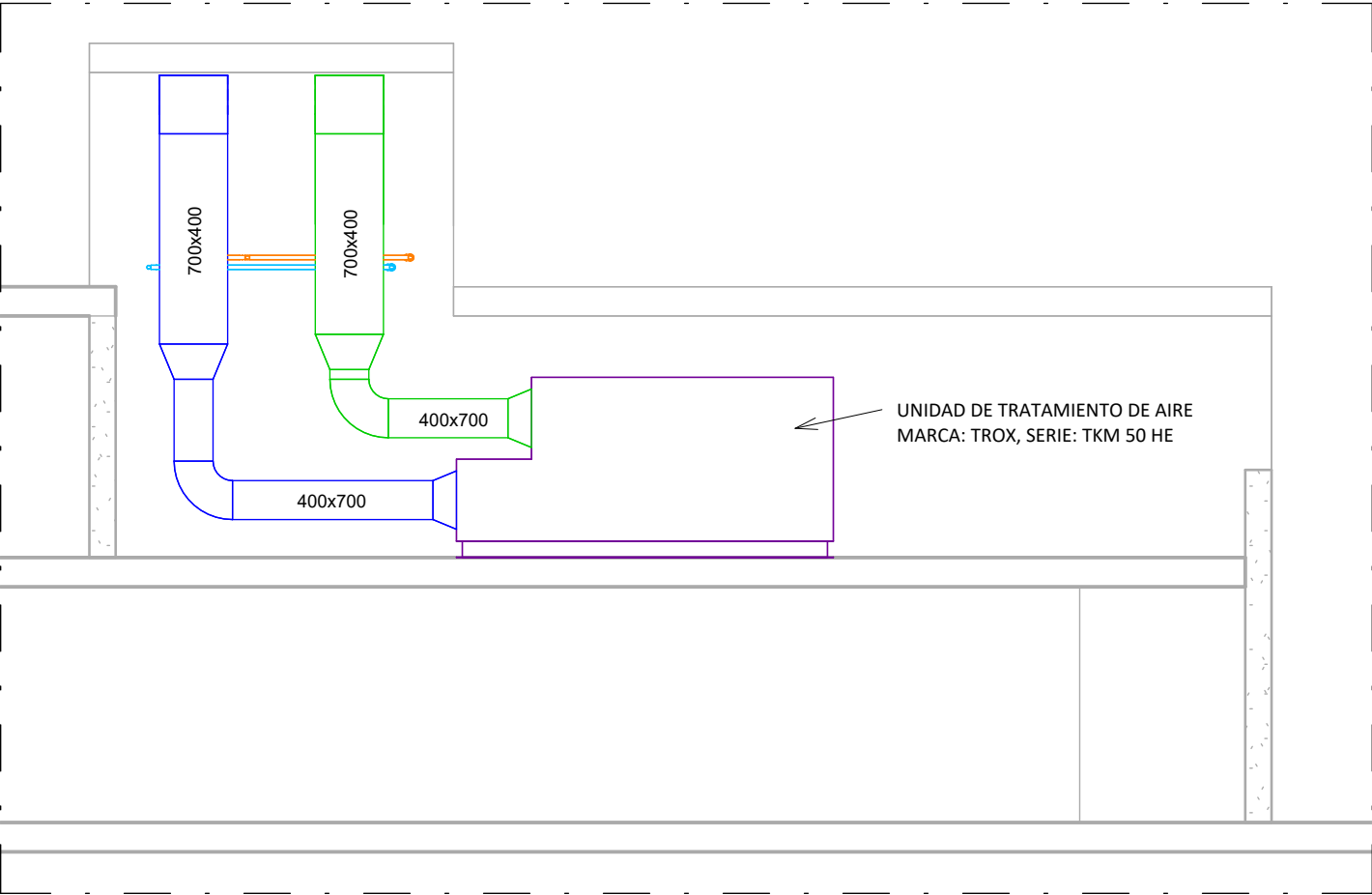
3 SECCIÓN TRANSVERSAL AIRE 1 : 75
