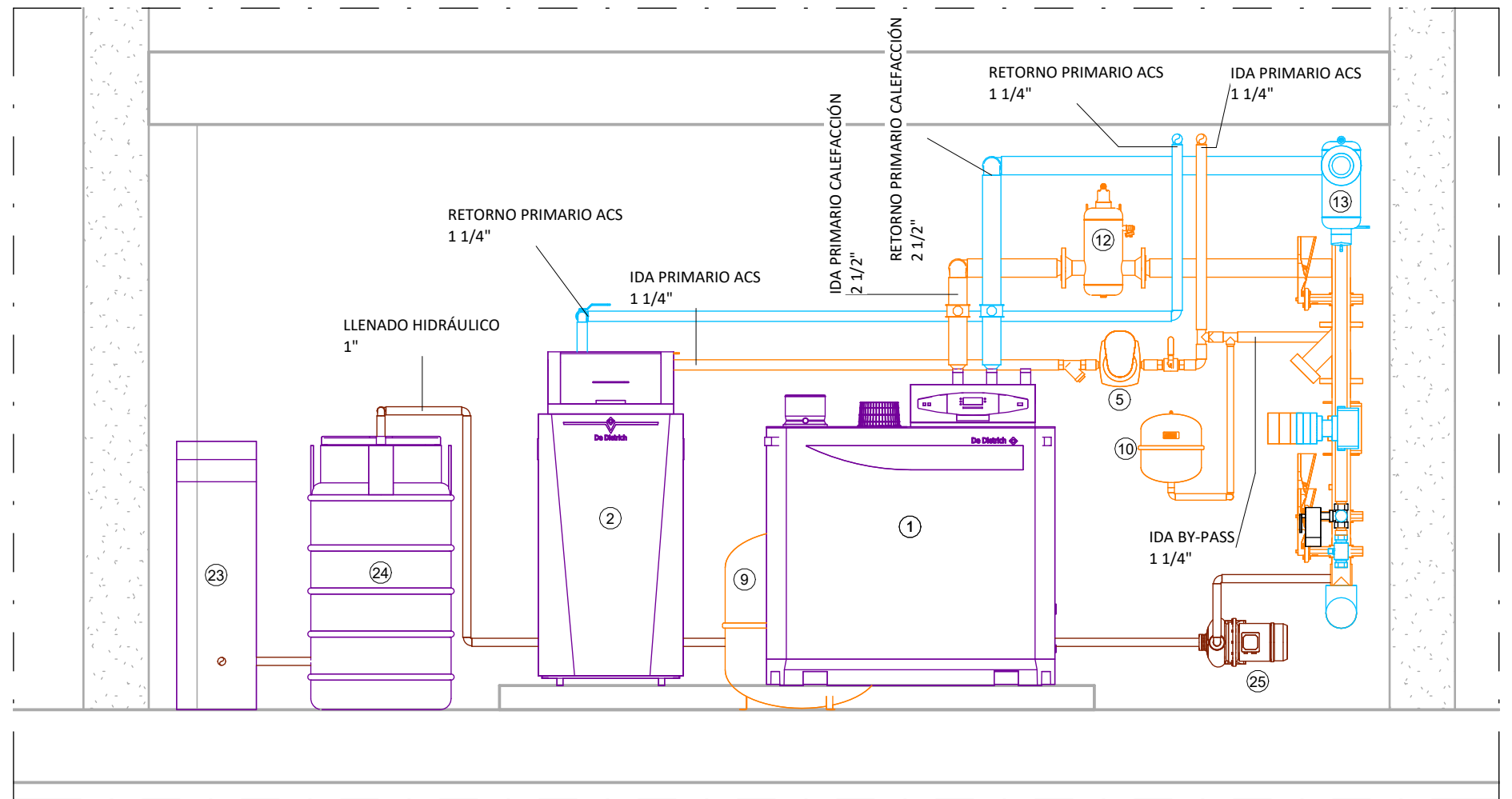
SECCIÓN CALDERAS 1 : 25
