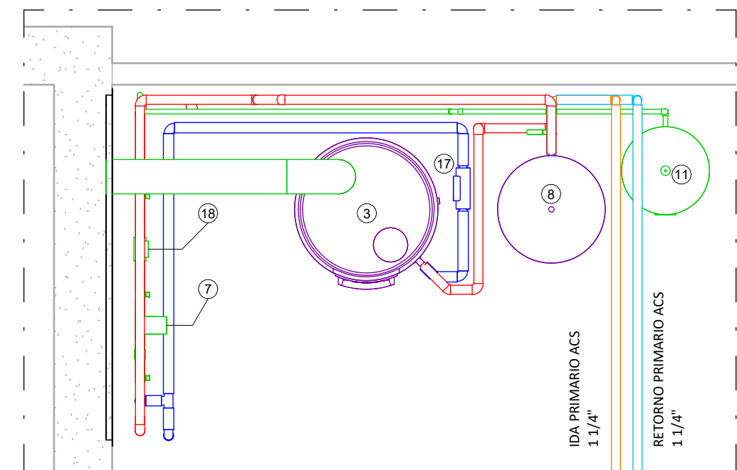
PLANTA ACS 1 : 25
