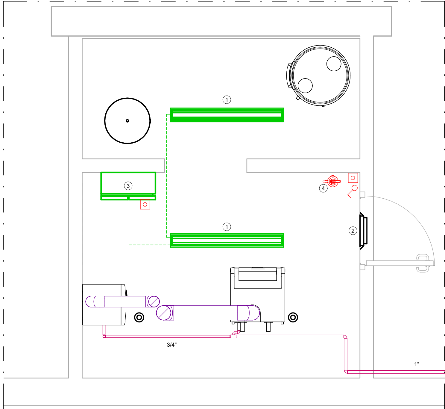
1 PLANTA SALA DE CALDERAS OBRA CIVIL
