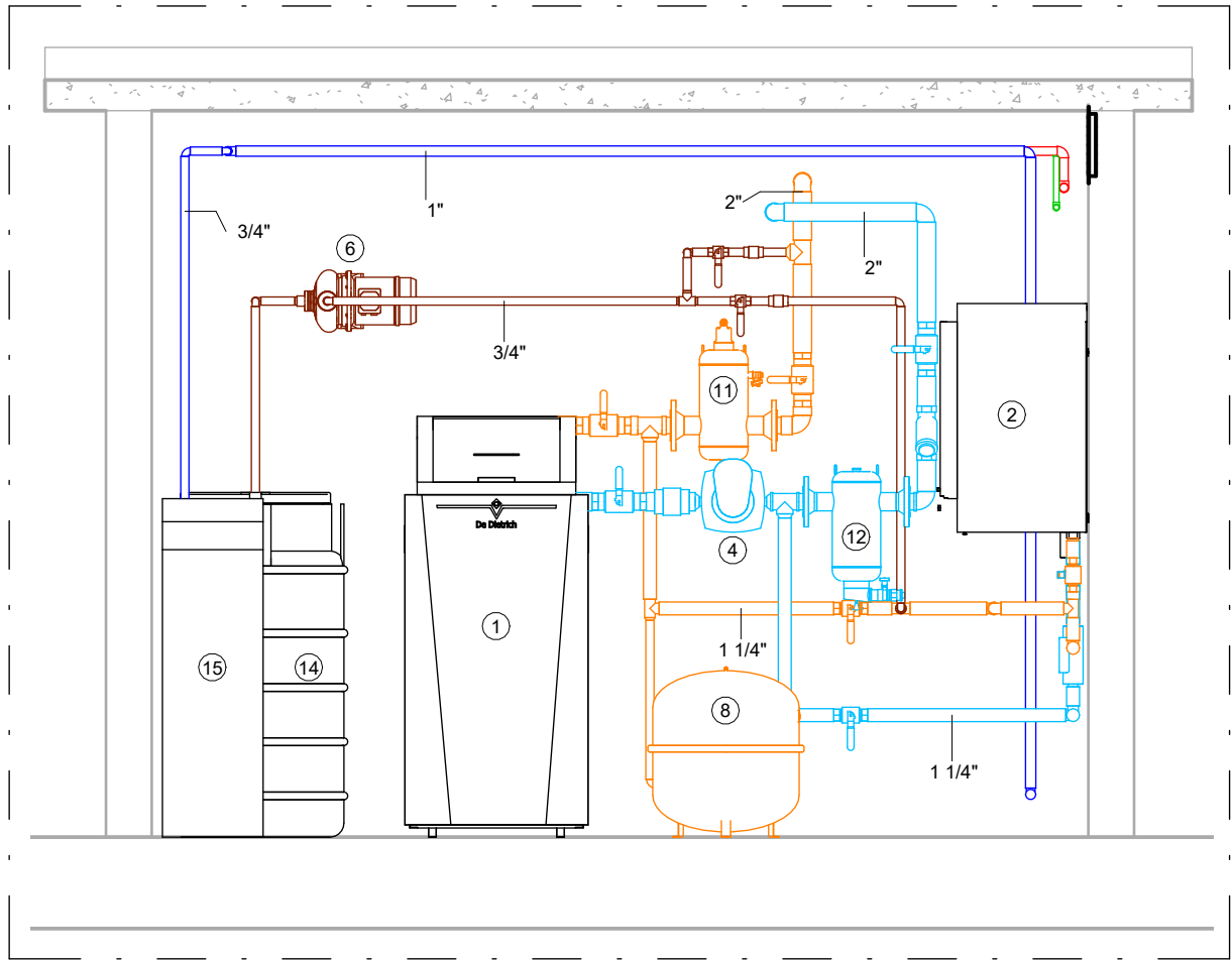
2 SECCIÓN CALDERA CALEFACCIÓN 1 : 25
