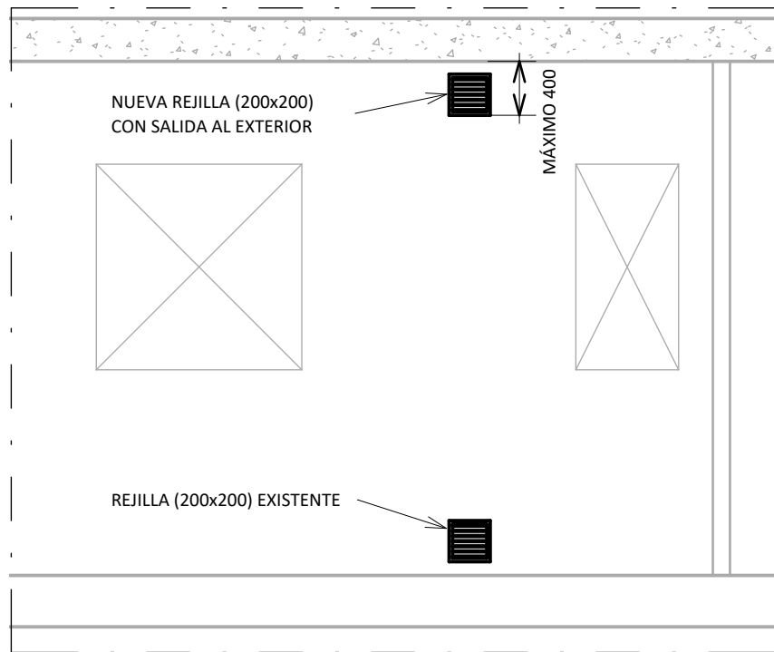
3 SECCIÓN VENTILACIÓN COCINA 1 : 40
