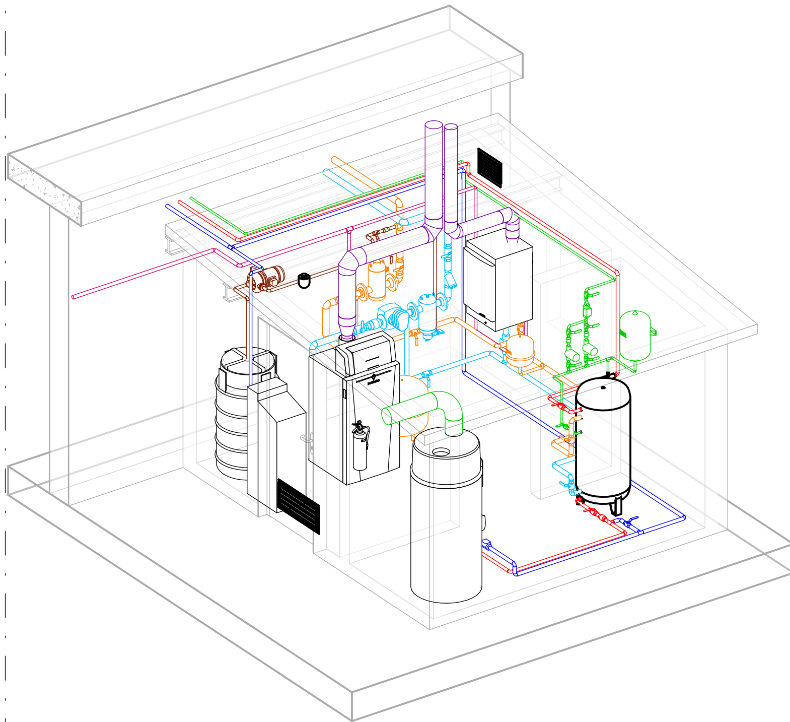
② 3D MECÁNICA SALA DE CALDERAS
