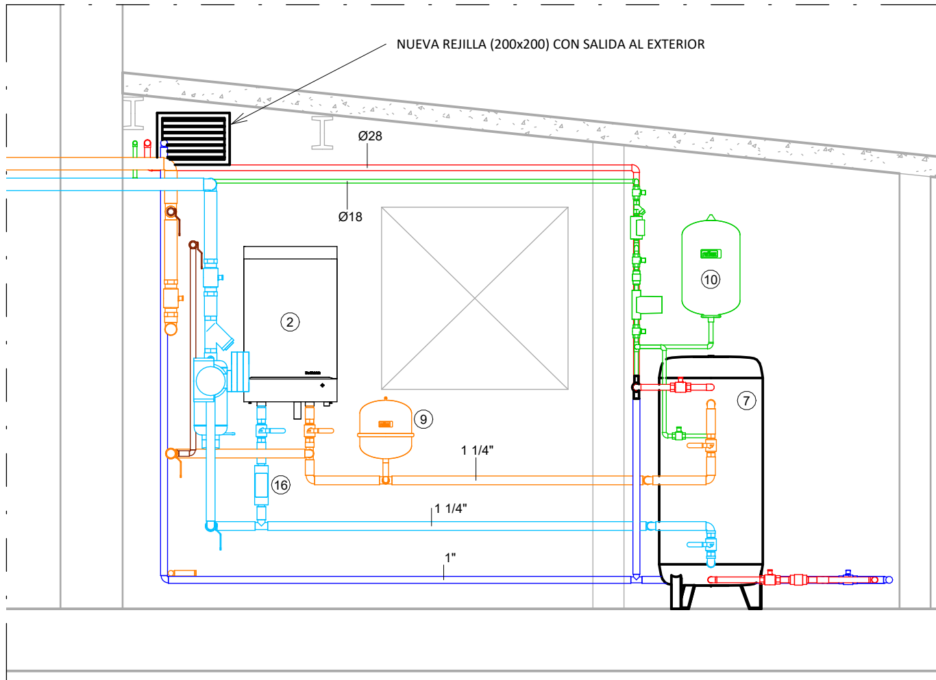
1 SECCIÓN CALDERA ACS 1 : 25
