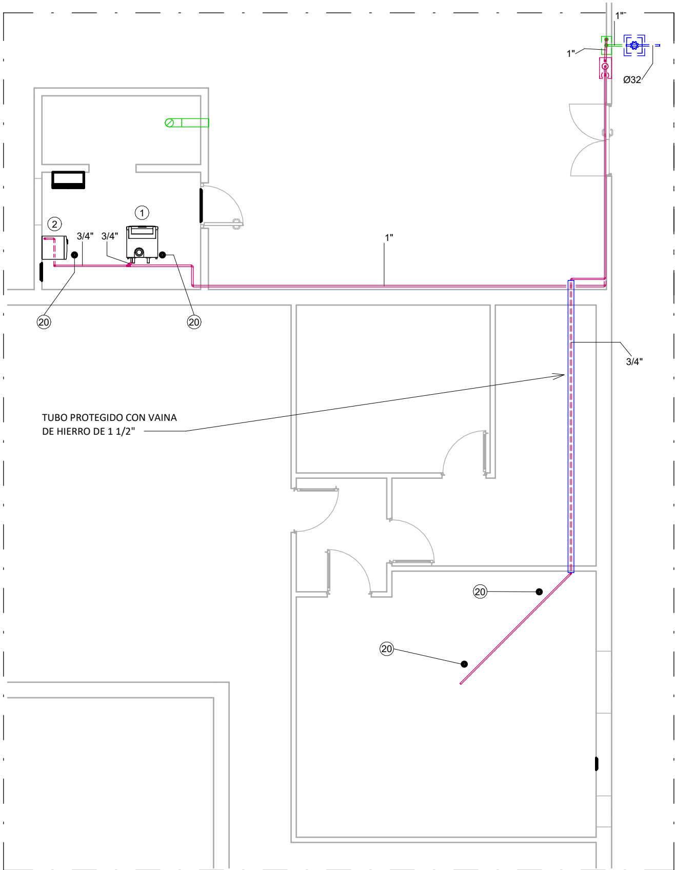
1 ACOMETIDA DE GAS 1 : 75
