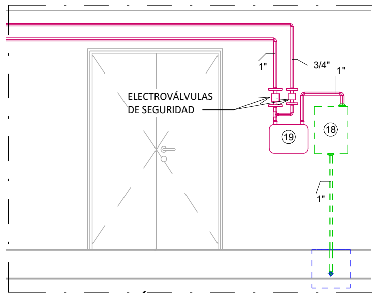
2 SECCIÓN ARMARIO GAS 1 : 40
