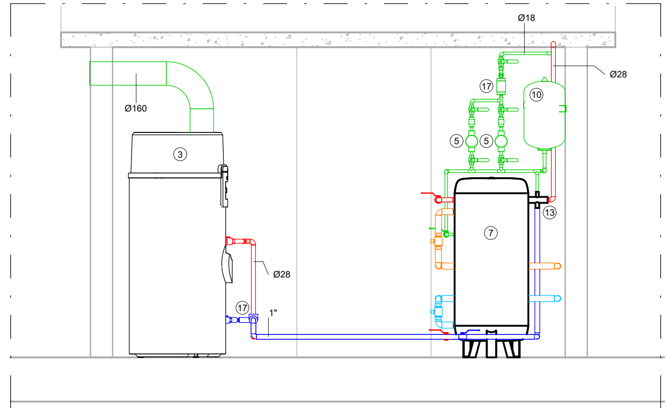
2 SECCIÓN ACUMULACIÓN ACS 1 : 25
