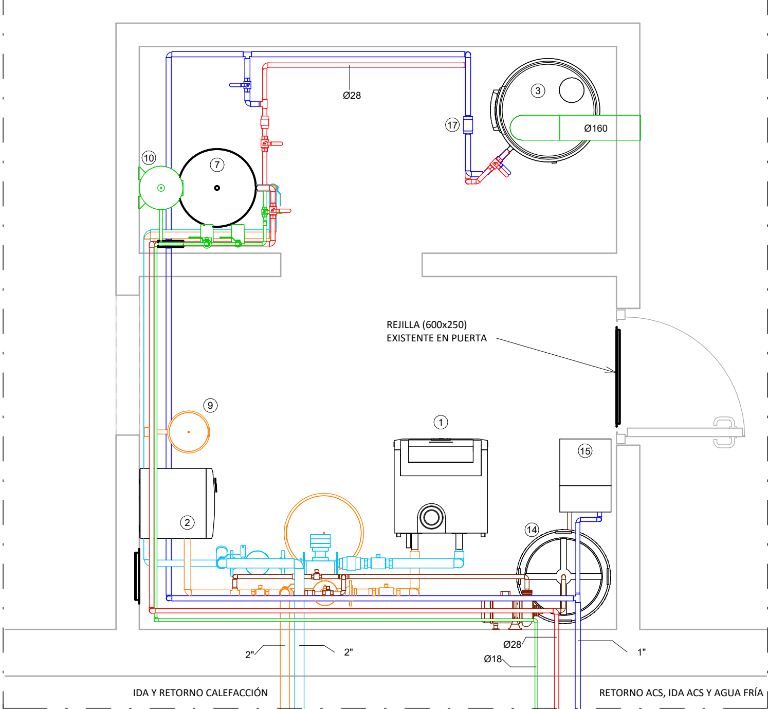
1 PLANTA SALA DE CALDERAS 1 : 25
