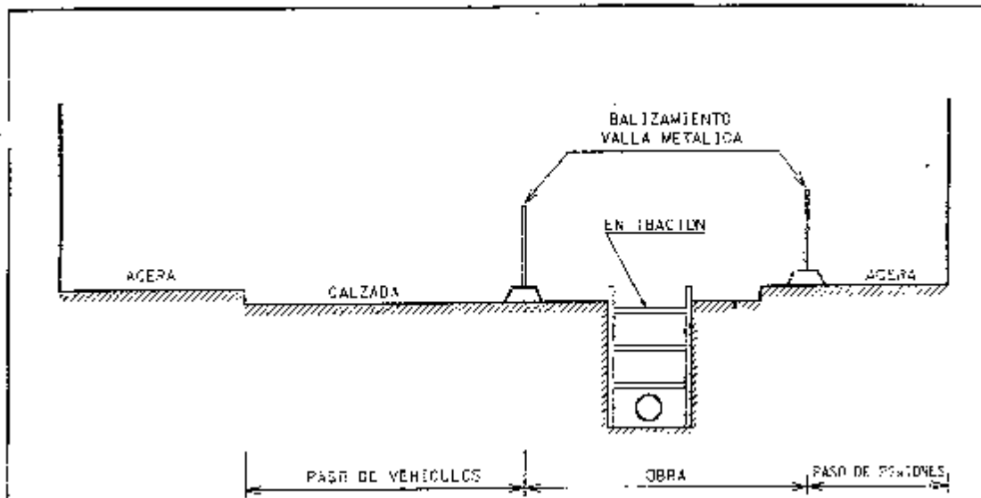
APERTURA DE ZANJA CON ENTIBACION EN CALZADA
