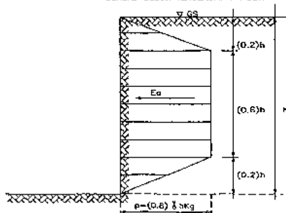
DIAGRAMA DE PRESIONES PARA ARENAS DENSAS O MEDIO DENSAS SEGUN TERGAZCHI Y PECK
