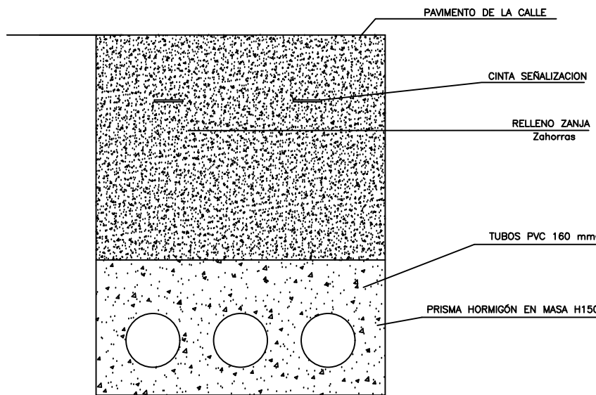
ZANJA BAJA TENSIÓN 3 TUBOS EN CALZADA
