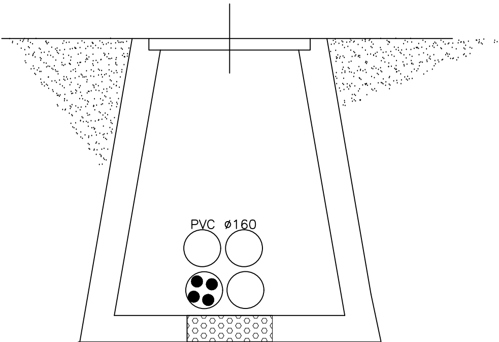
ARQUETAS MEDIA Y BAJA TENSIÓN LÍNEA SUBTERRANEA ALZADO
