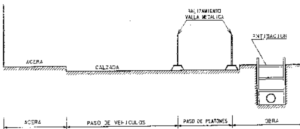
APERTURA DE ZANJA CON ENTIBACION EN ACERA
