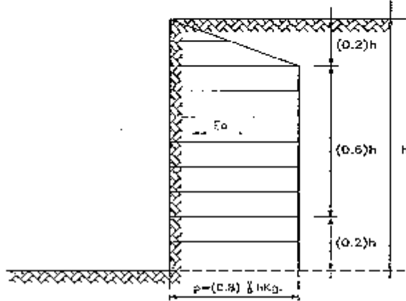
DIAGRAMA DE PRESIONES PARA ARCILLA
