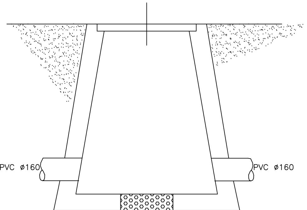
ARQUETAS MEDIA Y BAJA TENSIÓN LÍNEA SUBTERRANEA PERFIL
