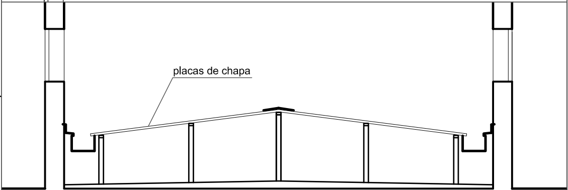
SECCION B-B' - E:1/50
