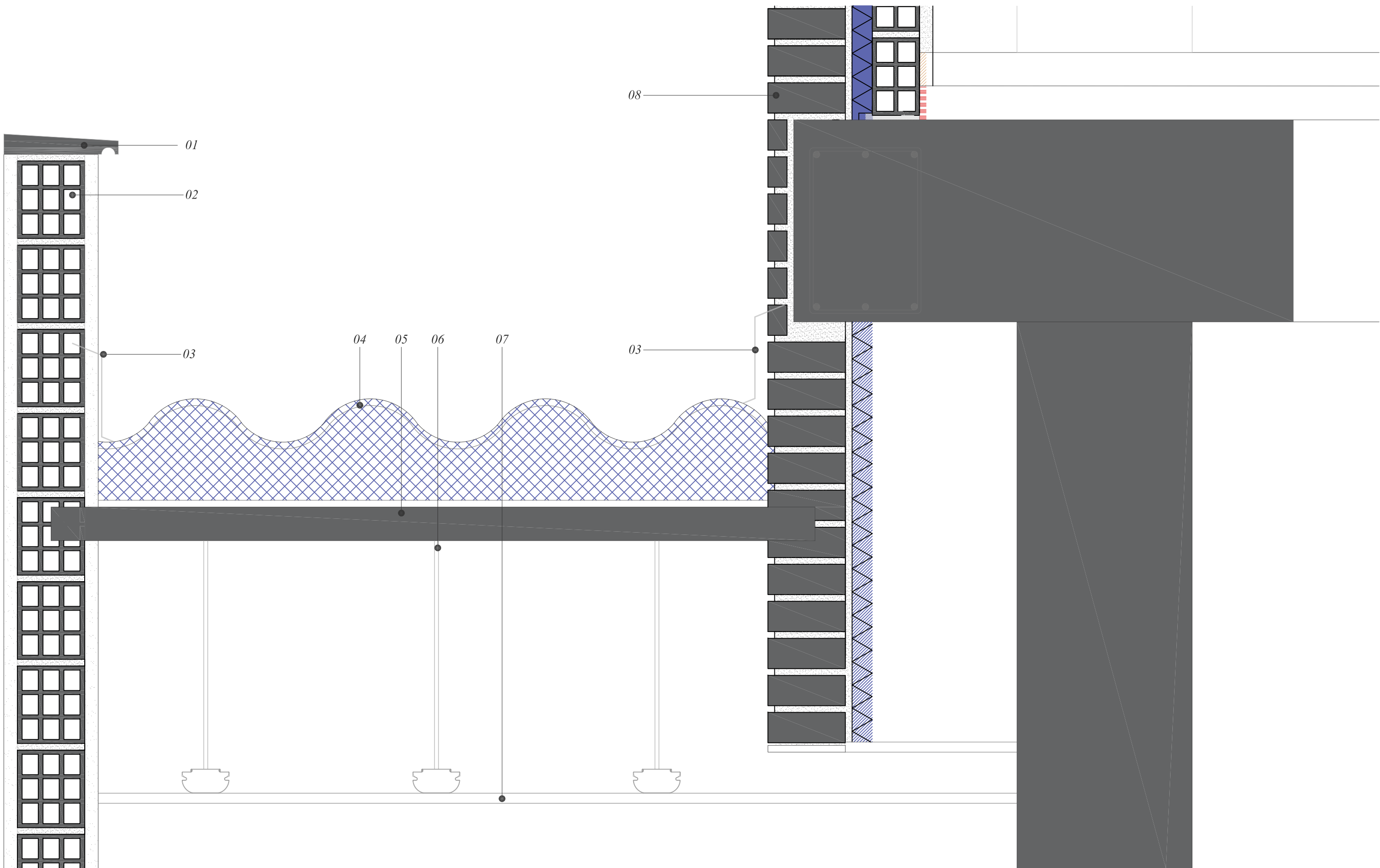
ESTADO REFORMADO - DETALLE CONSTRUCTIVO 1/15
