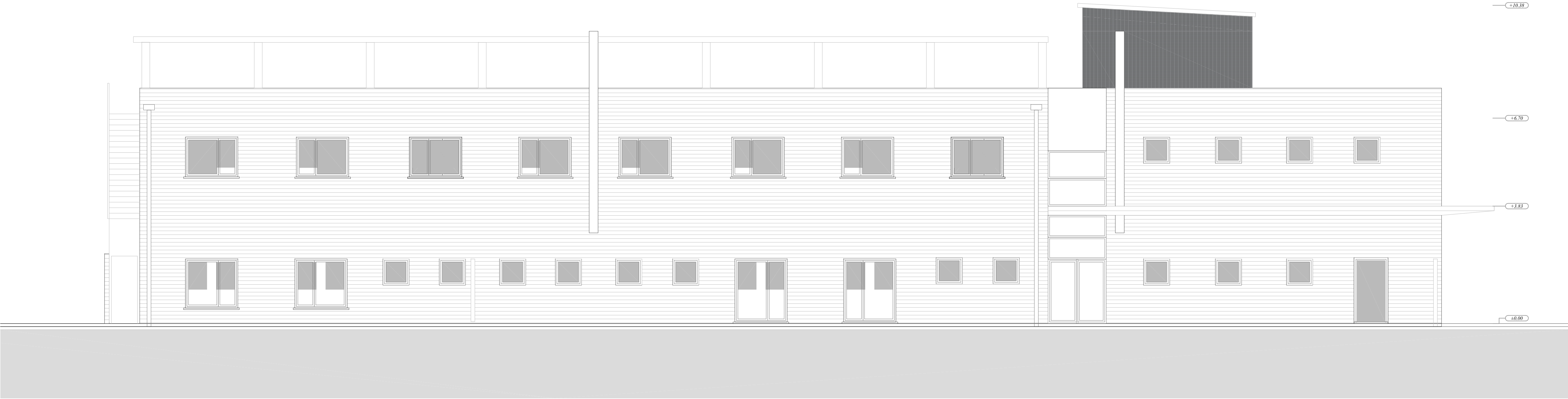
1 ESTADO ACTUAL - ALZADO LONGITUDINAL 1/75
