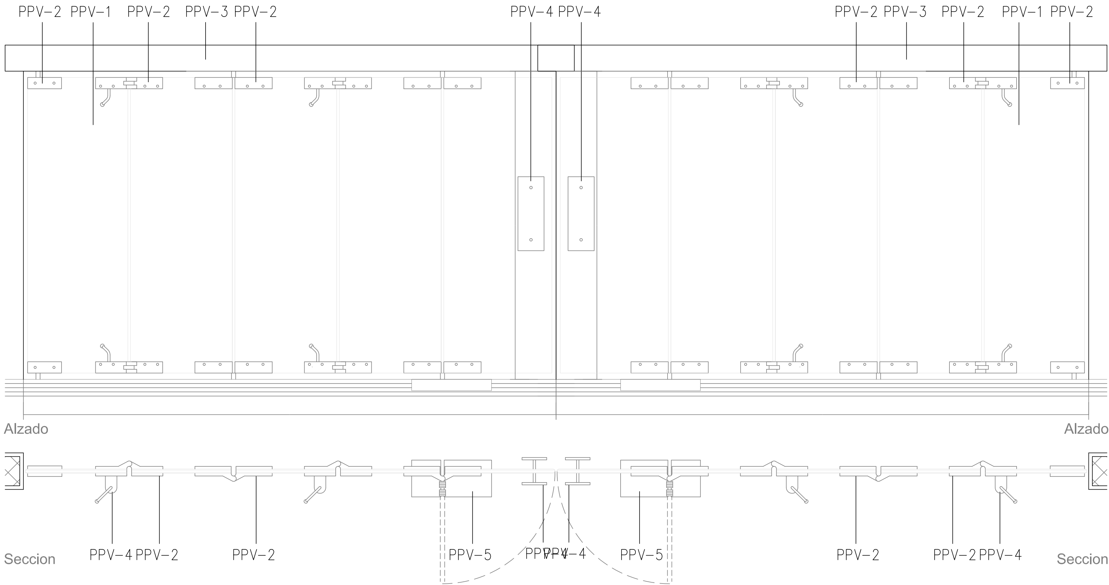
ESTADO REFORMADO - ALZADO PUERTA PLEGABLE 1/20
