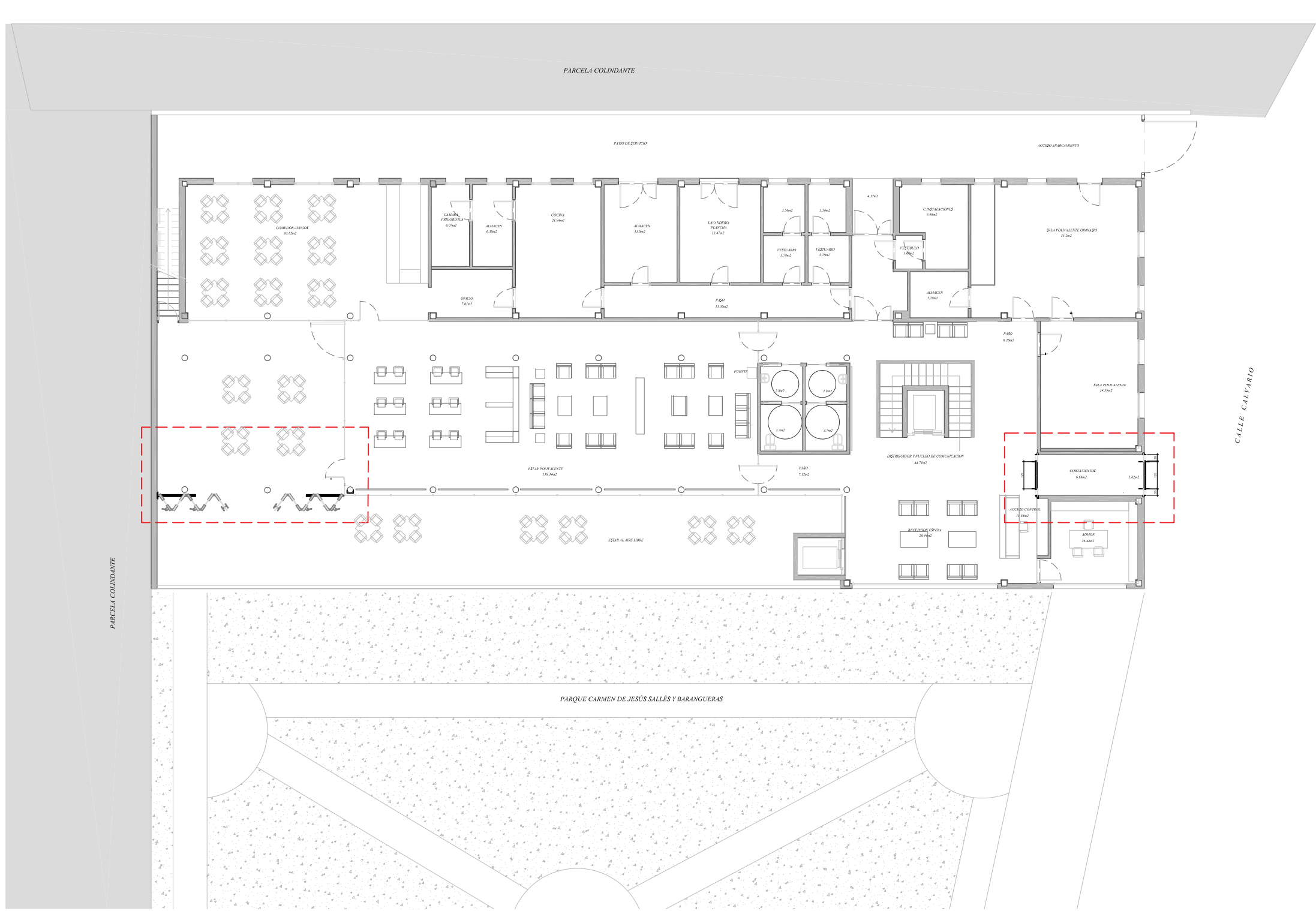
ESTADO REFORMADO - PLANTA BAJA GENERAL 1/300
