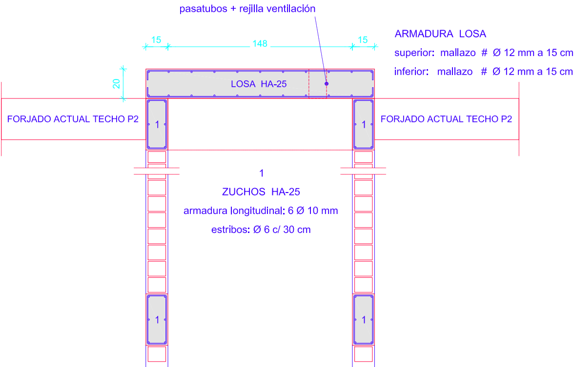
LOSA CIERRE SUPERIOR HUECO ASCENSOR. SECCIÓN VERTICAL
