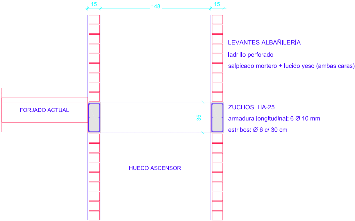
SECCIÓN TIPO HUECO ASCENSOR
