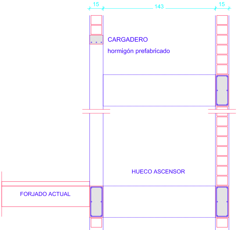
CABEZAL PUERTA ASCENSOR. SECCIÓN VERTICAL
