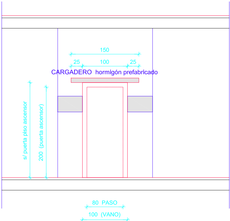
CABEZAL PUERTA ASCENSOR. ALZADO
