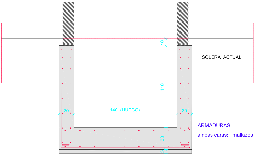
SECCIÓN DE FOSO
