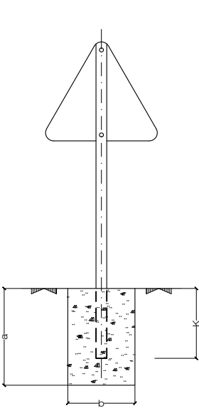
SEÑAL TRIANGULAR
