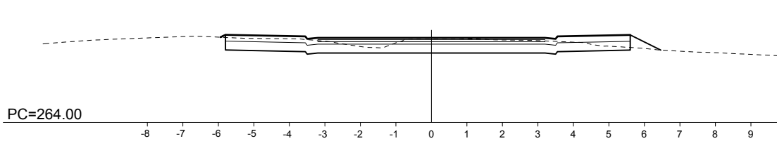
P.K.= 0+290
