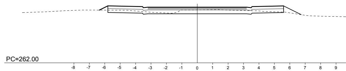
P.K.= 0+260
