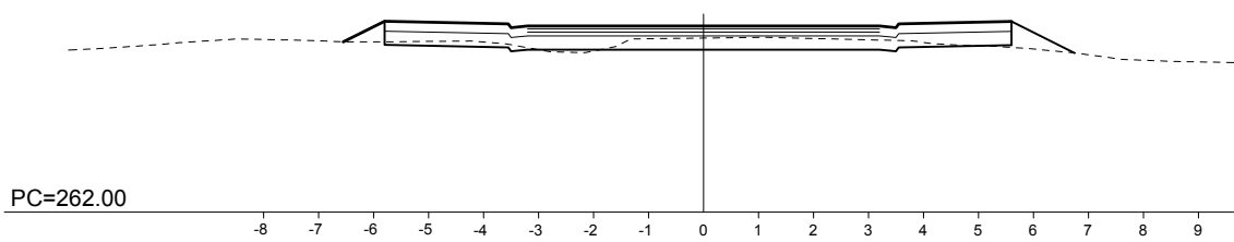
P.K.= 0+250
