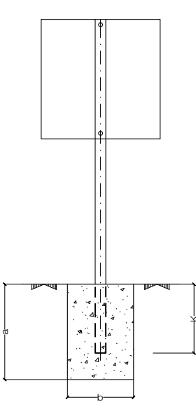
SEÑAL CUADRANGULAR
