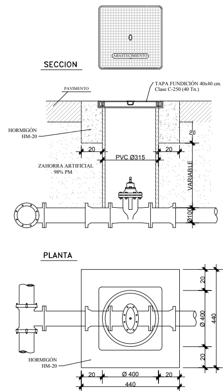
ARQUETA DE TUBO DE PVC PARA VÁLVULA DE SECCIONAMIENTO= < Ø 150 mm S/E
