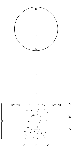
SEÑAL CIRCULAR
