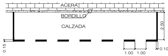
M-7.3 LINEA ESTACIONAMIENTO SIN DELIMITACIÓN DE PLAZAS
