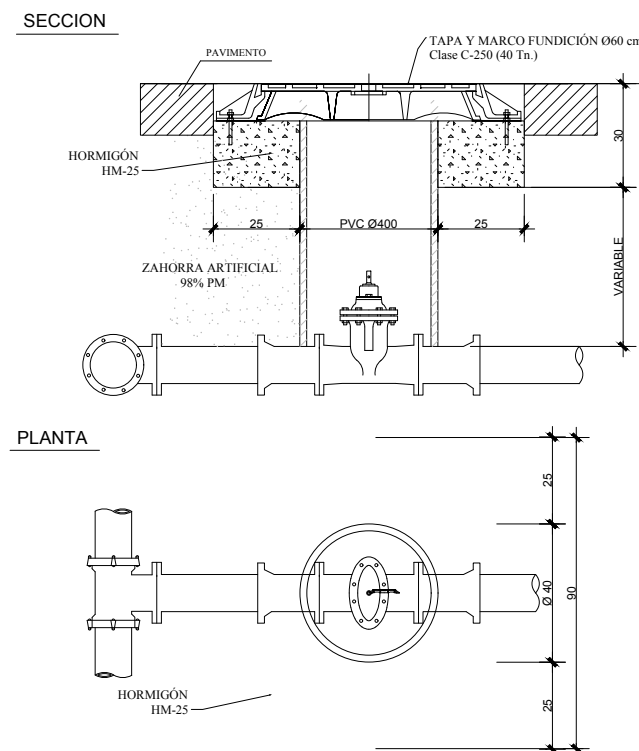
ARQUETA DE TUBO DE PVC PARA VÁLVULA DE SECCIONAMIENTO > Ø 150 mm S/E
