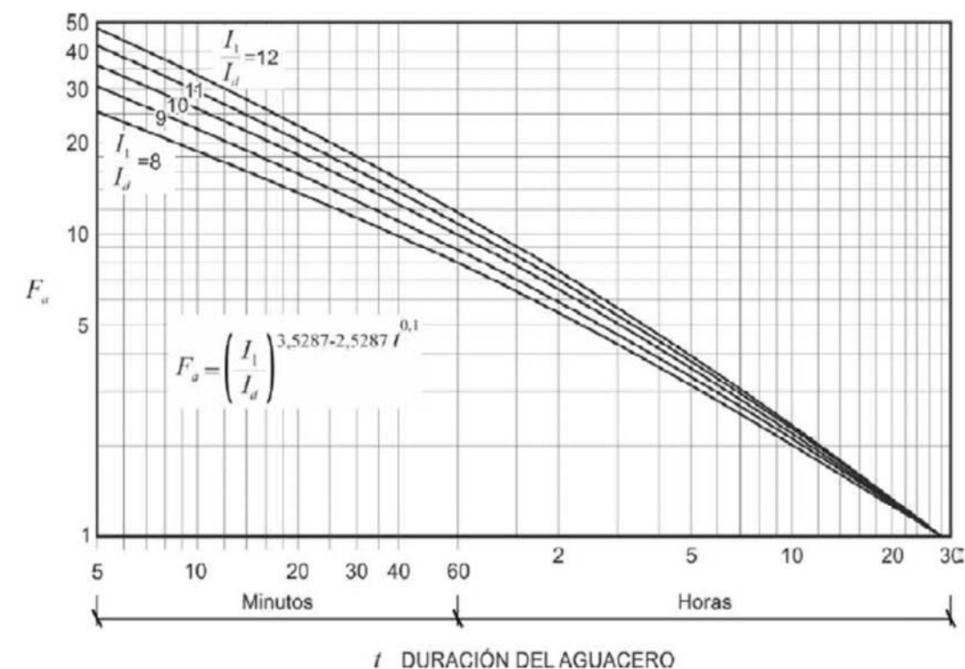
FIGURA 2.3.- FACTOR Fa
