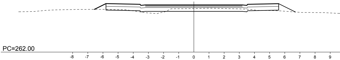
P.K.= 0+240
