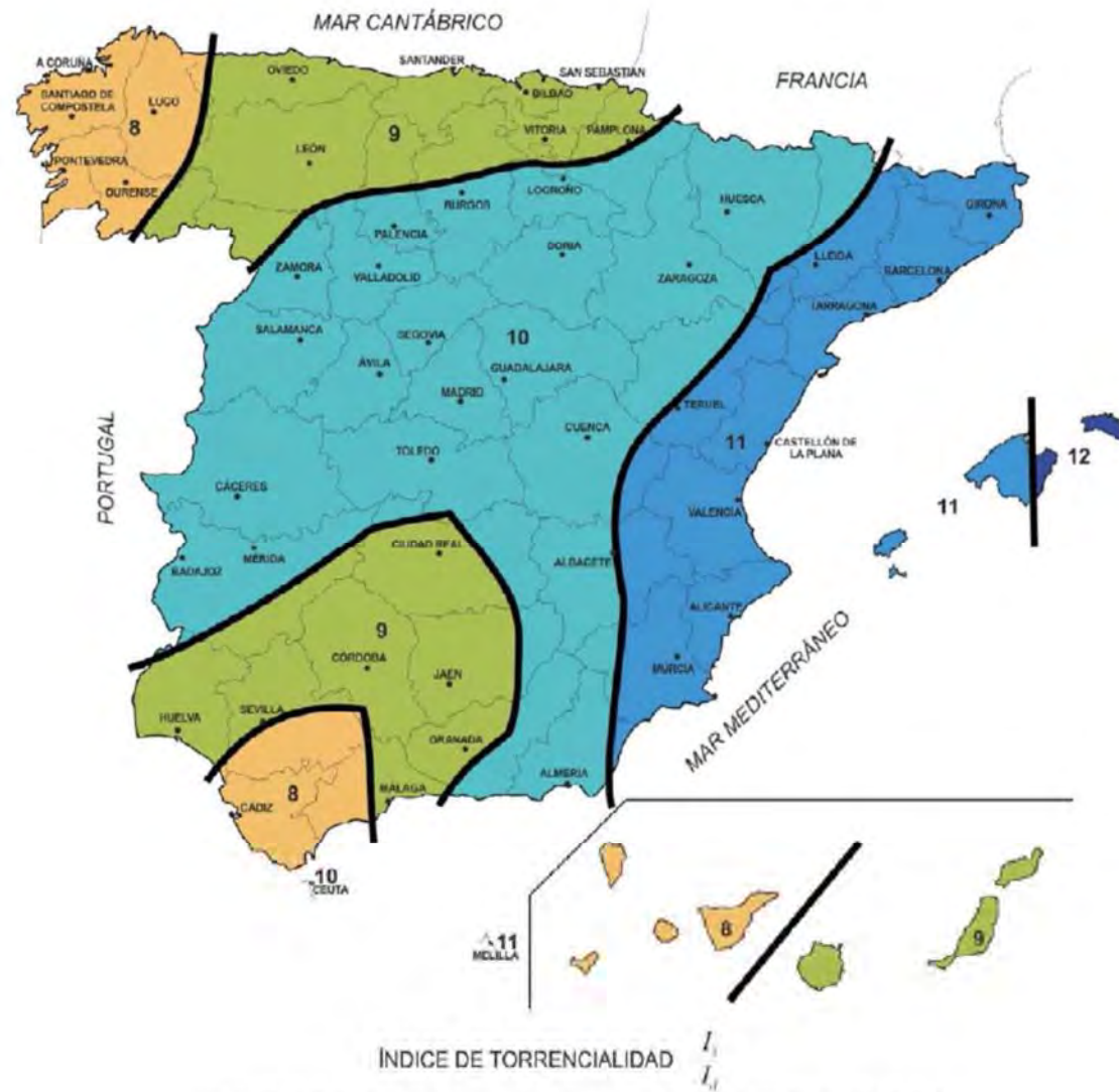
FIGURA 2.4.- MAPA DEL ÍNDICE DE TORRENCIALIDAD ( I_i/I_a )
