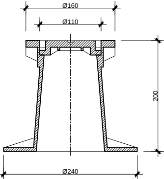
DETALLE ARQUETA
