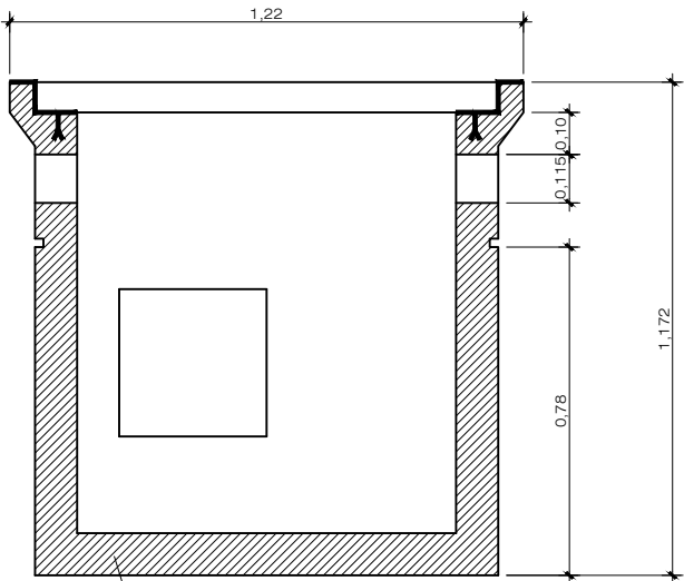
Alzado Seccion B-B
