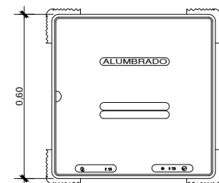
Tapa de registro Fundición ductil 12.5 o 40 tm.
