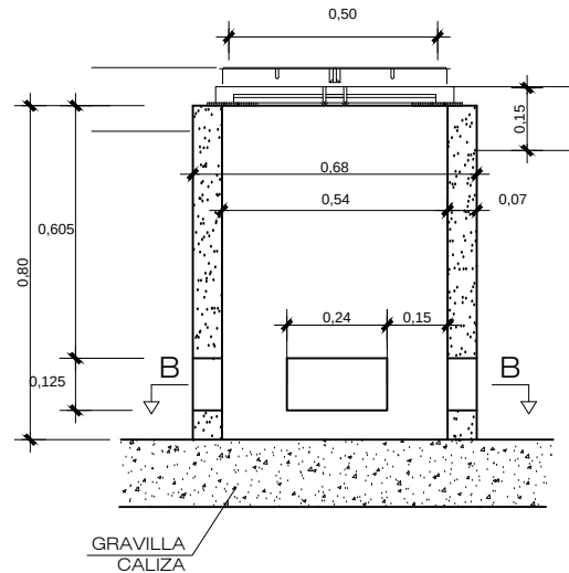
Alzado Sección A-A
