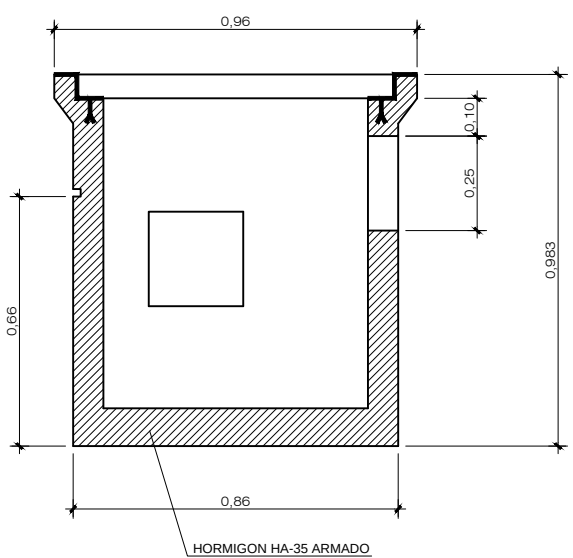
Seccion D-D
