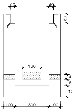
Sección B-B
