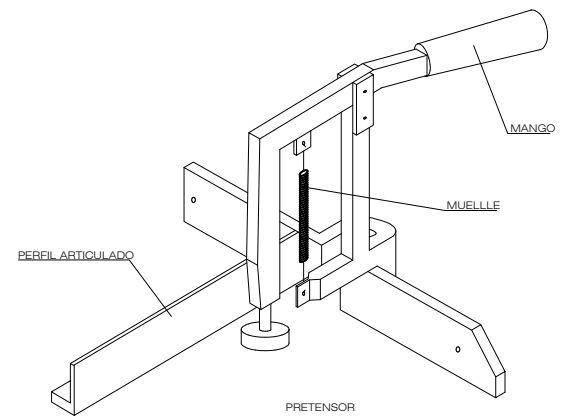
DISPOSITIVO FABRICACION DE CUÑAS
