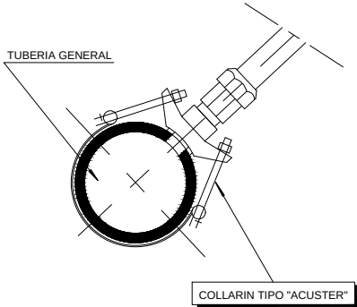
DETALLE DE CONEXION CON GENERAL
