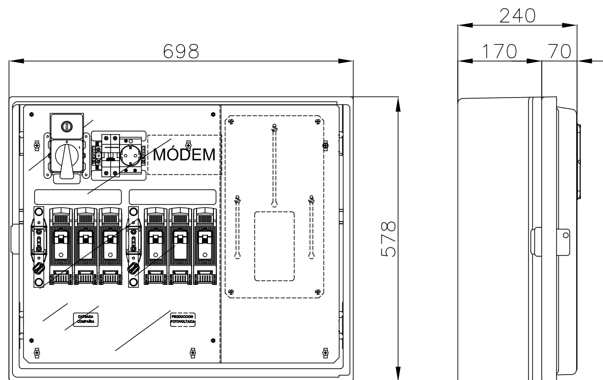
CAJA GENERAL DE PROTECCIÓN Y MEDIDA IF 1TE/C EMPOTRADA
