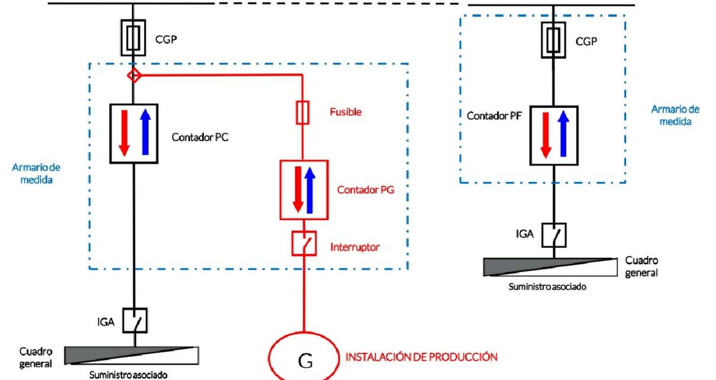
ESQUEMA DE CONEXIÓN AUTOCONSUMO COLECTIVO CON EXCEDENTES A COMPENSACIÓN (GENERACIÓN EN RED INTERIOR) PC+PG EN PARALELO RED BT i-DE-distribución
