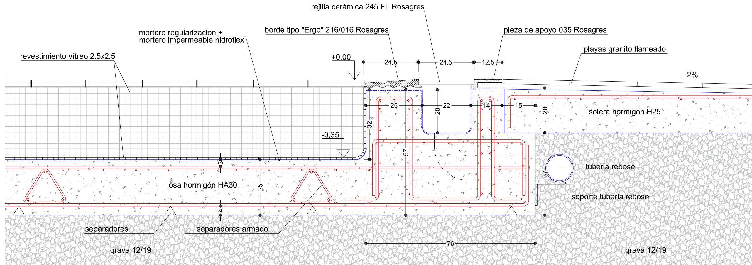
SECCION A-A'
