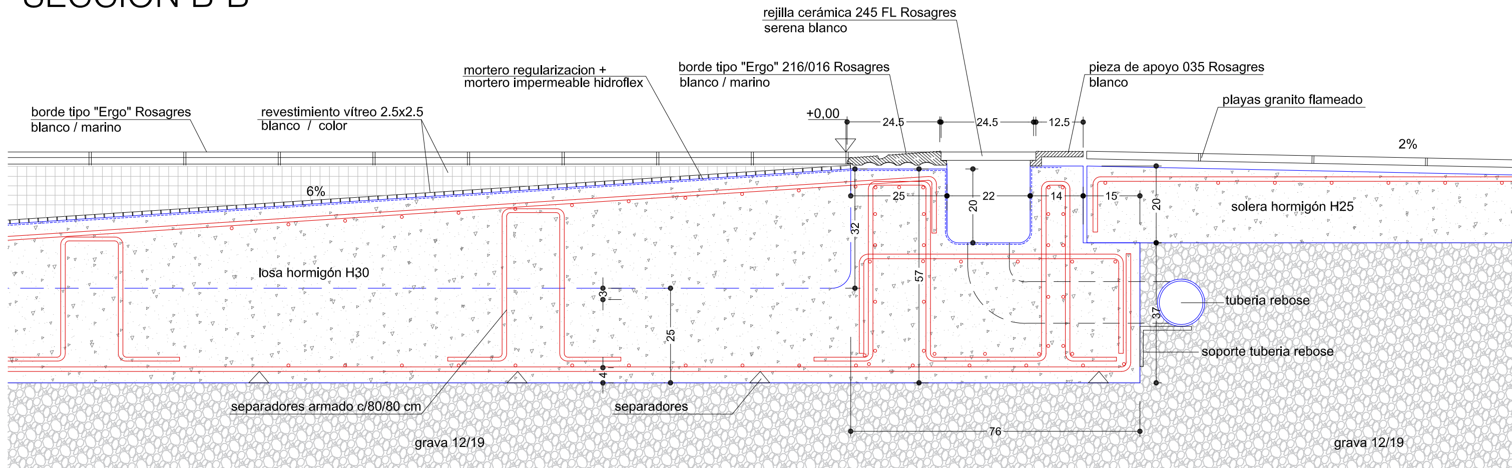
SECCION B-B'
