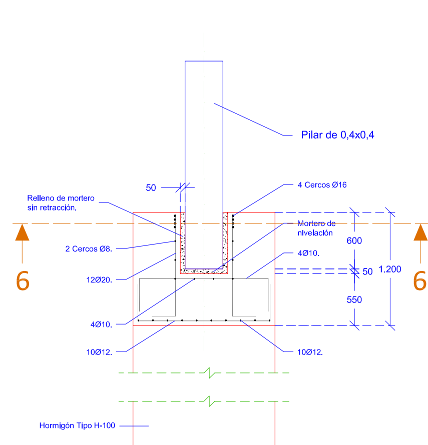
ALZADO SECCIÓN 5-5
