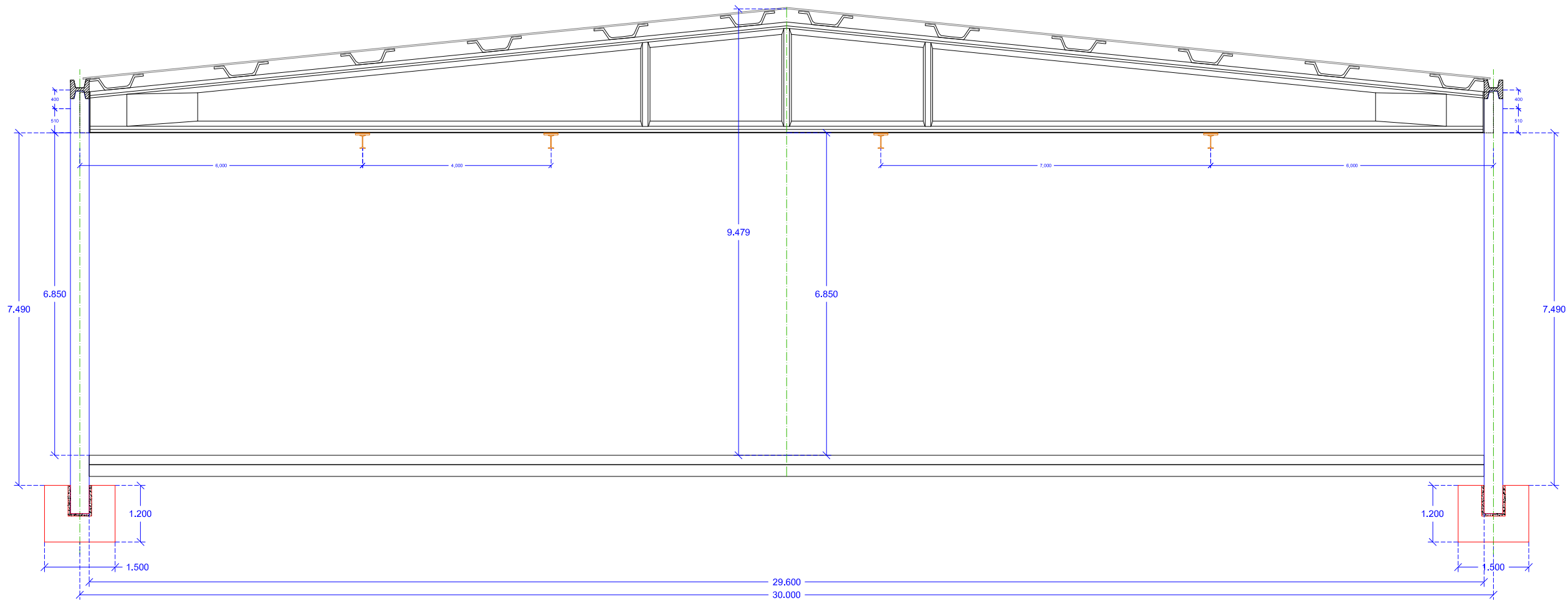
PÓRTICOS 2-3-4-5 y 6
