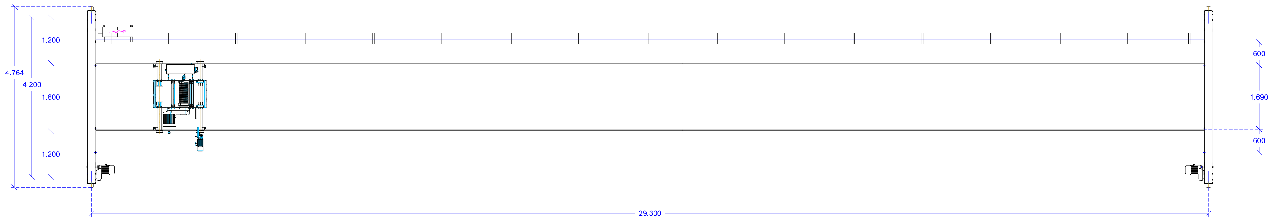
PLANTA DEL PUENTE GRÚA
