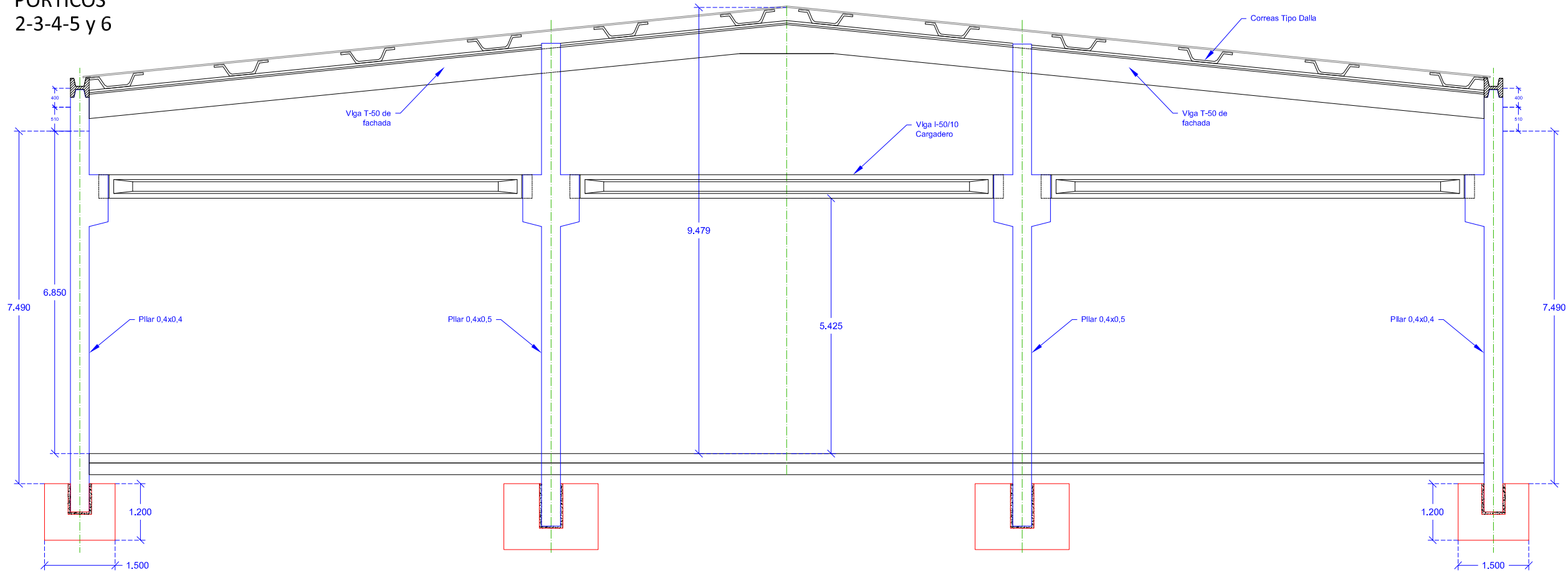
PÓRTICO 7
