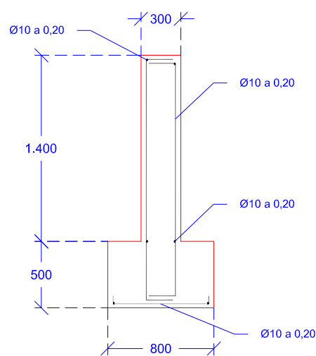
ARMADURA MURO PERIMETRAL
