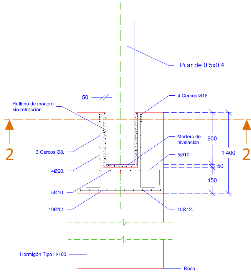
ALZADO SECCIÓN 1-1
