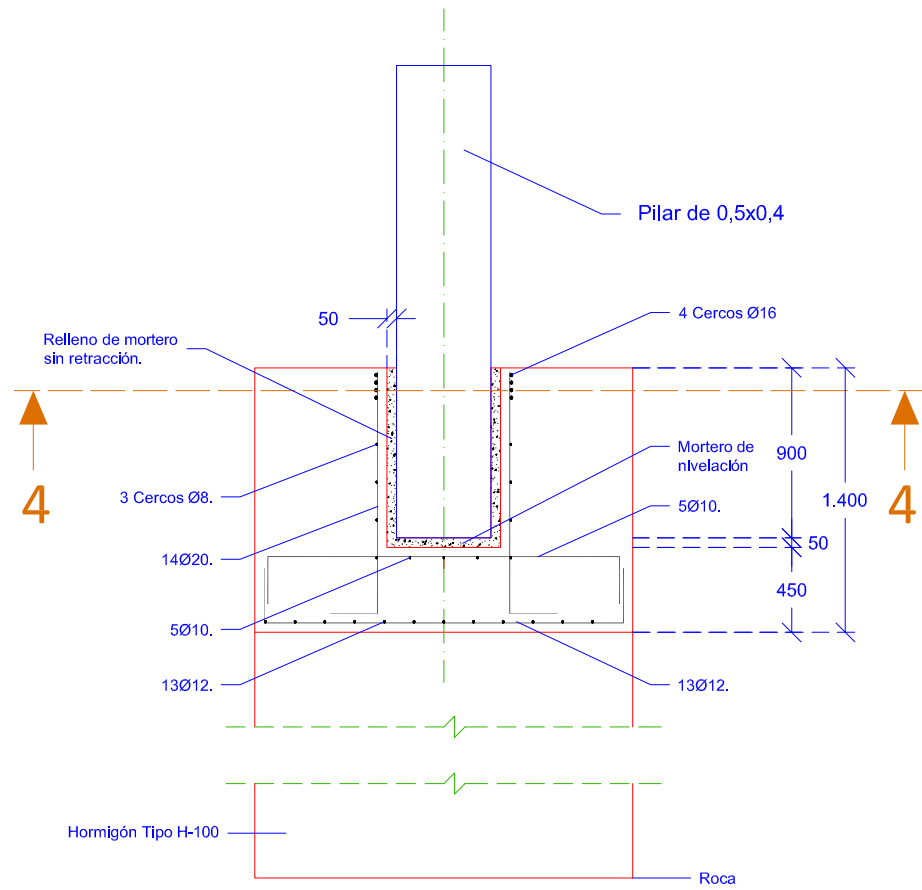
ALZADO SECCIÓN 3-3
