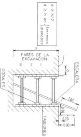
ENTIBACION LIGERA
