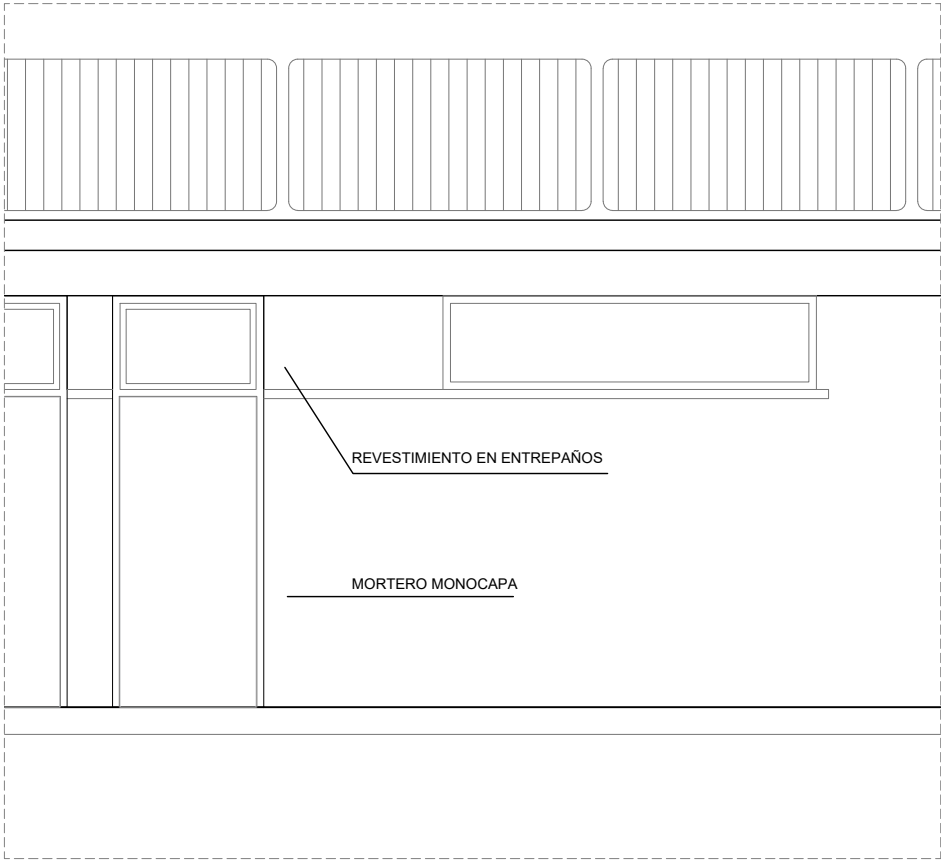
DETALLE ALZADO ACCESO A VESTUARIO_ Esc. 1/50
