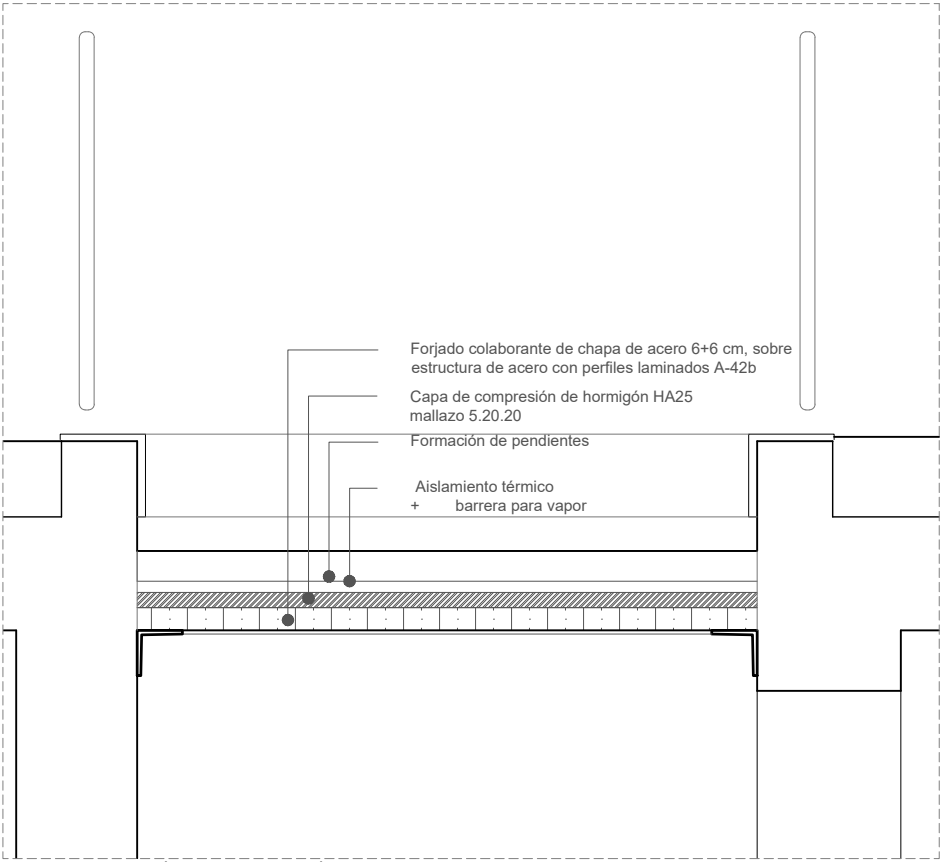
DETALLE MODIFICACIÓN CUBIERTA ALMACÉN GENERAL_ Esc. 1/20
