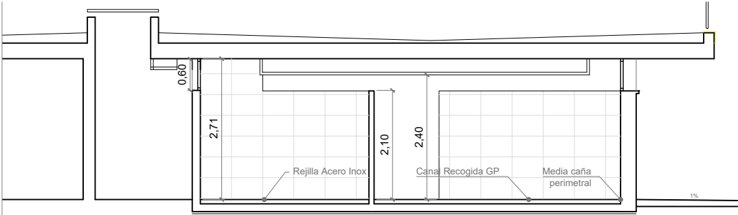
SECCIÓN TRANSVERSAL 3 - VESTUARIOS
