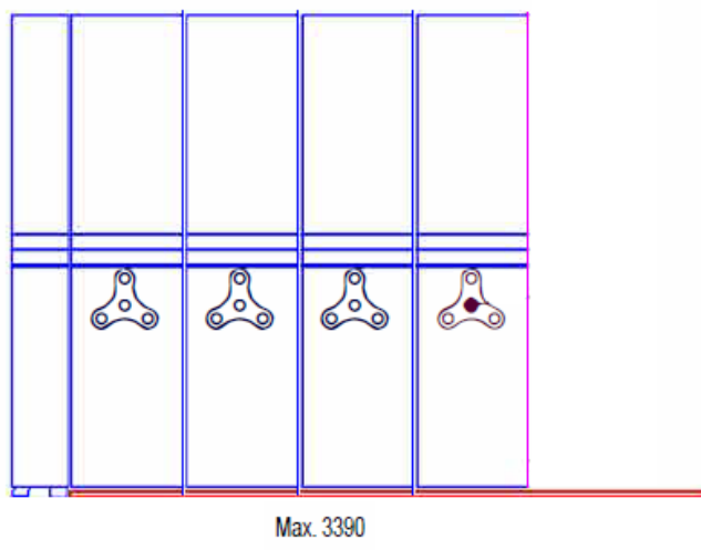
Gráfico 6: Medidas de la envolvente de la planta (sin escala), con estanterías dibujadas y donde el extremo izquierdo es más corto que el resto.
