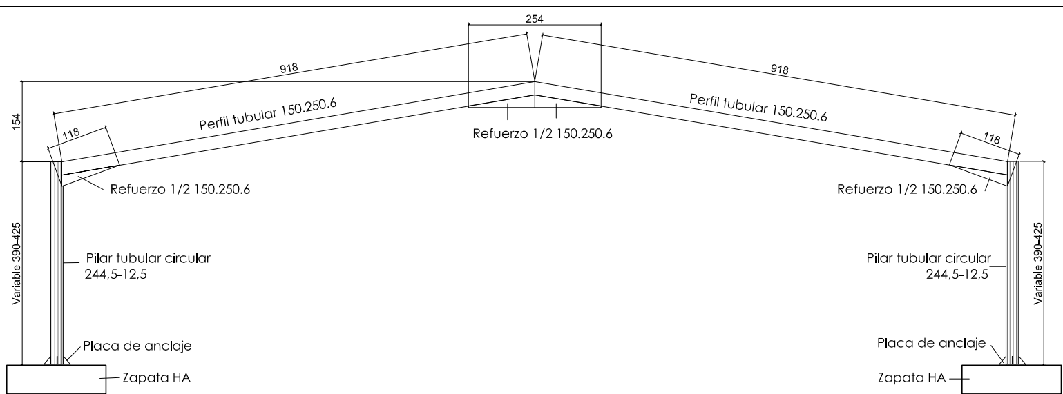
ALZADO PÓRTICO DIAGONAL. V.M. 1/100
