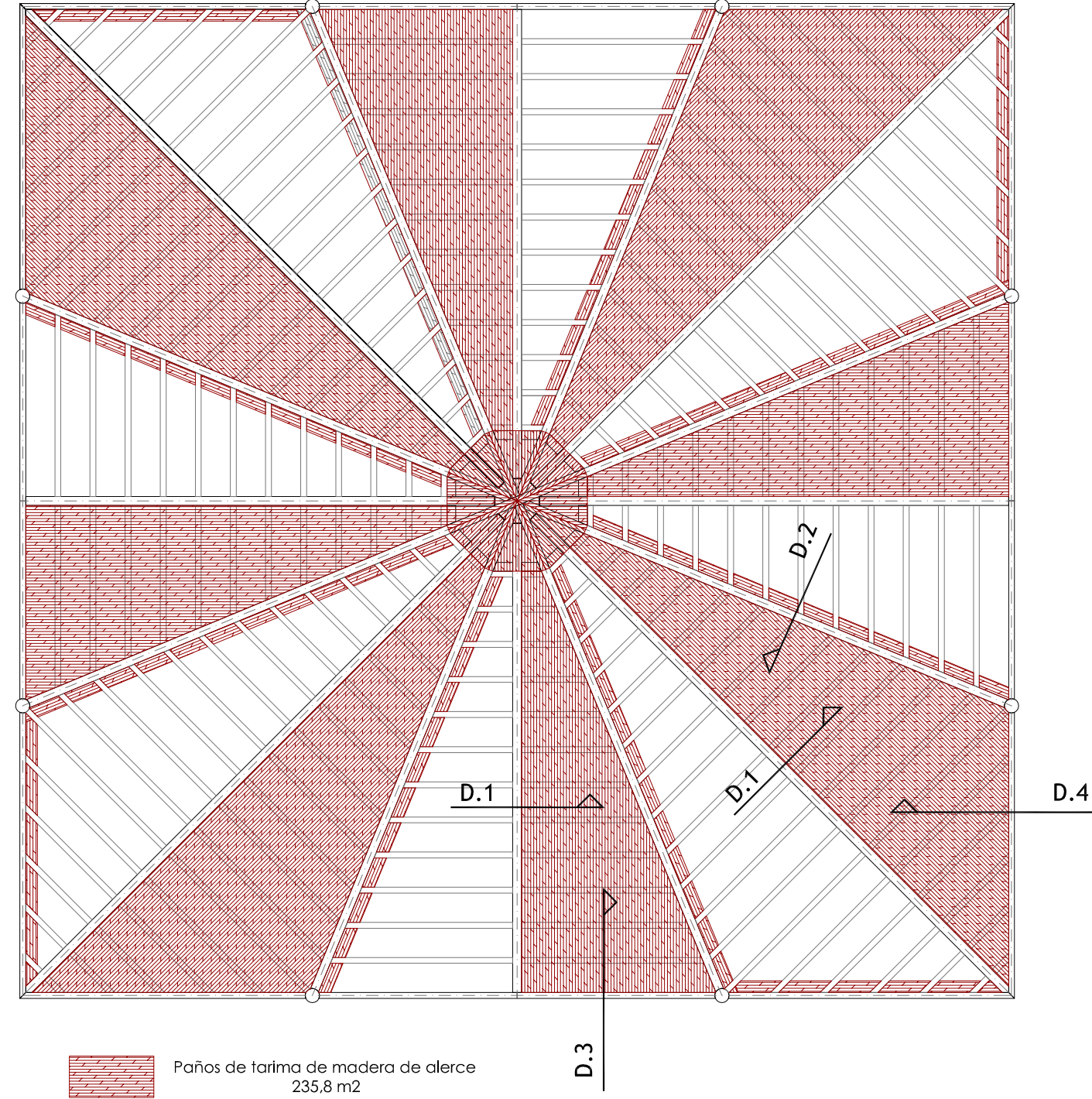
PLANTA PAÑOS DE TARIMA DE MADERA 1/100
