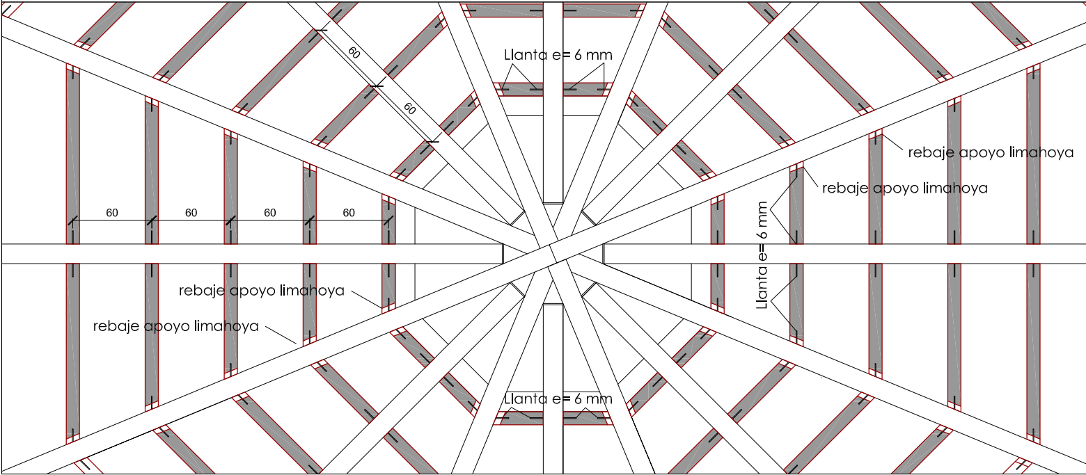
PLANTA DETALLE UNIÓN CABIOS-VIGAS DE MADERA 1/40
