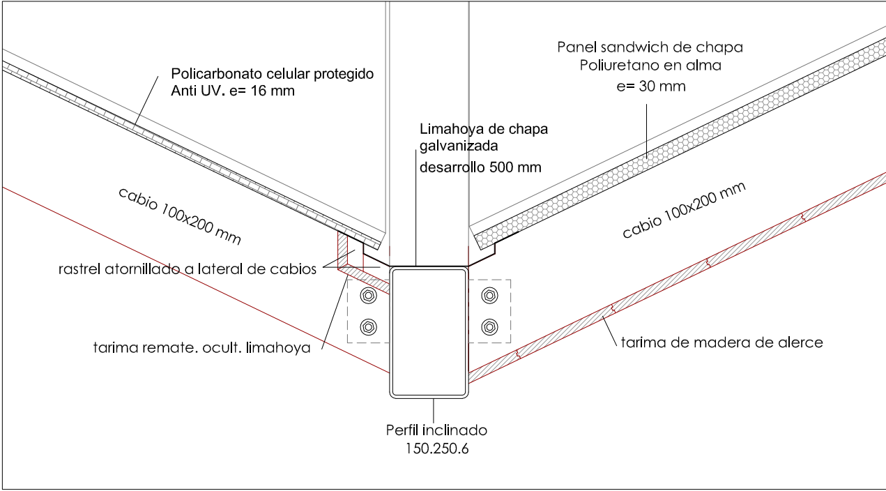
DETALLE D.2. SECCIÓN LIMAHoya 1/10
