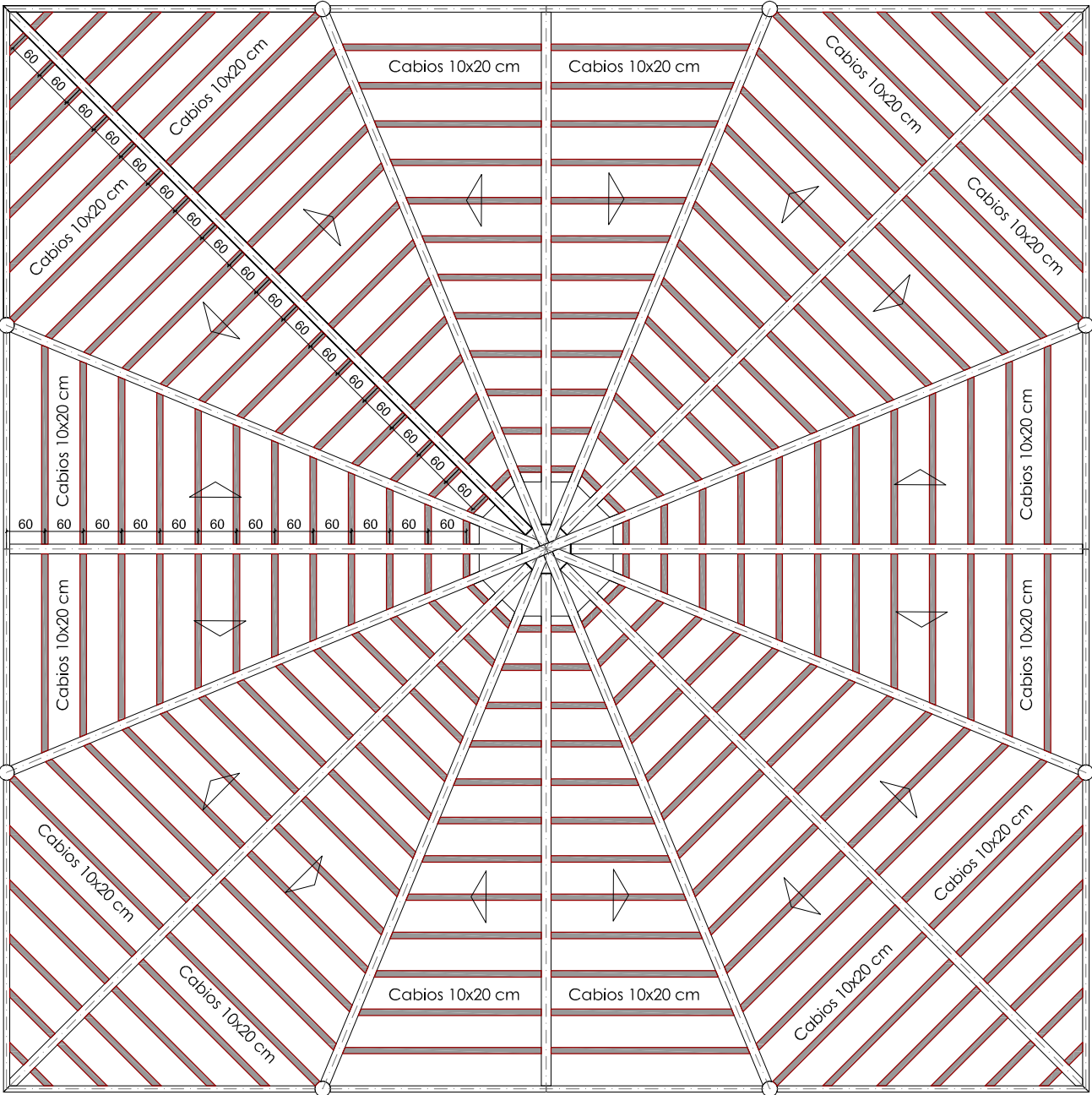
PLANTA DETALLE UNIÓN CABIOS-VIGAS DE MADERA 1/40
