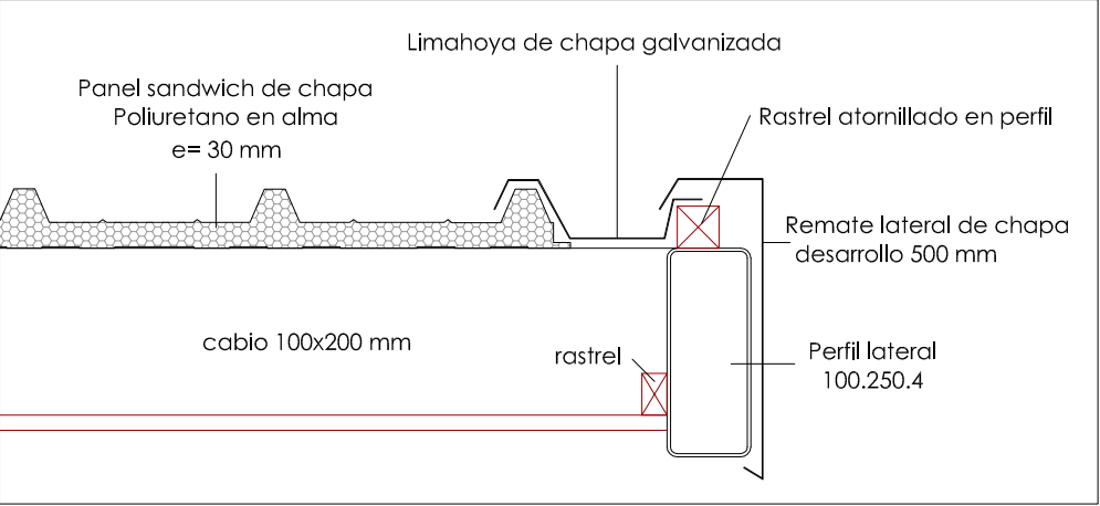
DETALLE D.4. SECCIÓN REMATE LATERAL OBLICUO 1/10
