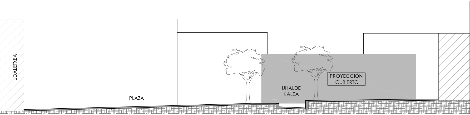
SECCIÓN B-B
