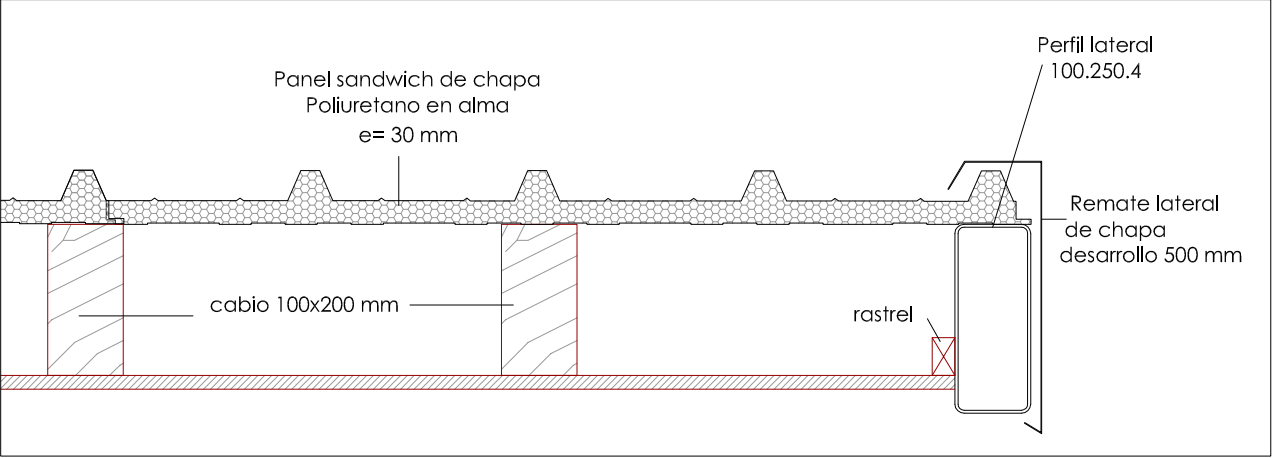
DETALLE D.3. SECCIÓN REMATE LATERAL RECTO 1/10
