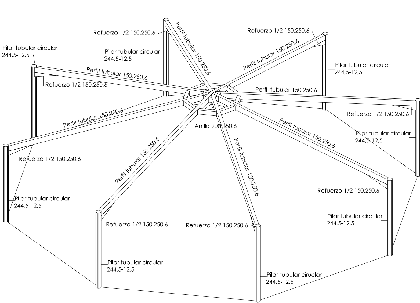
AXONOMÉTRICO ESTRUCTURA PRINCIPAL 1/100
