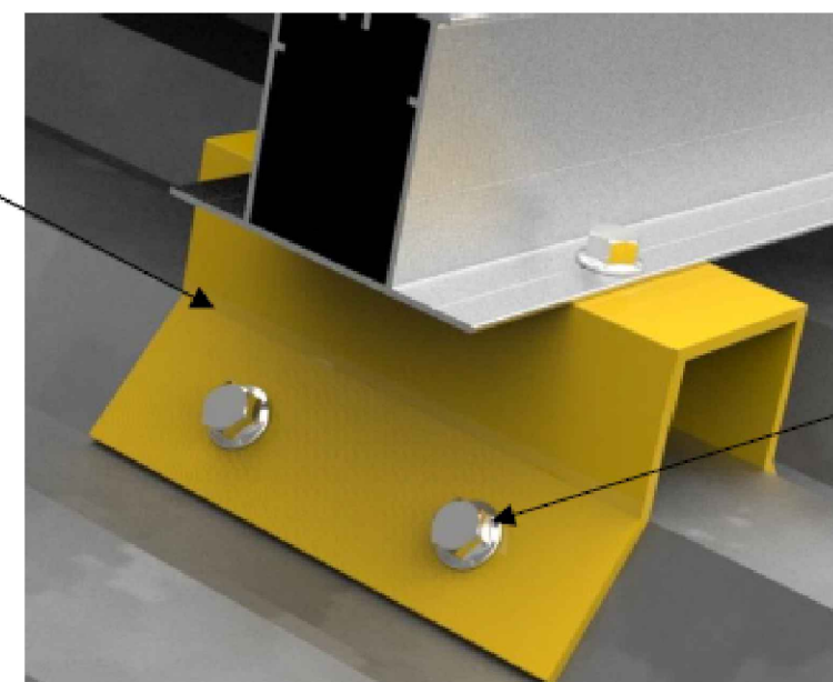
Autotaladrantes zincados DIN 7504-KORe 6,3x25
