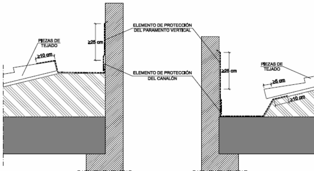
Figura 2.17 Canalones
