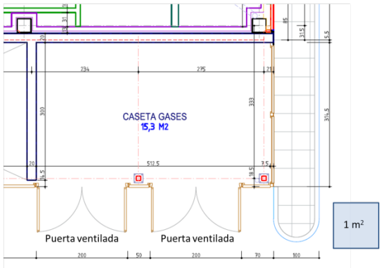
Caseta de gases proyecto obra civil: Planta
