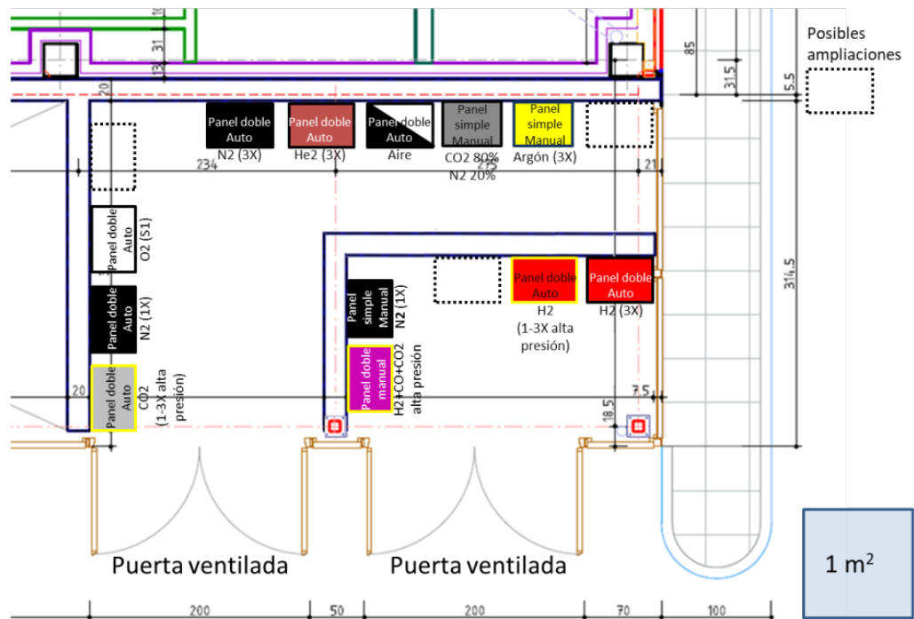
Caseta de gases: Organización propuesta
