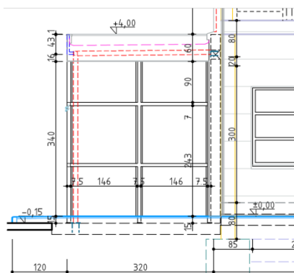
Caseta de gases proyecto obra civil: Perfil
