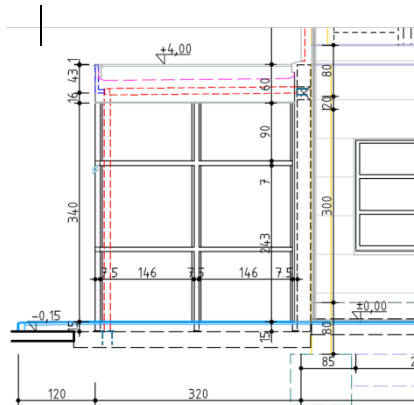
Caseta de gases proyecto obra civil: Perfil
