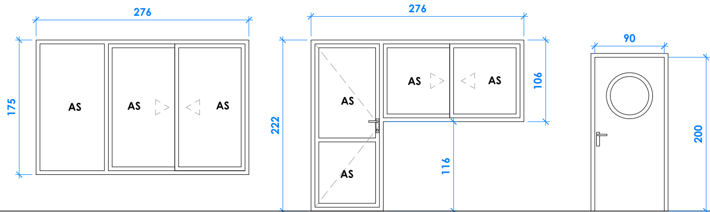
V1 ALUMINIO ANODIZADO PLATA 2 ud.
