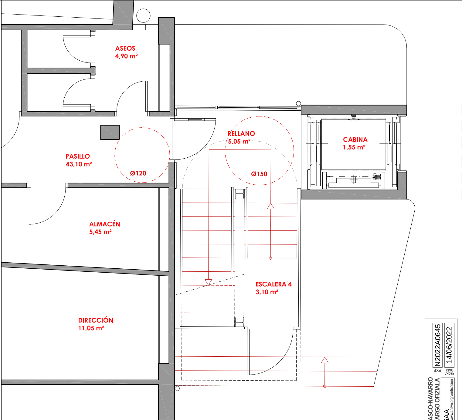
PLANTA BAJA
