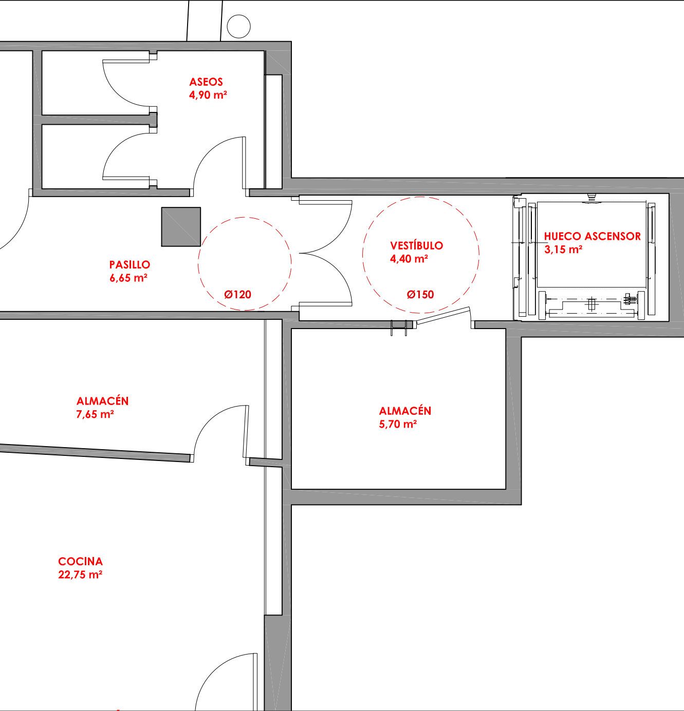
PLANTA SEMISÓTANO
