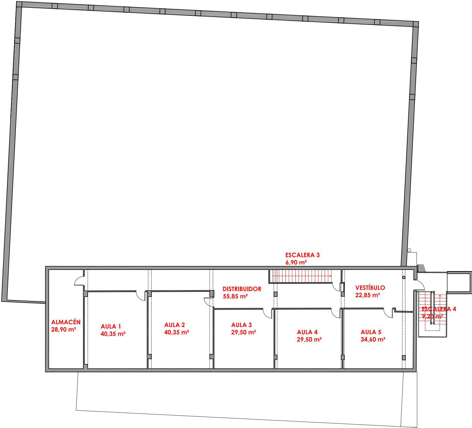
PLANTA TERCERA
