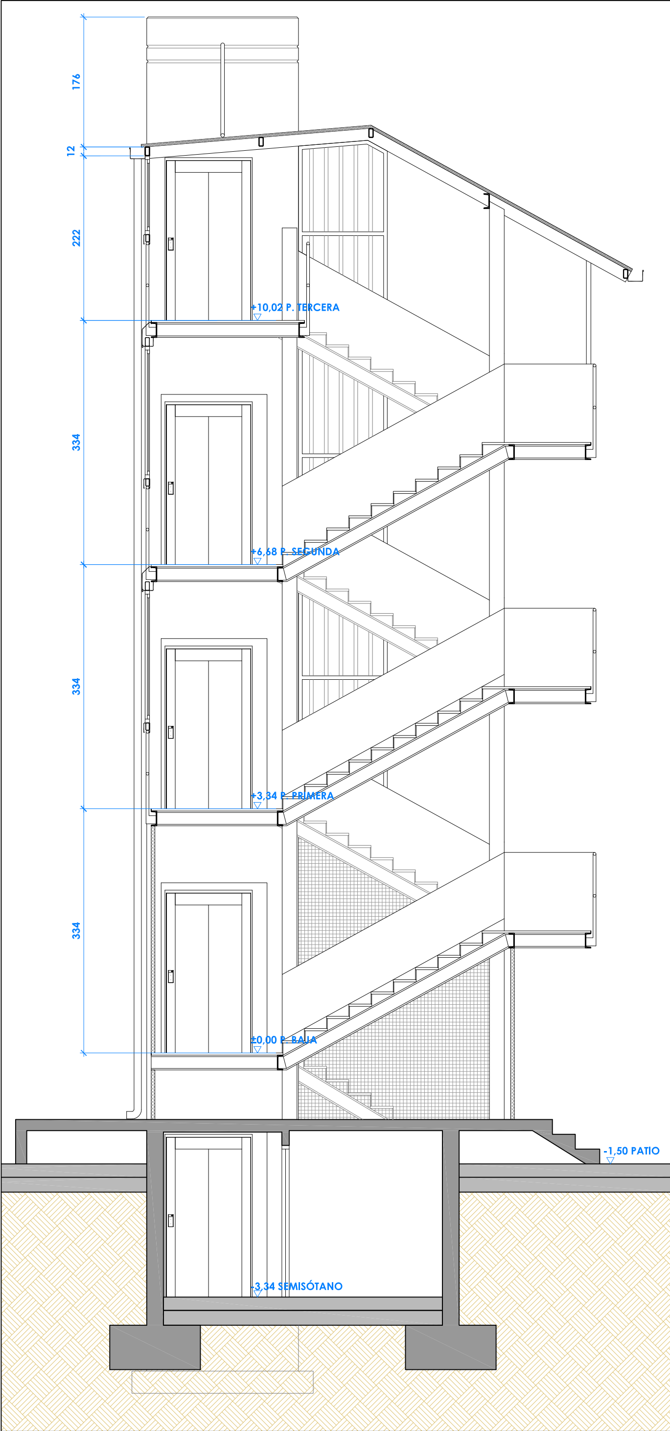
SECCIÓN B-B'
