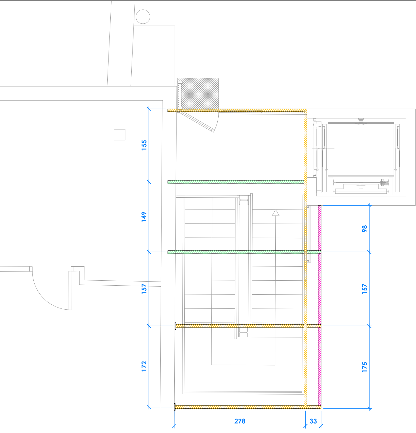
PLANTA TERCERA
