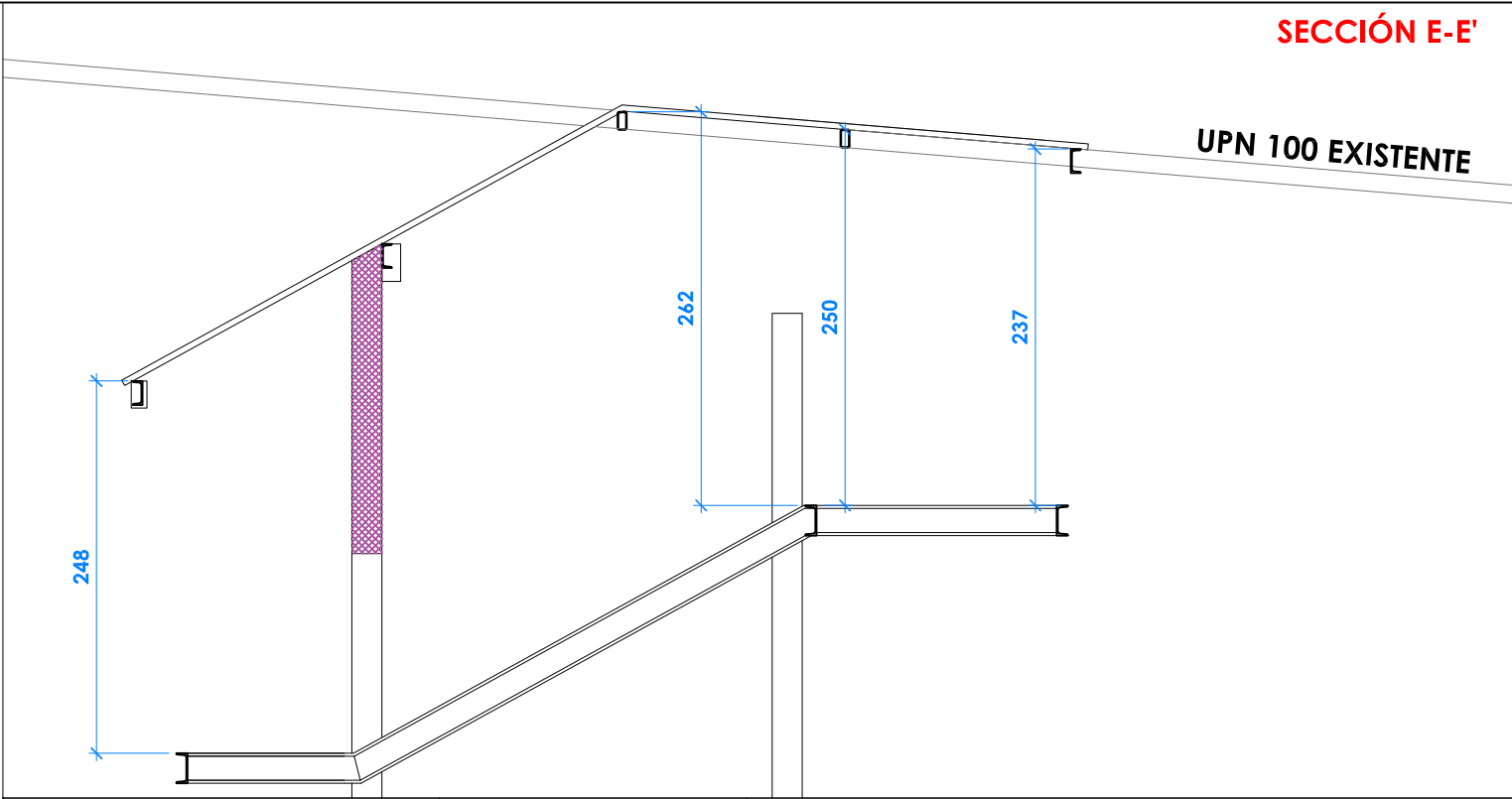
SECCIÓN E-E'
