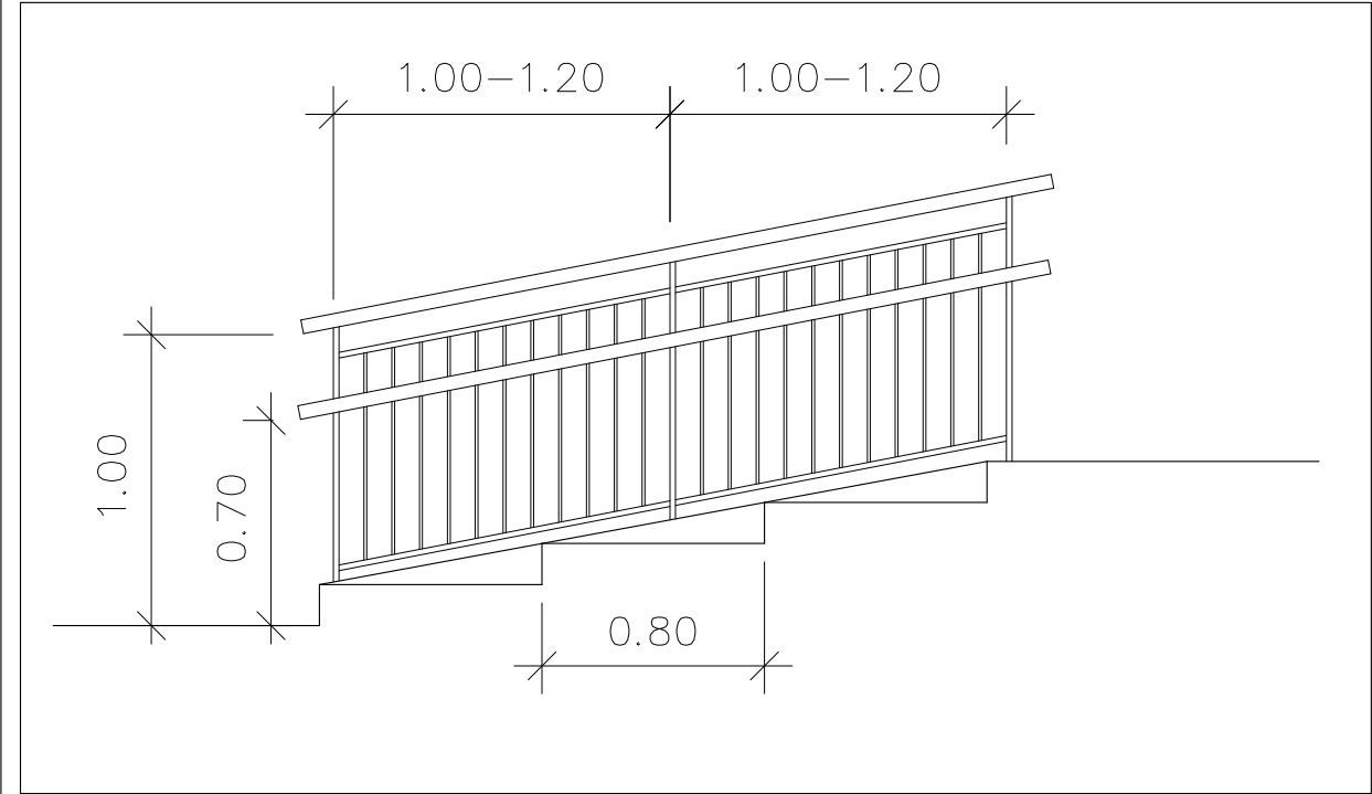
DETALLE BARANDILLAS E:1/30
