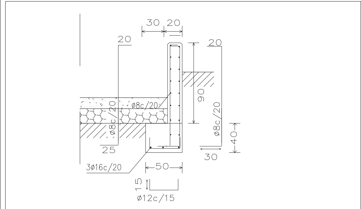
DETALLE MURO SEPARACIÓN RAMPA-ESCALERAS
