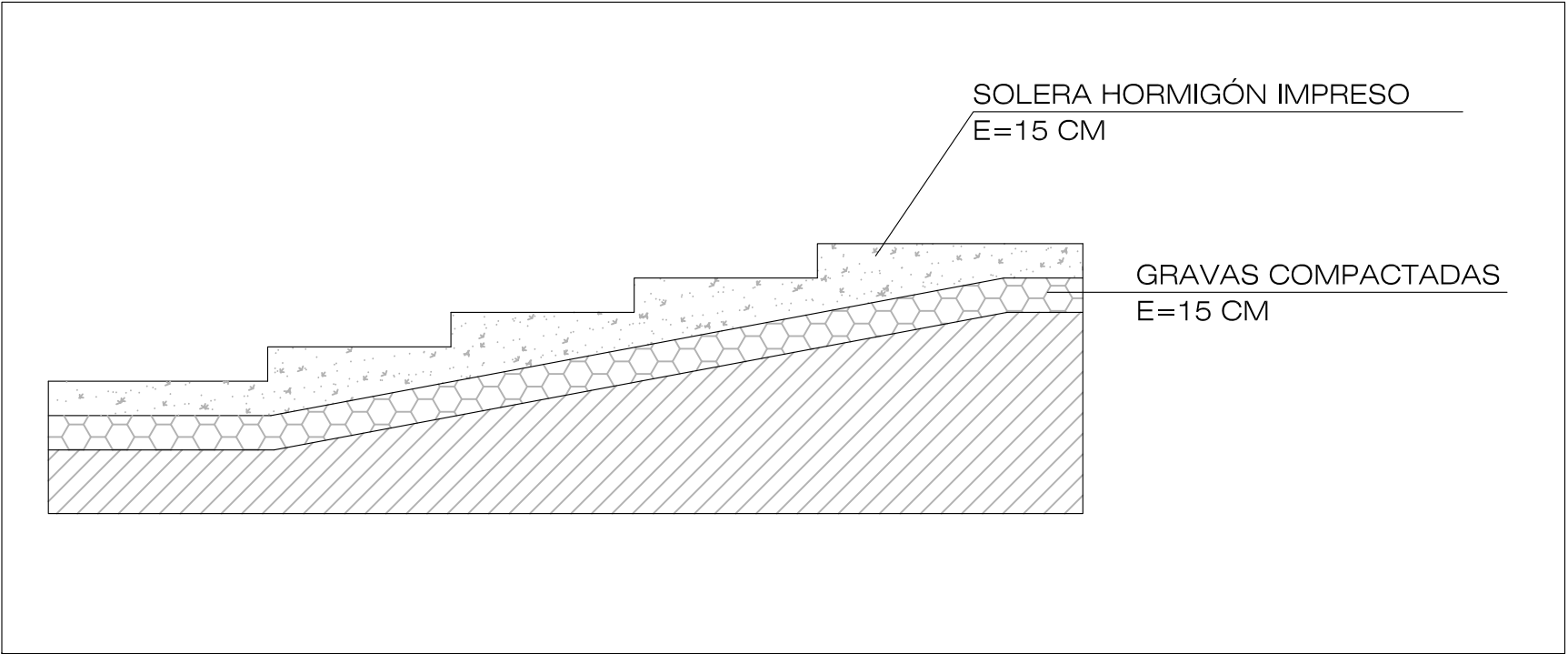
SECCIÓN POR ESCALERAS E:1/30
