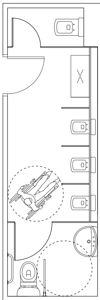
ESTADO REFORMADO
