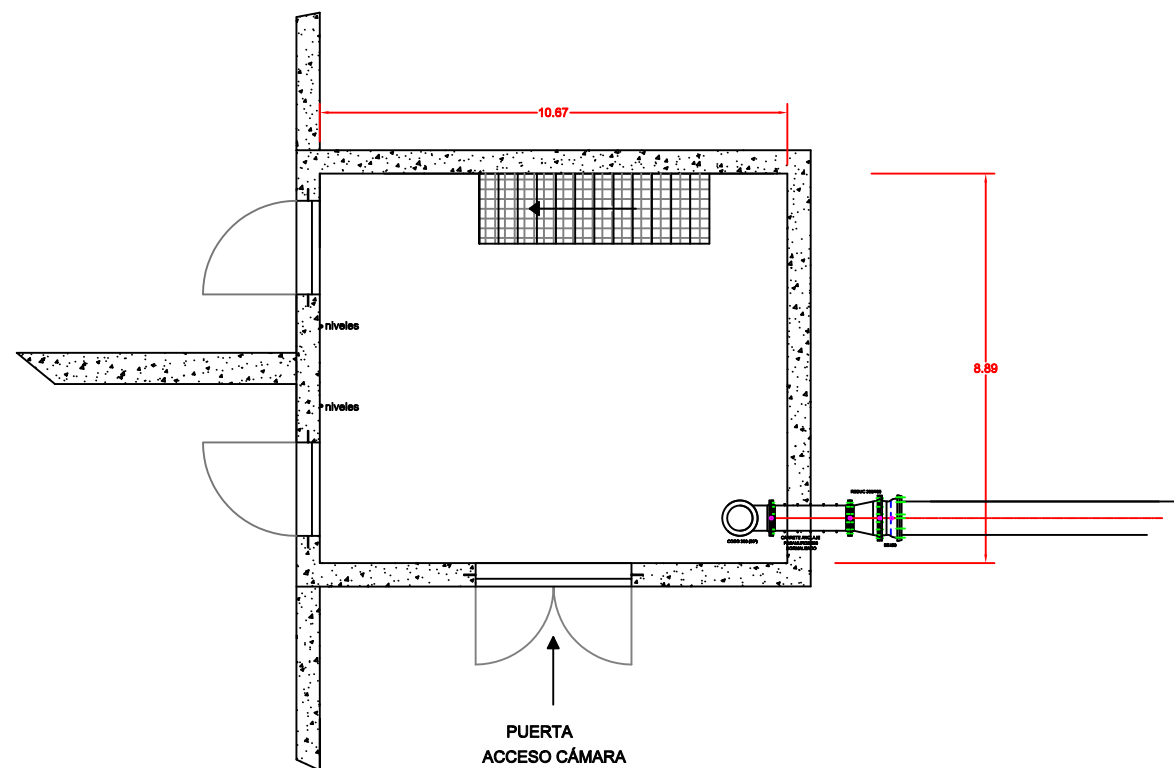
PLANTA BAJA- Almacén, Puertas de acceso vasos
