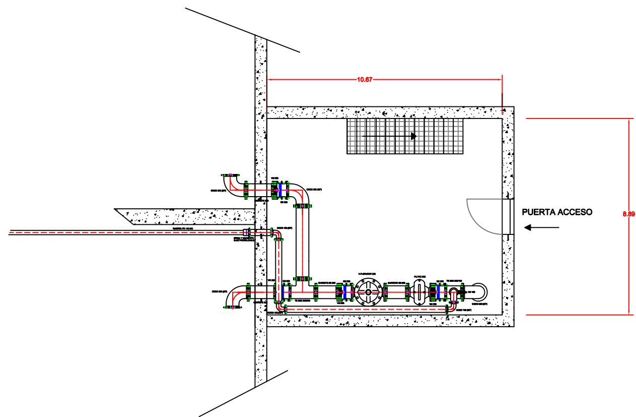
PLANTA 1ª- Válvulas
