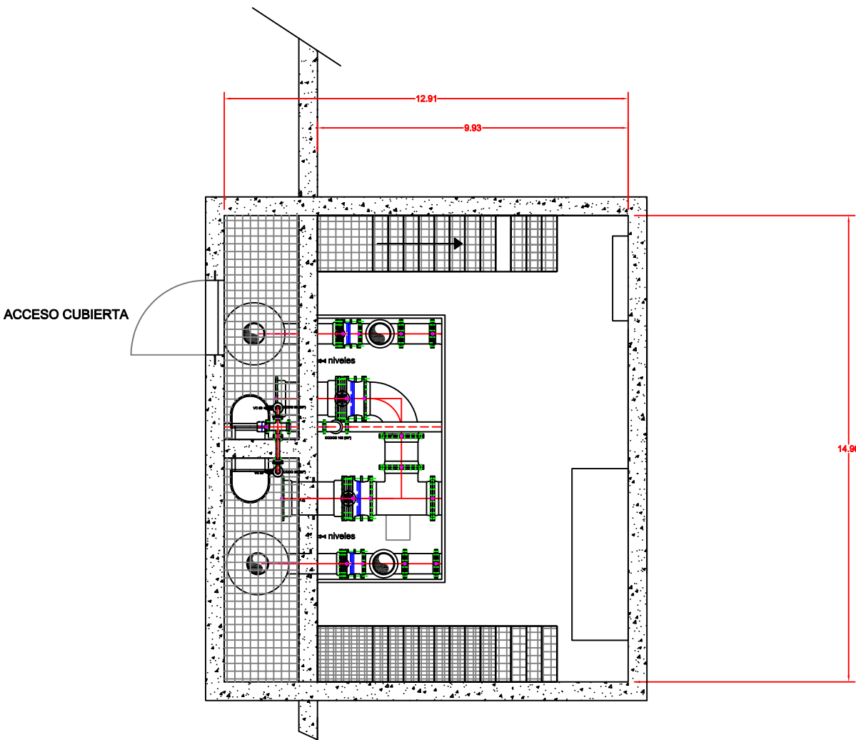
PLANTA 1ª- Accesos cubierta y vasos
