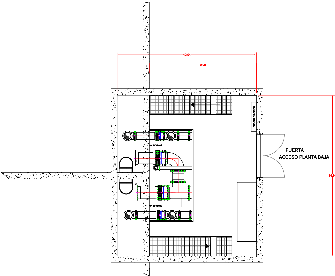
PLANTA BAJA- Almacén, niveles, cuadros electricos y laboratorio
