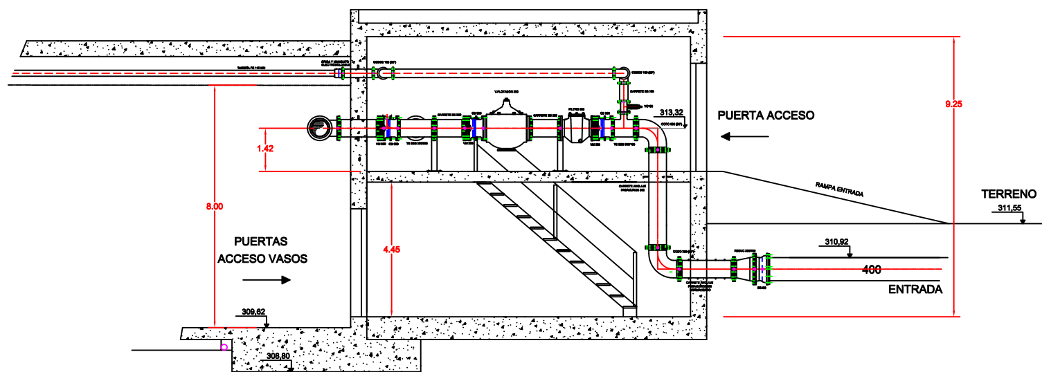
ALZADO
