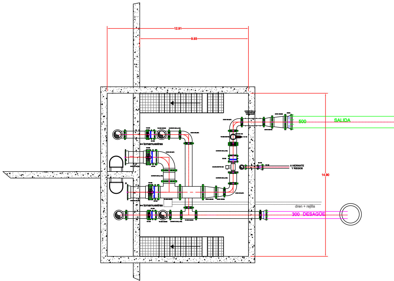
PLANTA SÓTANO- Válvulas y puertas de acceso vasos
