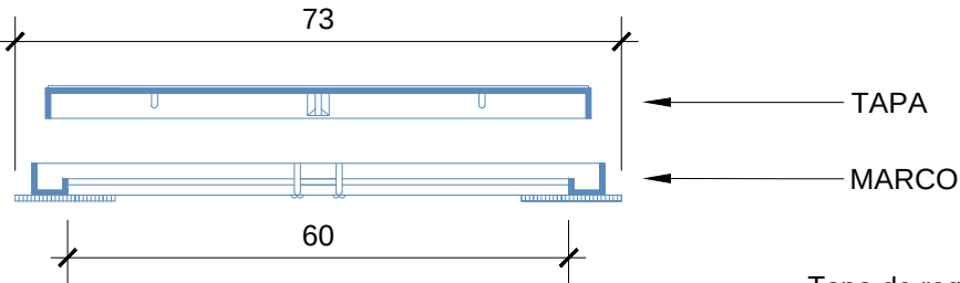
DETALLE DE TAPA Y MARCO
