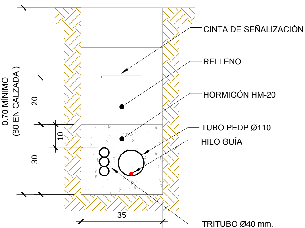
DETALLE DE ZANJA
