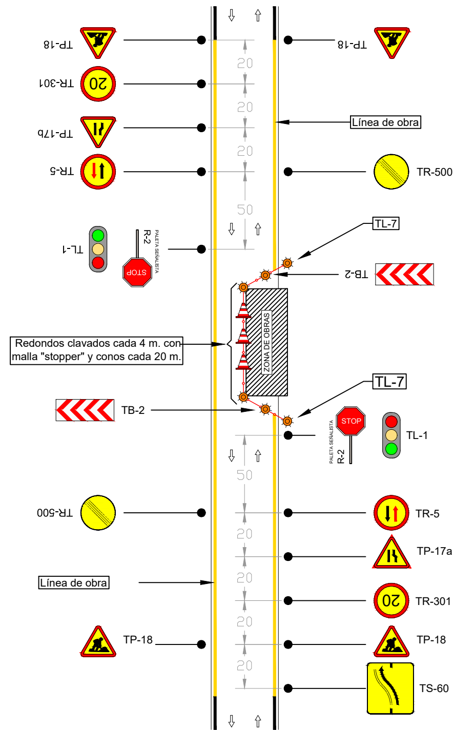
DETALLE DE CRUCE DE CARRETERA PRIVADA CON INTERRUPCIÓN TEMPORAL DE UN CARRIL.
