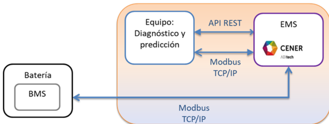
Figura 1. Comunicaciones entre el Software, el EMS y la batería.
