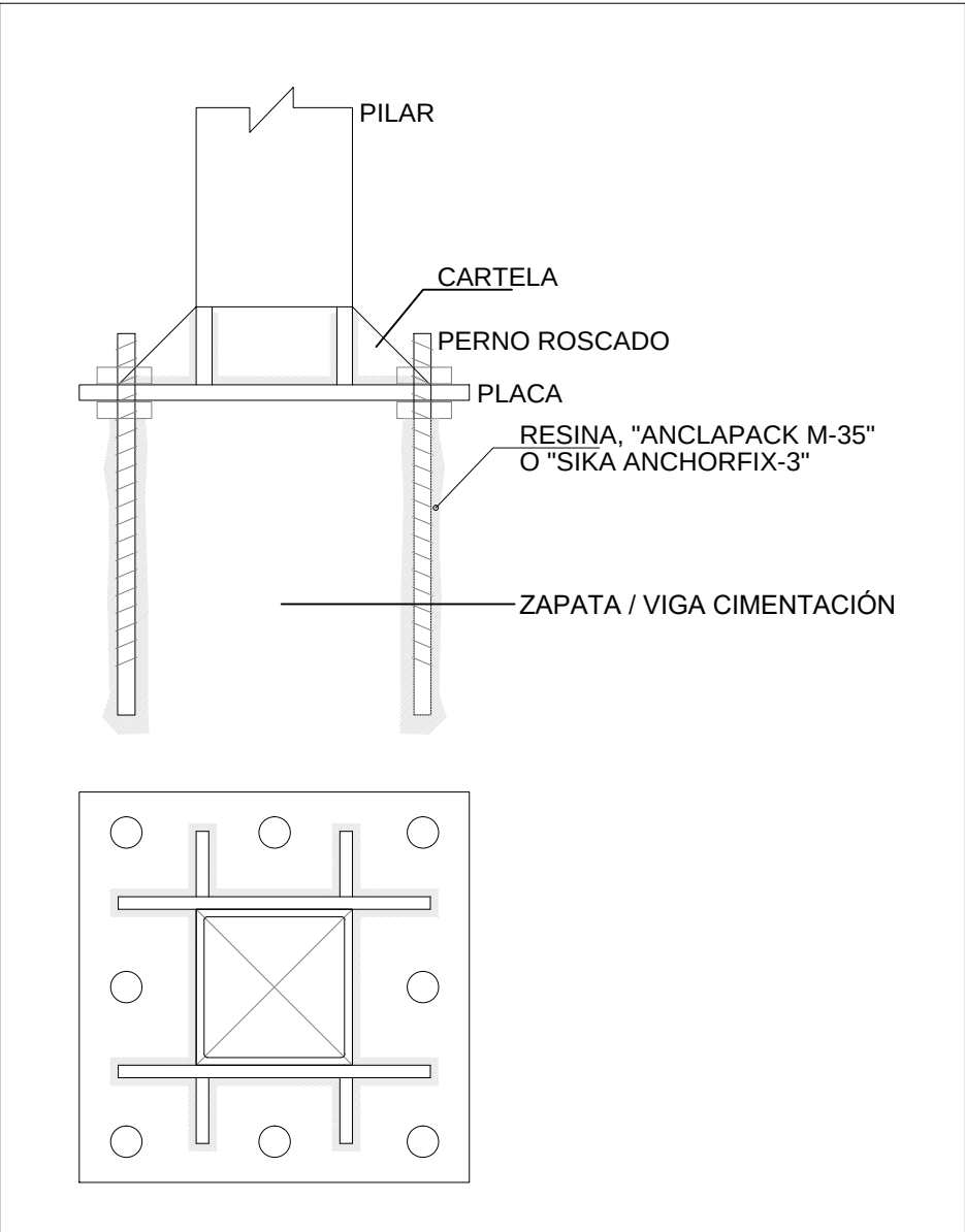
DETALLE PLACA ANCLAJE. E: 1/5
