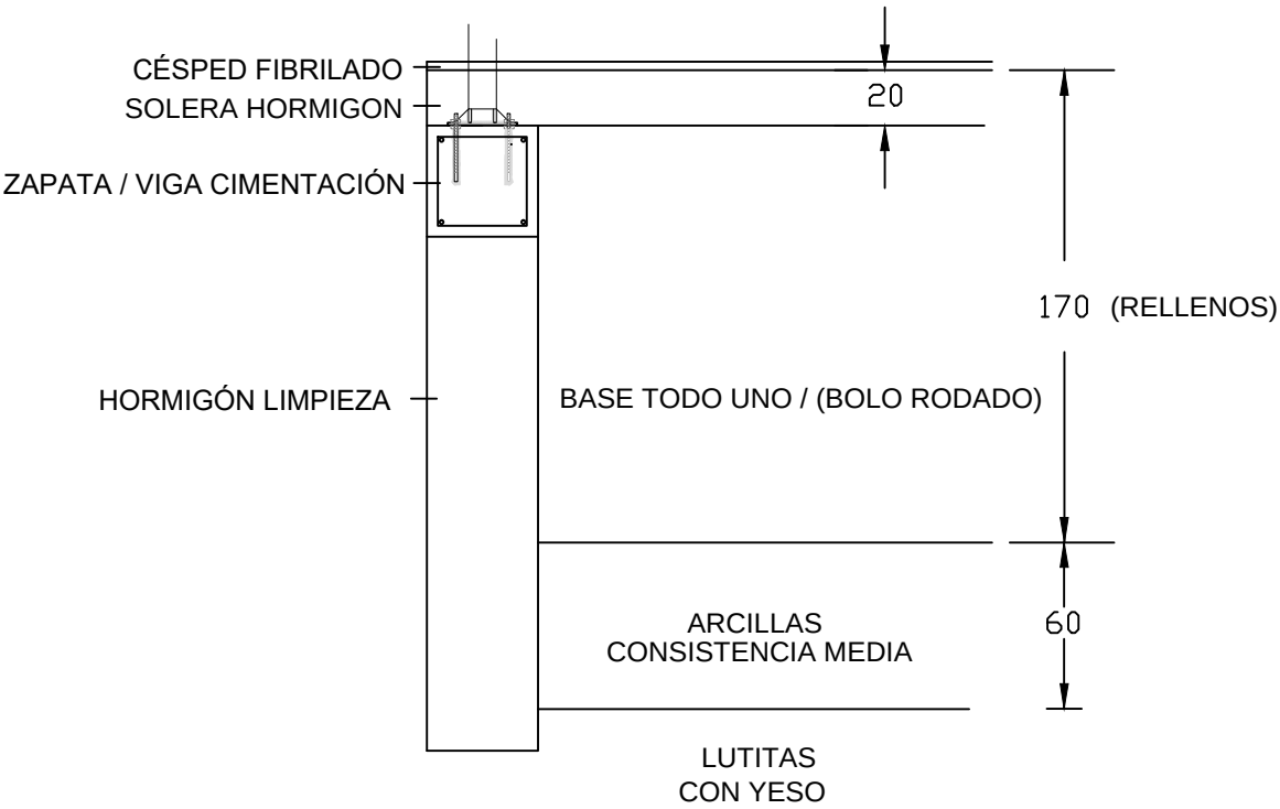
DETALLE CIMENTACIÓN. E: 1/30
