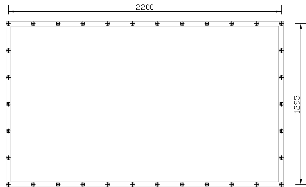
PLANTA GENERAL CIMENTACIÓN. E: 1/150
