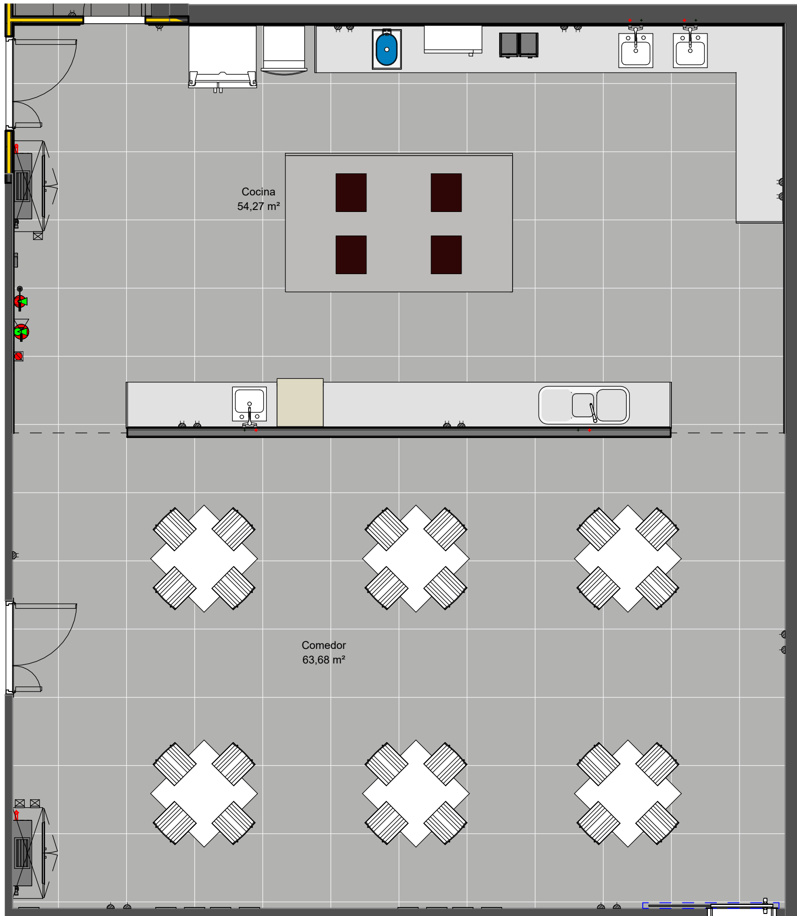
2 OC-DISTRIB COCINA PROP 1 : 50
