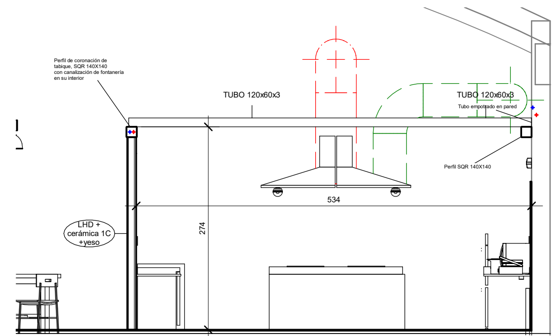
3 OC-SEC-ESTR-CAMPANA 1 : 50
