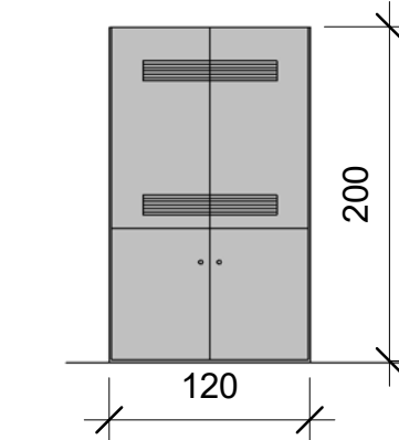
CUBRE COLECTORES-FANCOILS A1
