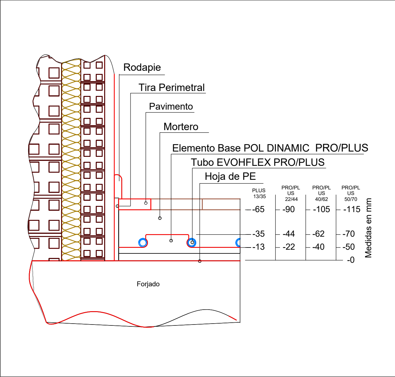
2 C-DET-SUELO 1 : 3
