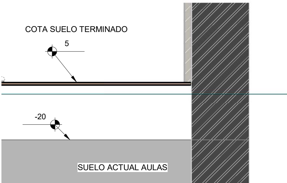
2 OC-SECCION SUELO AULAS 1 : 10
