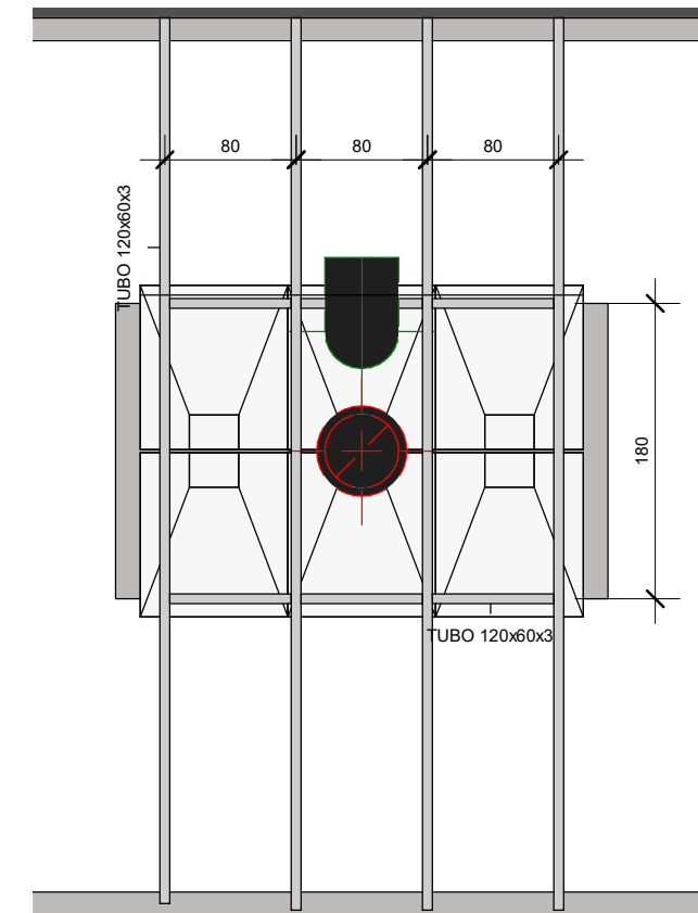
1 OC- ESTRUCTURA CAMPANA 1 : 50
