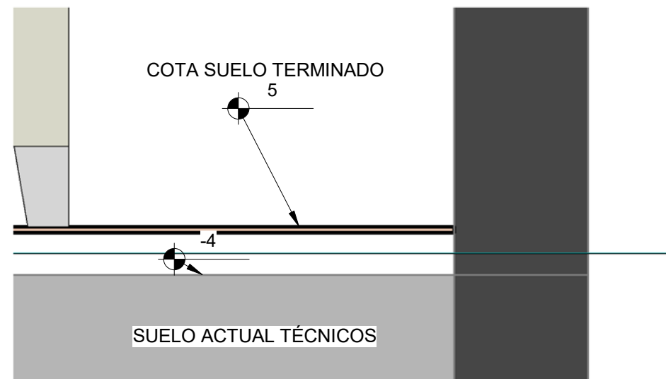
3 OC-SECCION SUELO TECNICOS 1 : 10
