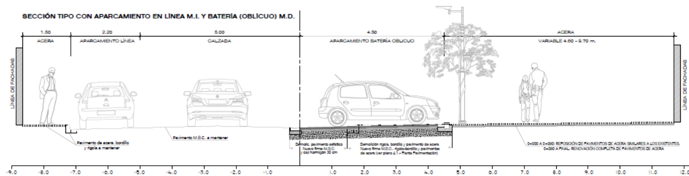
Sección-tipo general propuesta
