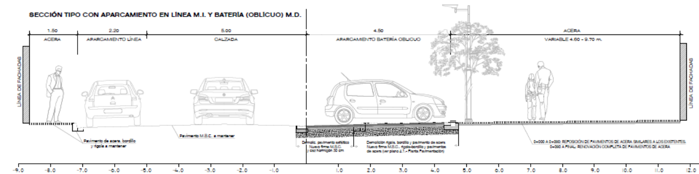
Sección-tipo general propuesta
