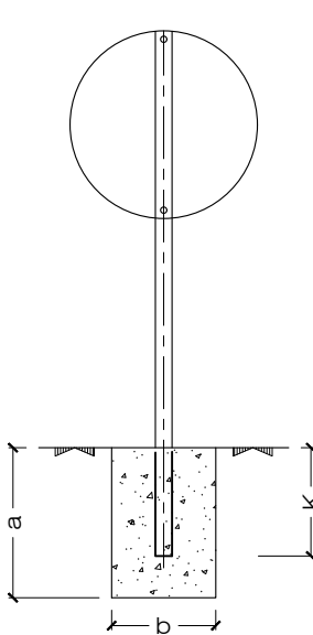
SEÑAL CIRCULAR
