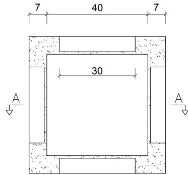
Planta Sección B-B
