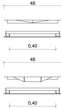
Tapa de registro Fundición ductil 12.5 o 40 tm.
