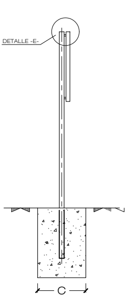
SECCIÓN TIPO
