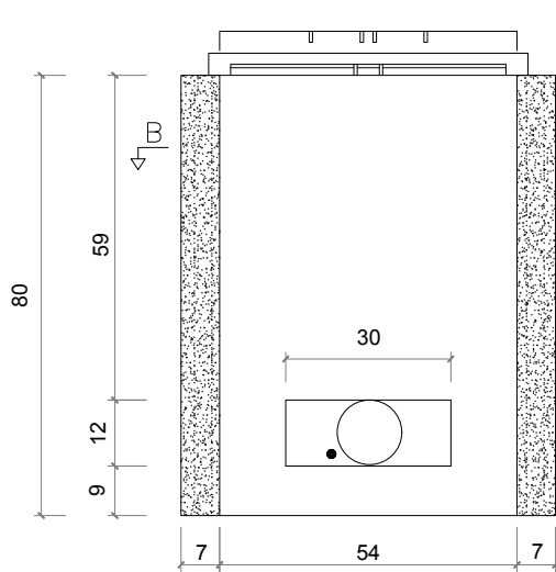
Tapa de registro Fundición ductil 12.5 o 40 tm.
