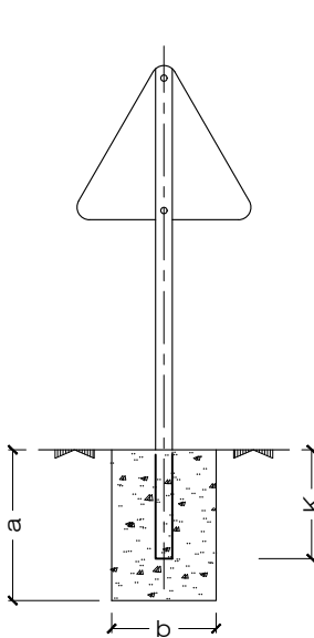
SEÑAL TRIANGULAR
