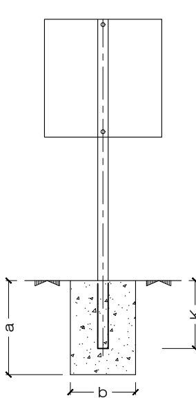
SEÑAL CUADRANGULAR
