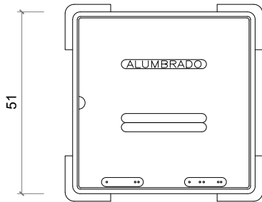
Tapa de registro Fundición ductil 12.5 o 40 tm.
