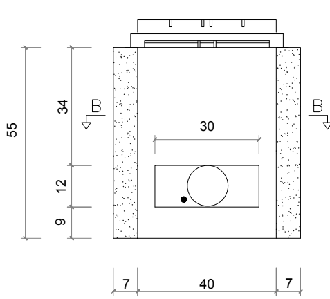
Alzado Sección A-A
