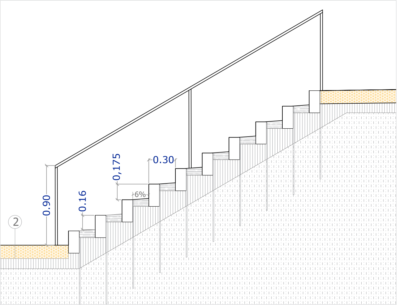
DETALLE 2: SECCIÓN ESCALERA (5 TRAMOS)
