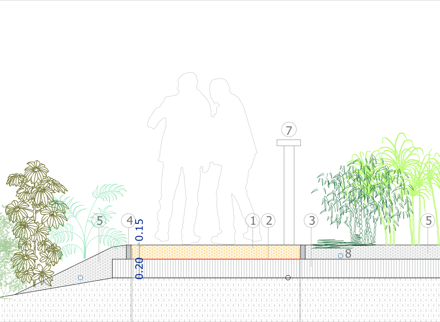
DETALLE 1: SECCIÓN TIPO
