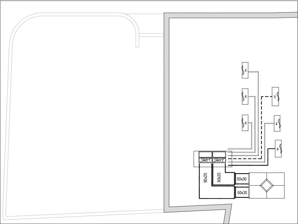
Disposicion maquinas en cubierta
