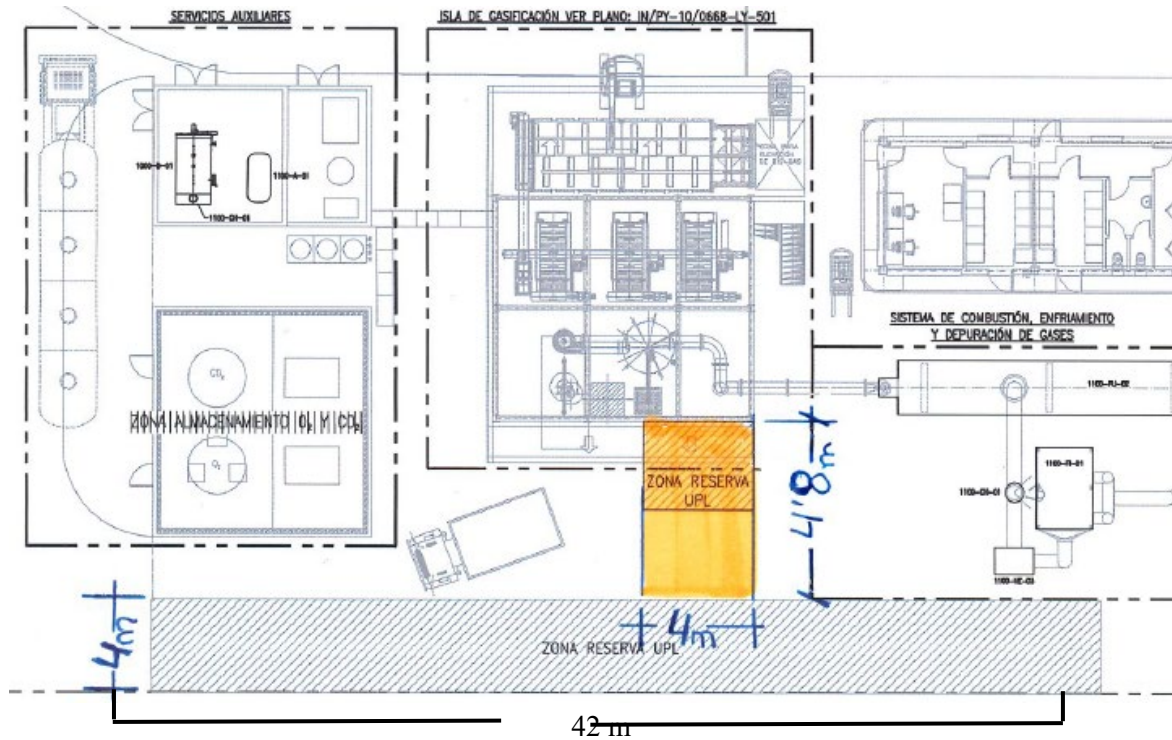
Figura 2. Superficie disponible para la unidad de depuración (marcada en naranja)
