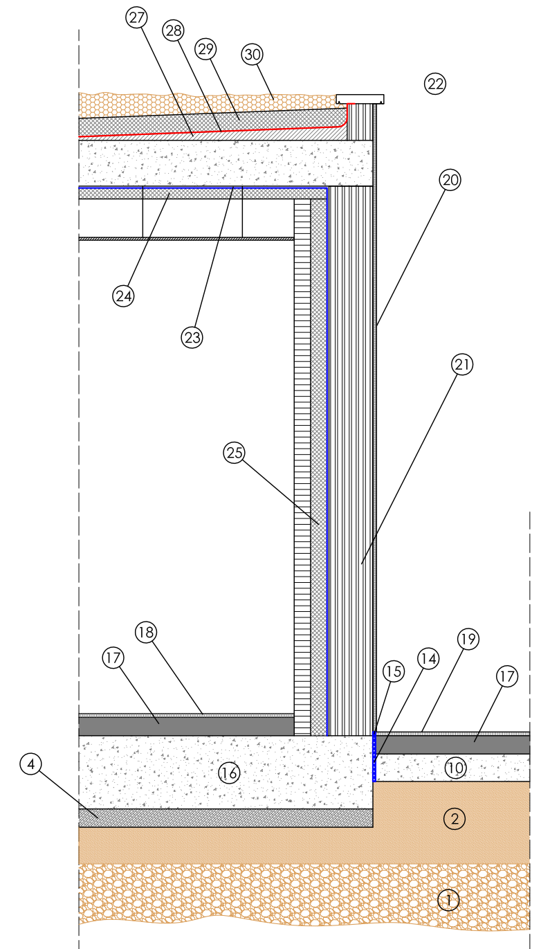
SECCIÓN VERTICAL CASETA
