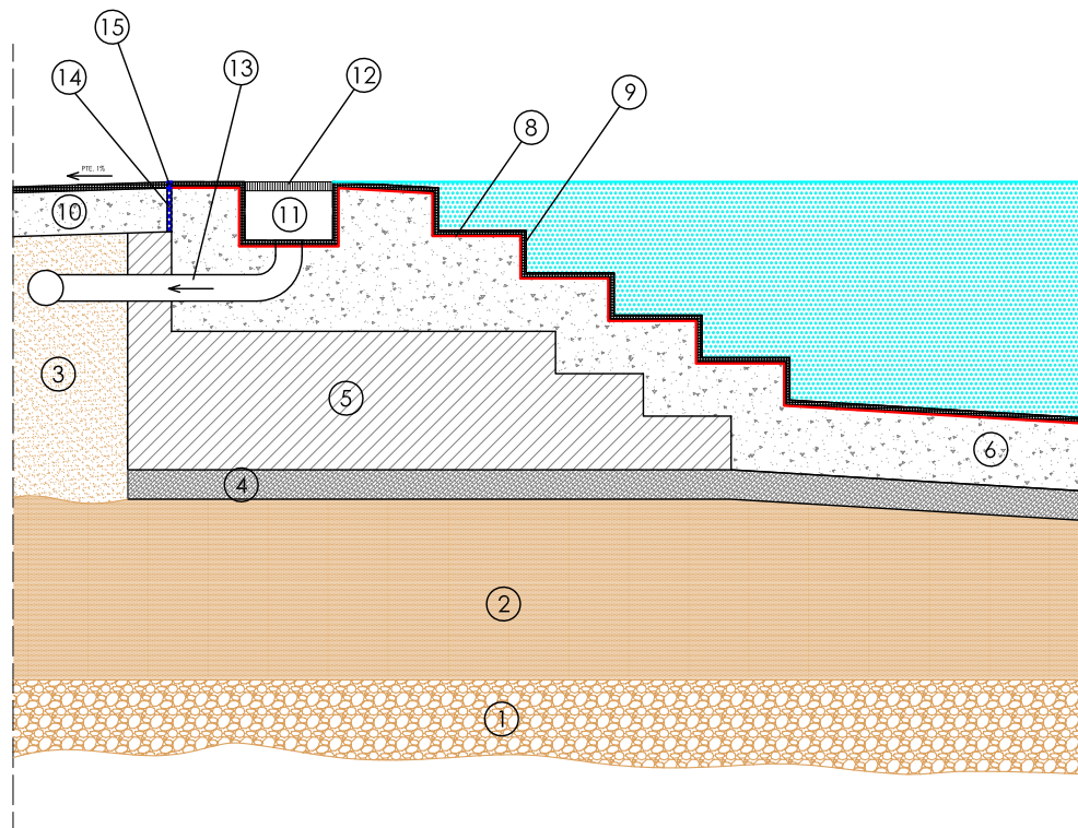
SECCIÓN LONGITUDINAL PISCINA
