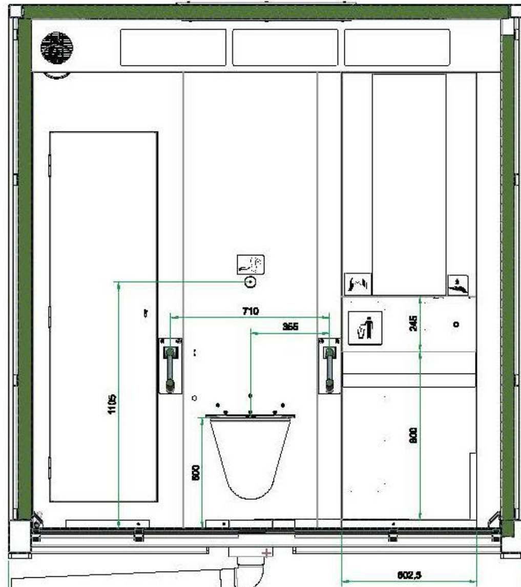
Sección B-B
