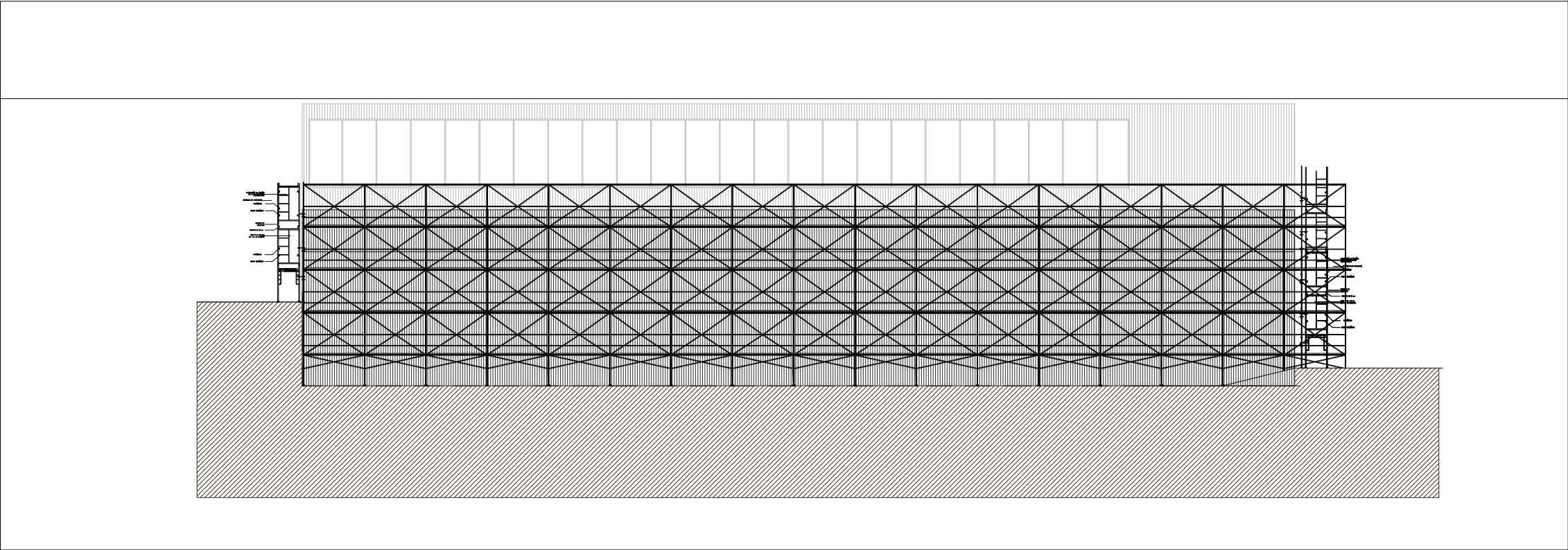
ALZADO NORTE
