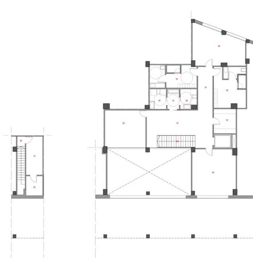
Estado reformado. Entreplanta.
