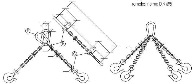
Eslingas de cadena de dos ramales, norma DIN 695
