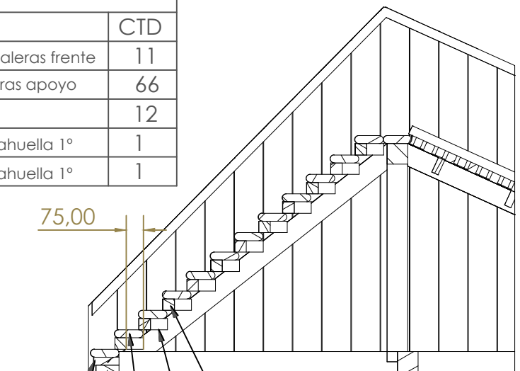
Sección transversal escalera
