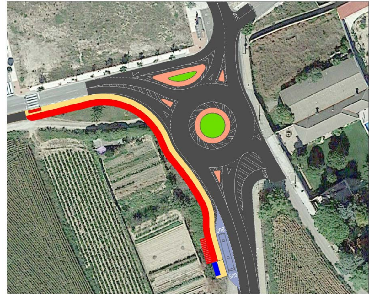
Planta general alternativa seleccionada por el proyecto constructivo
