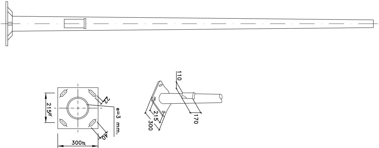
COLUMNA DE 4 m. DE ALTURA
