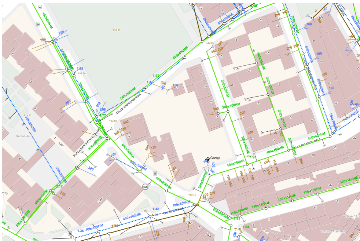
Red de saneamiento existente en la Plaza del Fuero y en su entorno.
