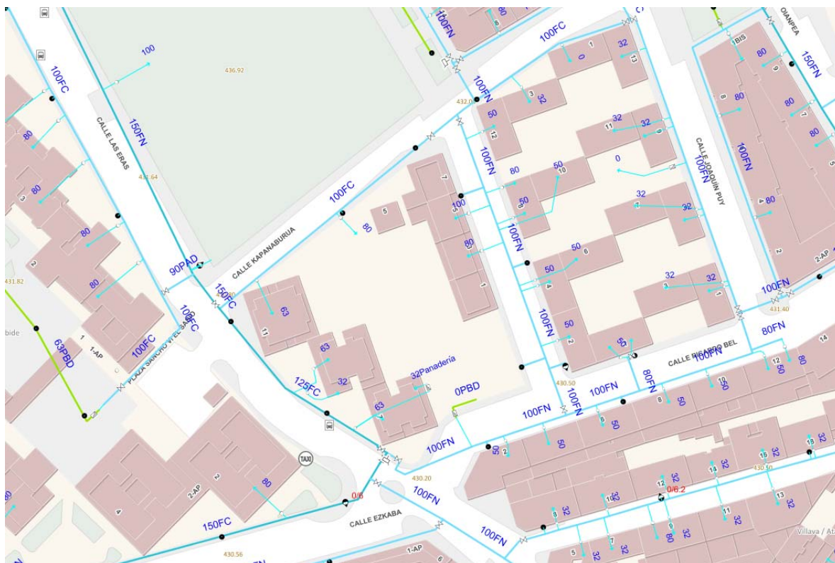
Red de abastecimiento existente en la calle Kapanaburua.
