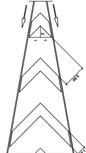
M-7.1.b VIA CON VM > 60 Km/h. CIRCULACION EN SENTIDO UNICO Y DIVERGENTE
