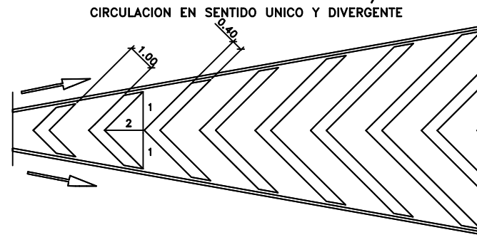
M-7.2.b VIA CON VM ≤ 60Km/h. CIRCULACION EN SENTIDO UNICO Y DIVERGENTE
