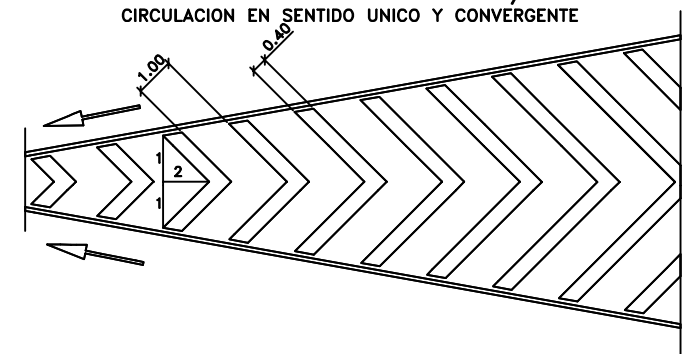
M-7.2.c VIA CON VM ≤ 60Km/h. CIRCULACION EN SENTIDO UNICO Y CONVERGENTE
