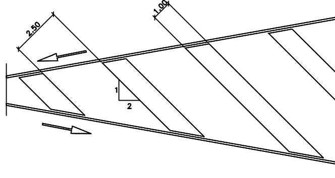
M-7.2.a VIA CON VM ≤ 60Km/h. CIRCULACION EN DOBLE SENTIDO
