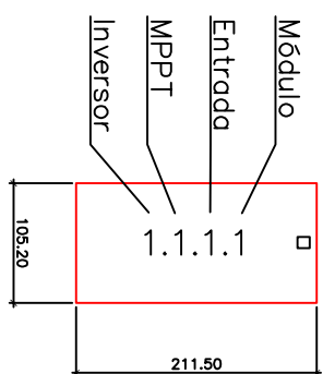
DETALLE MODULO FV
