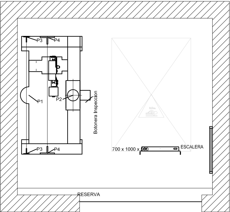
PLANTA DE FOSO
