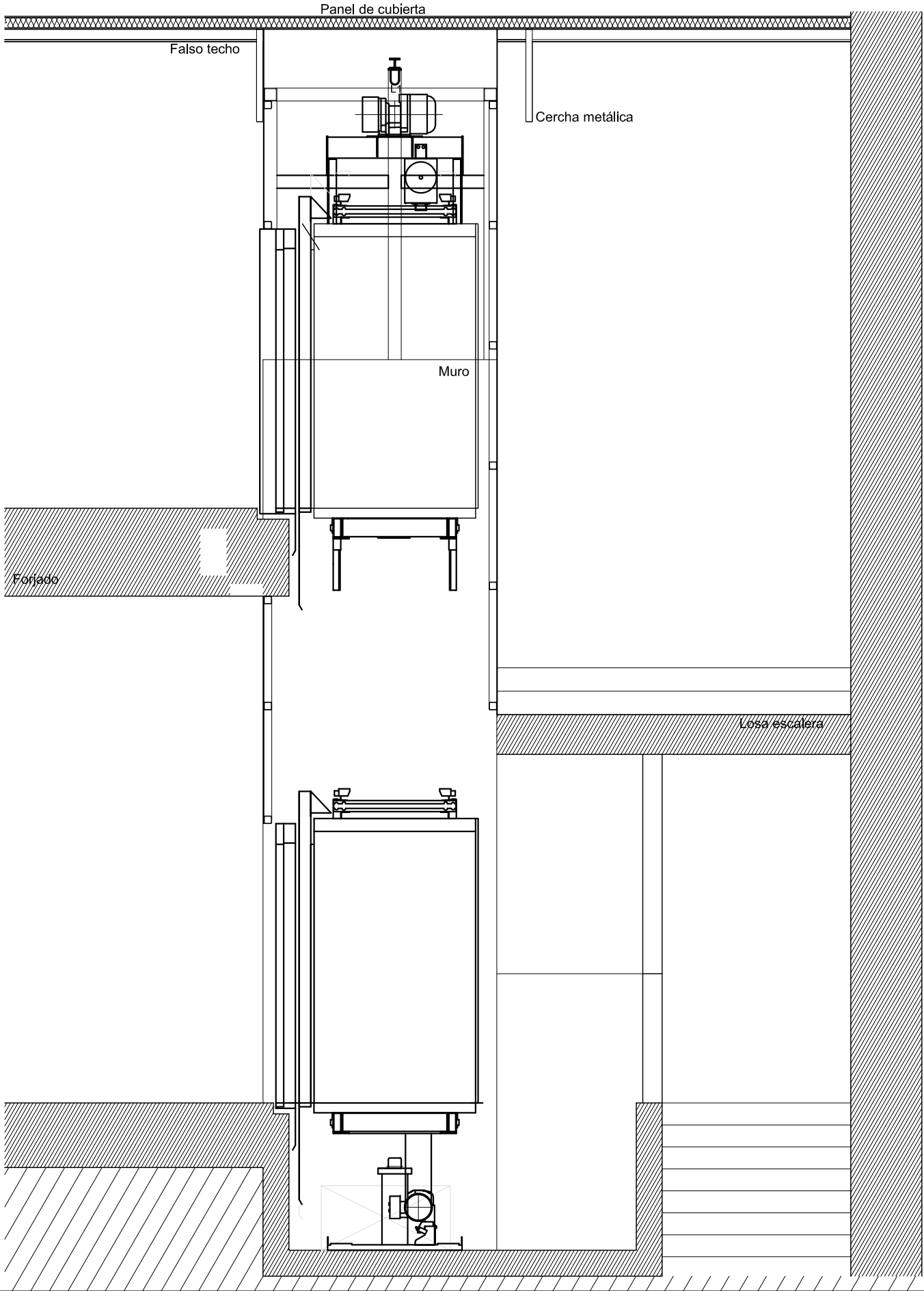
SECCIÓN AA
