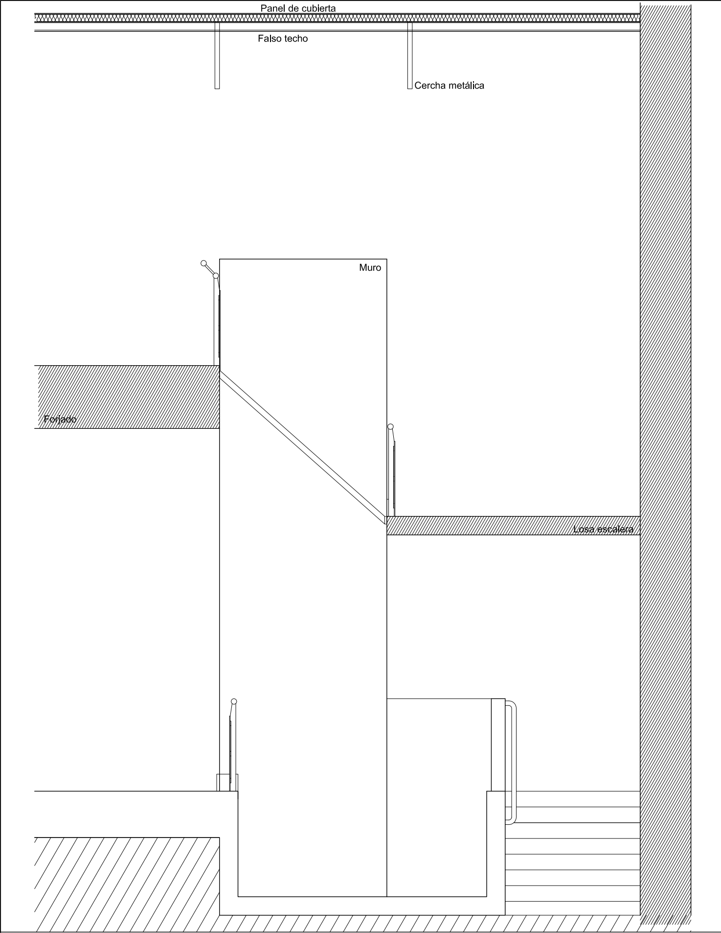
SECCIÓN AA
