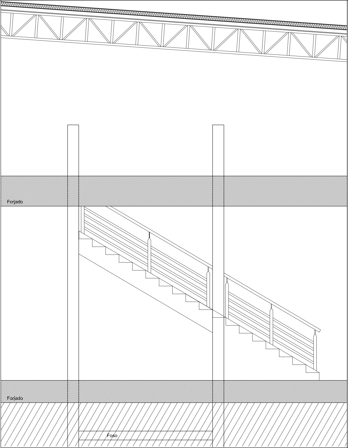
SECCIÓN BB
