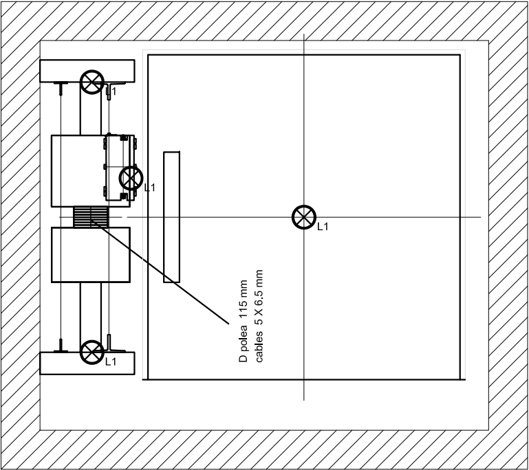
PLANTA DE MÁQUINA
