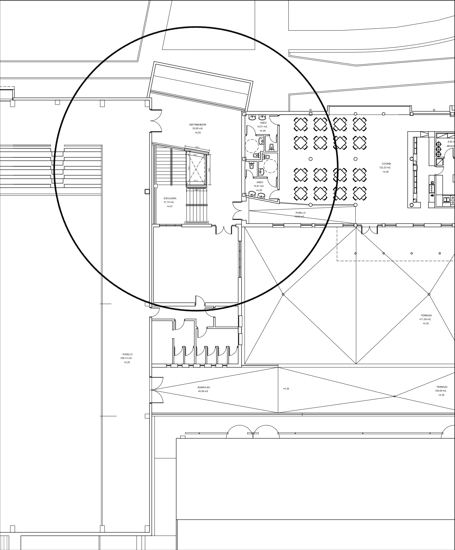
PLANTA PRIMERA
