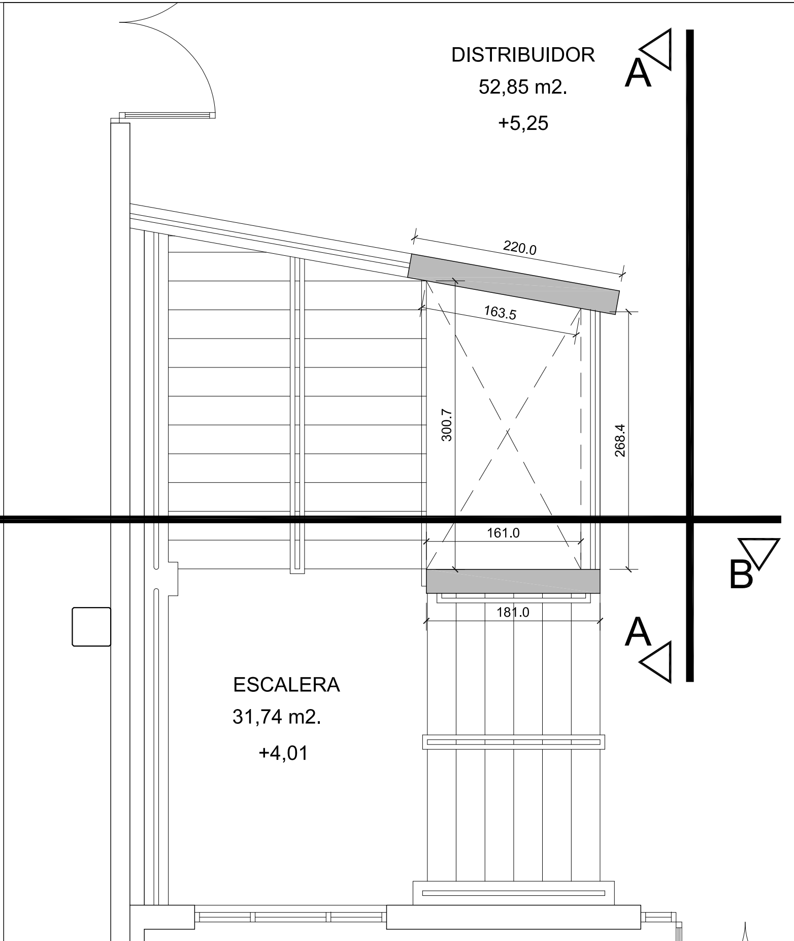
PLANTA PRIMERA
