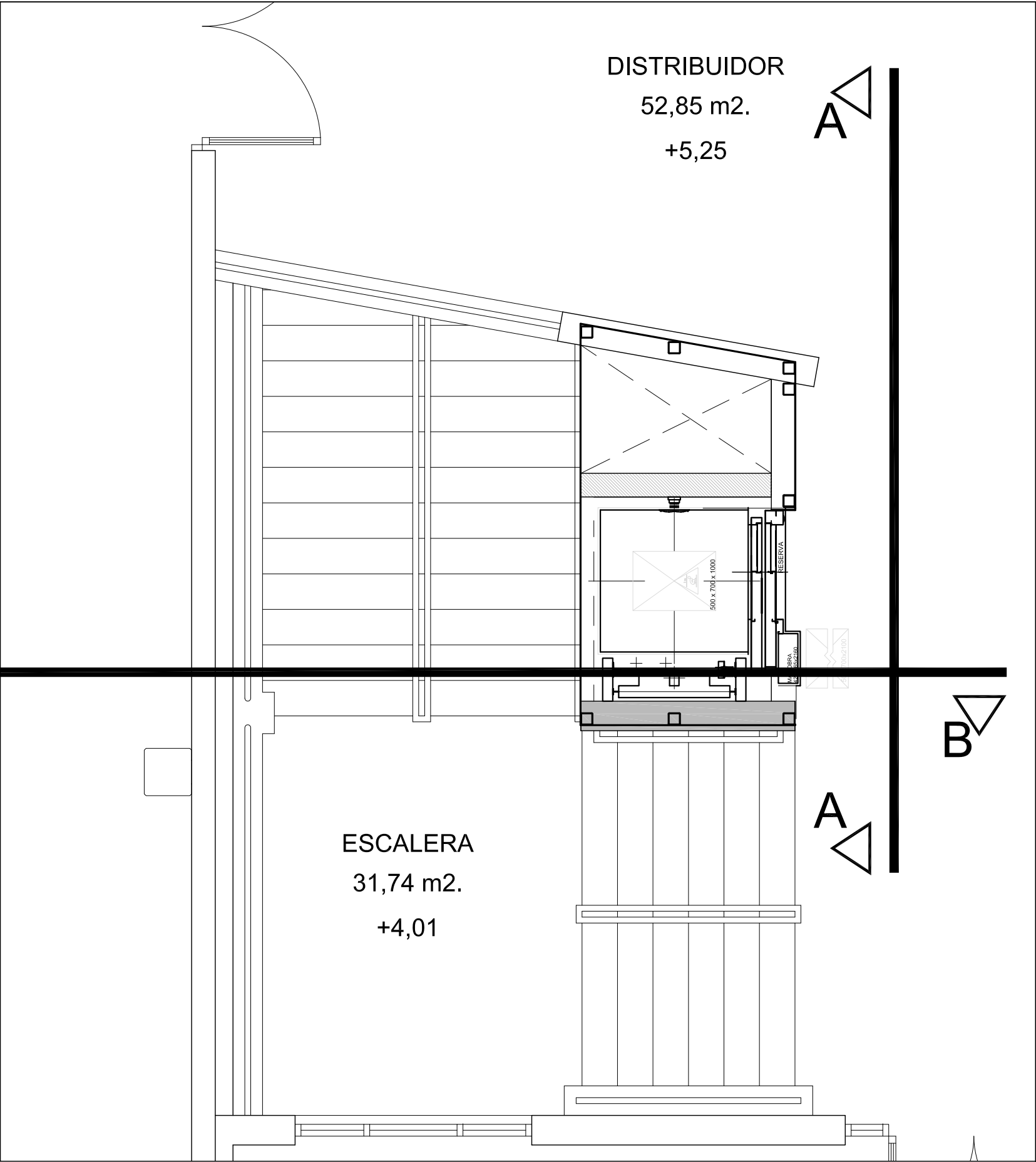
PLANTA PRIMERA
