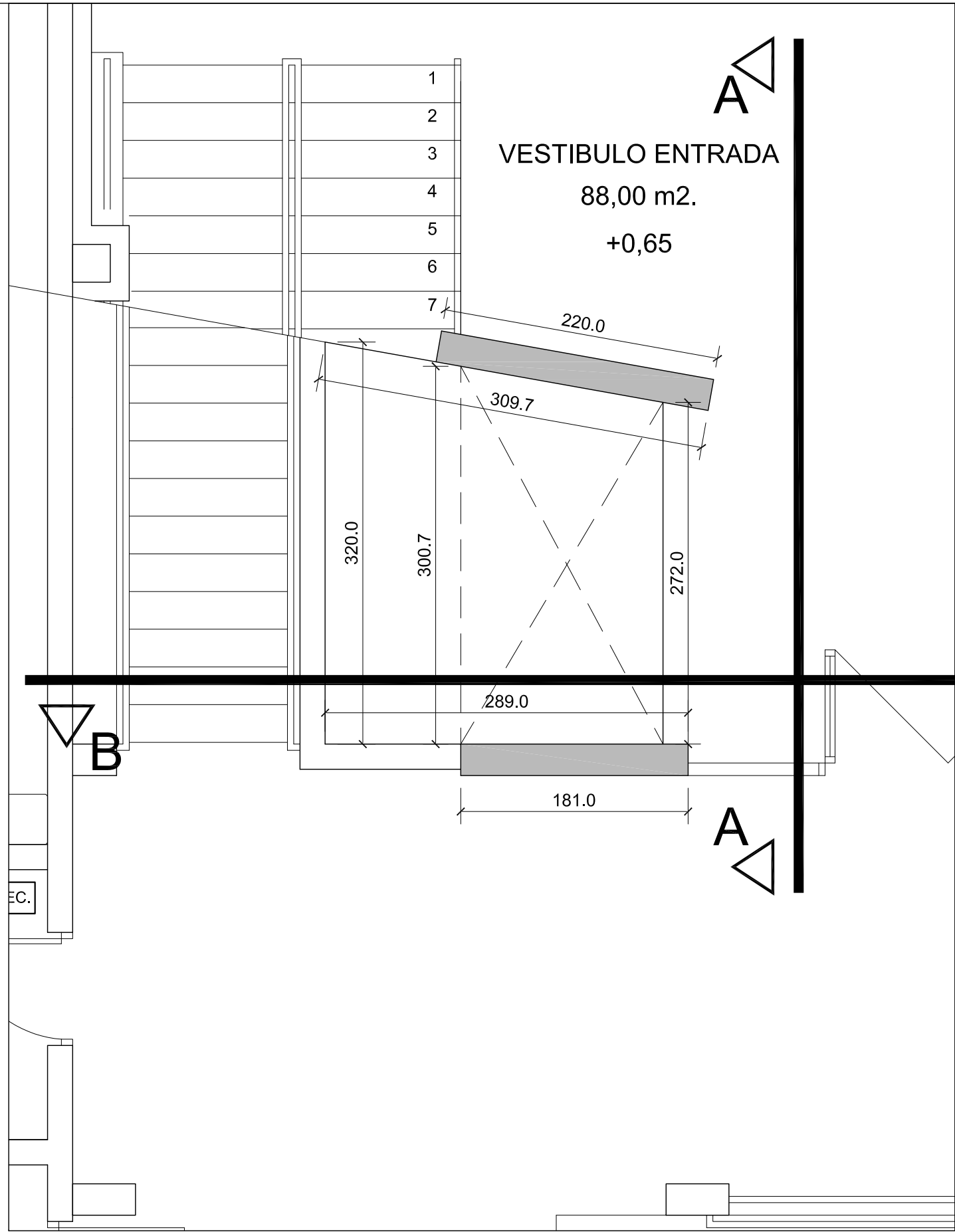
PLANTA BAJA
