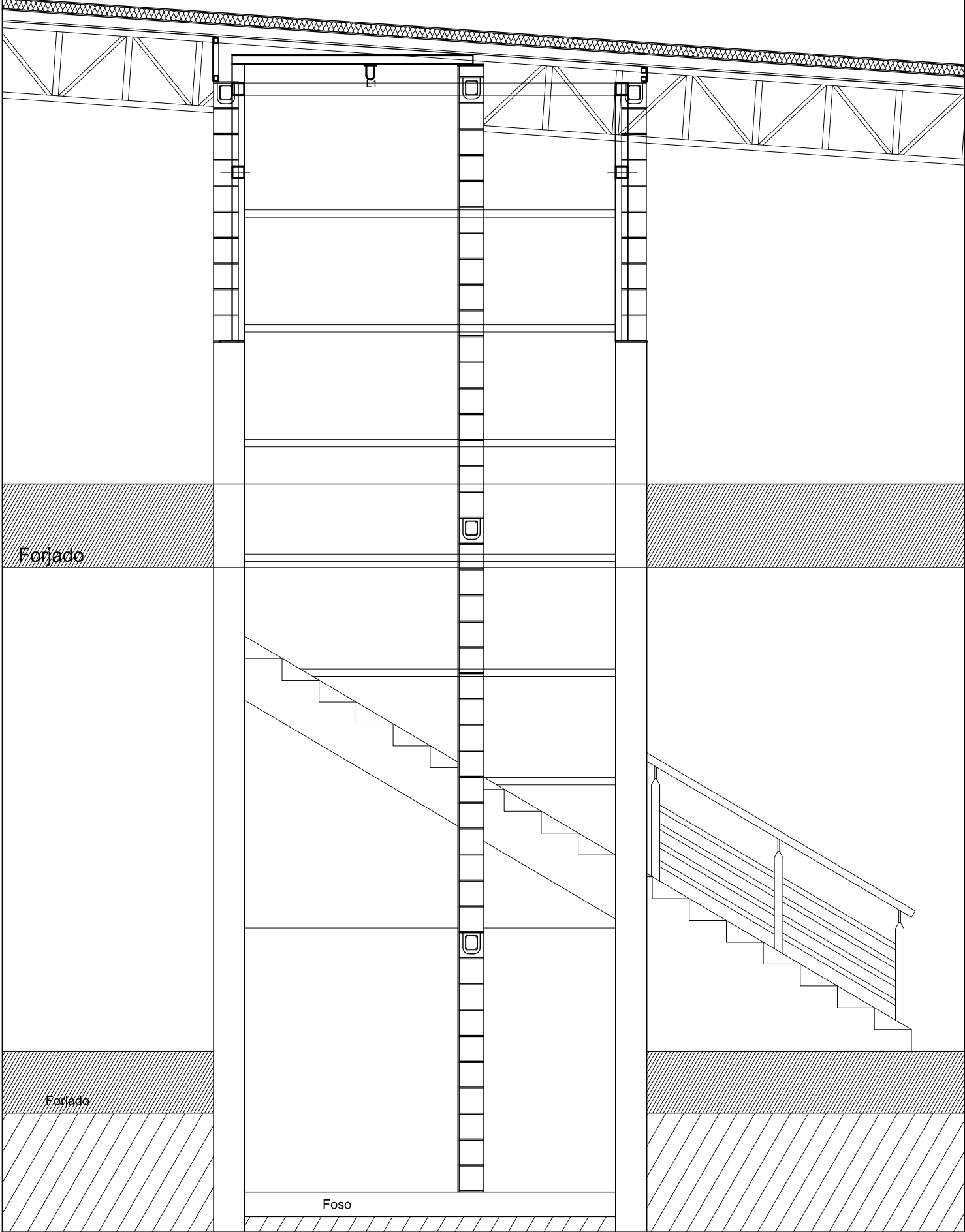
SECCIÓN BB
