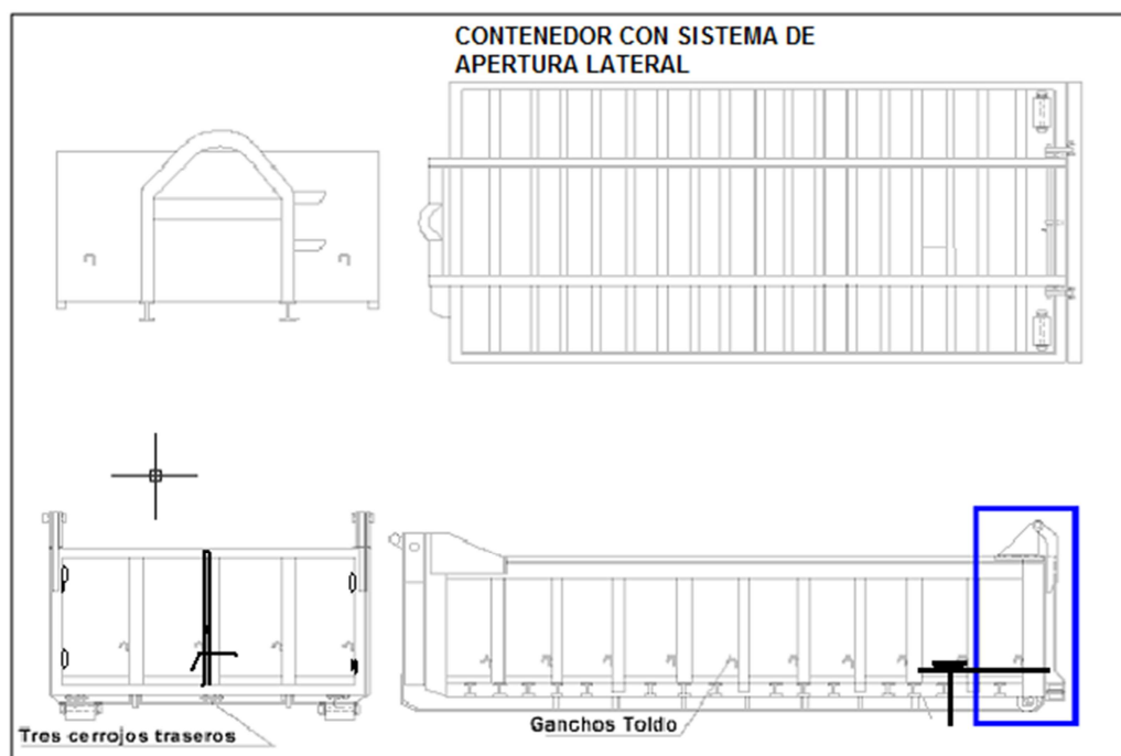
Figura 1: Detalle del sistema de apertura trasera y apertura lateral
