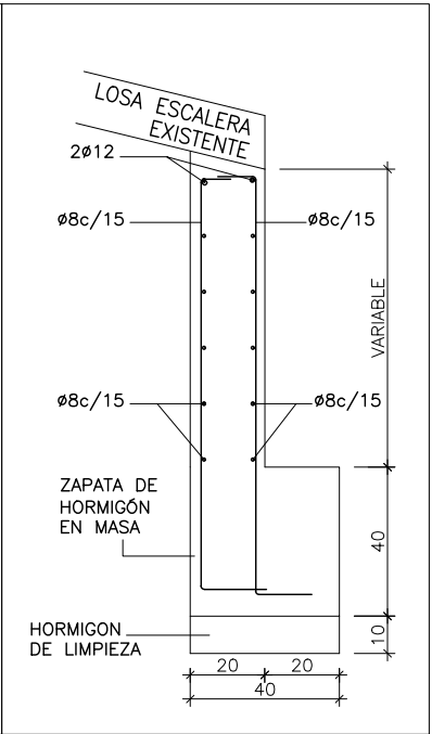
DETALLE MURETE 20cm
