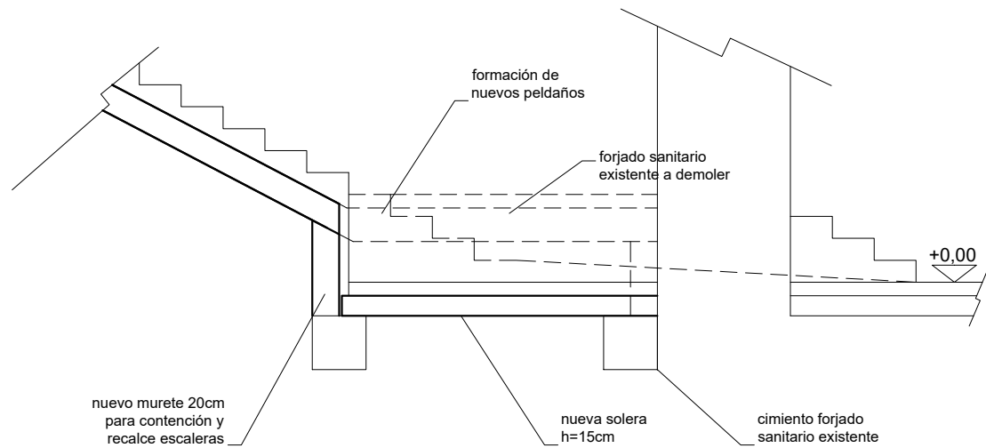
Sección S-3
