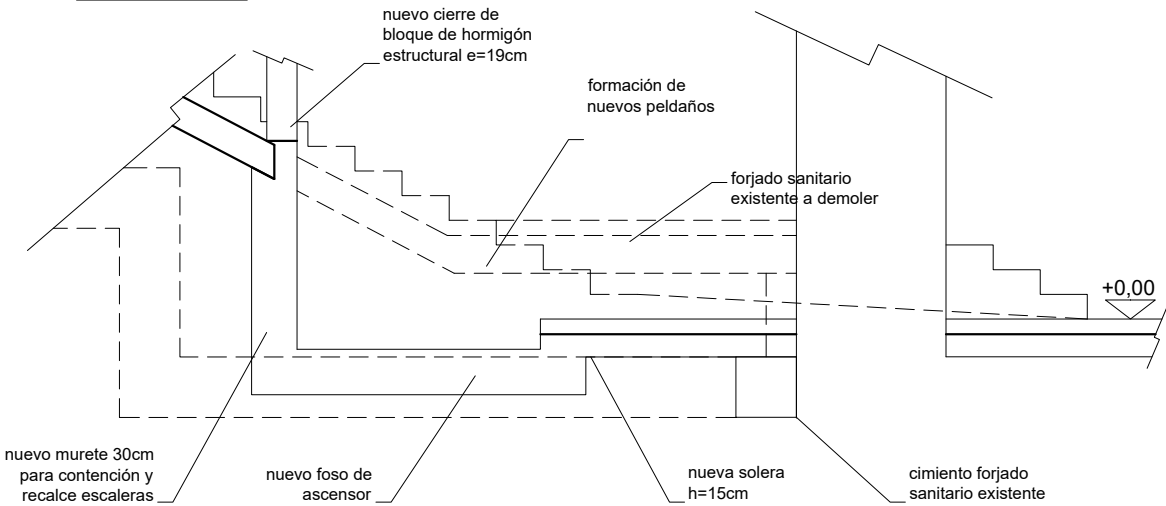
Sección S-2
