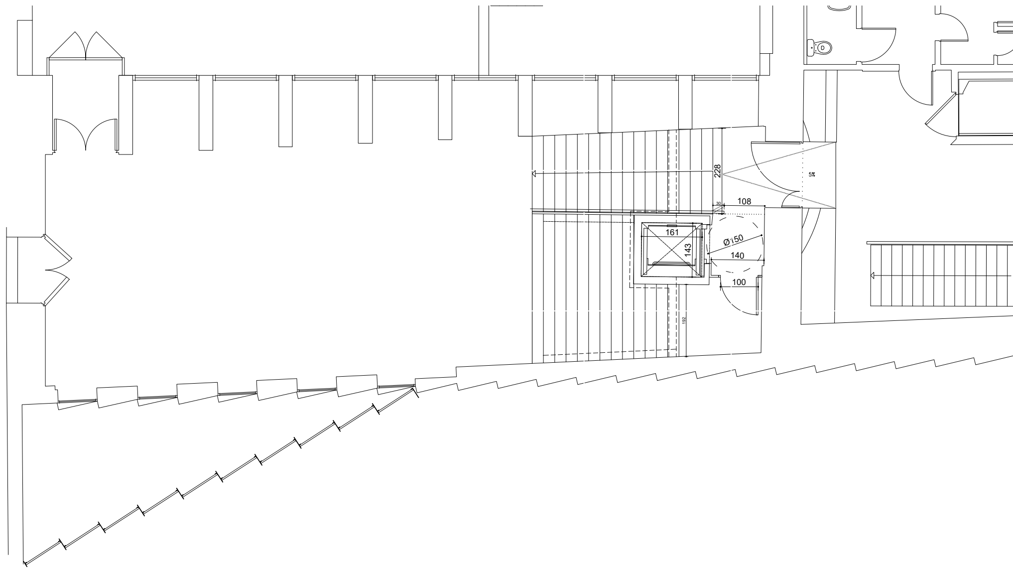
NIVEL +0,00 REFORMADO
