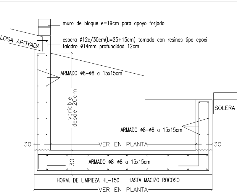
DETALLE FOSO DE ASCENSOR Y MURETE CONTENCIÓN
