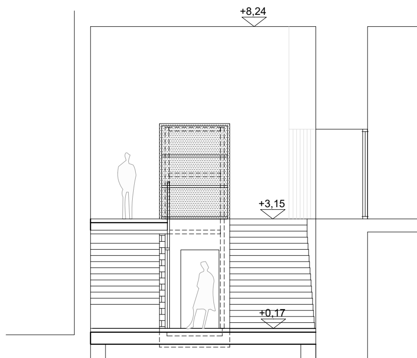
ALZADO FRONTAL ESTADO REFORMADO
