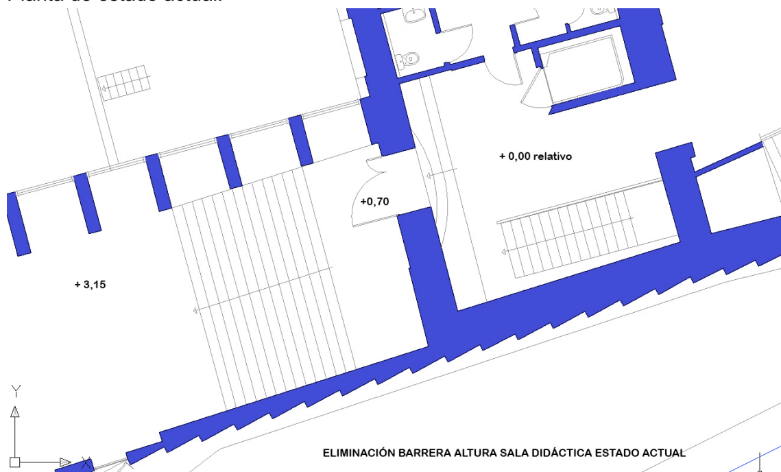
Planta de estado actual.
