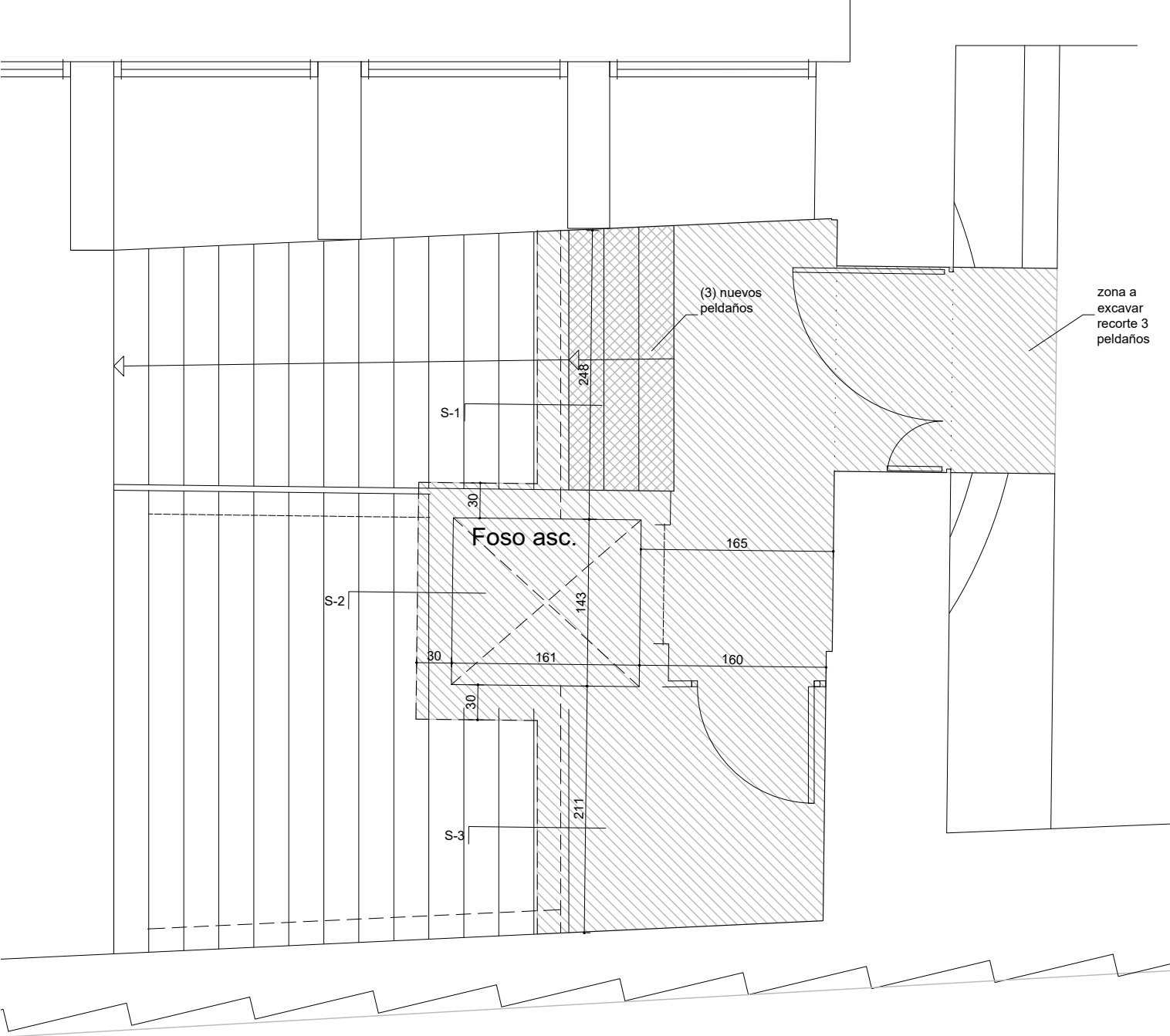
CIMENTACIÓN Y SOLERA (COTA +0,00)
