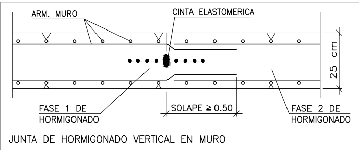
DETALLE ENCUESTRO HORIZONTAL ARMADURAS
