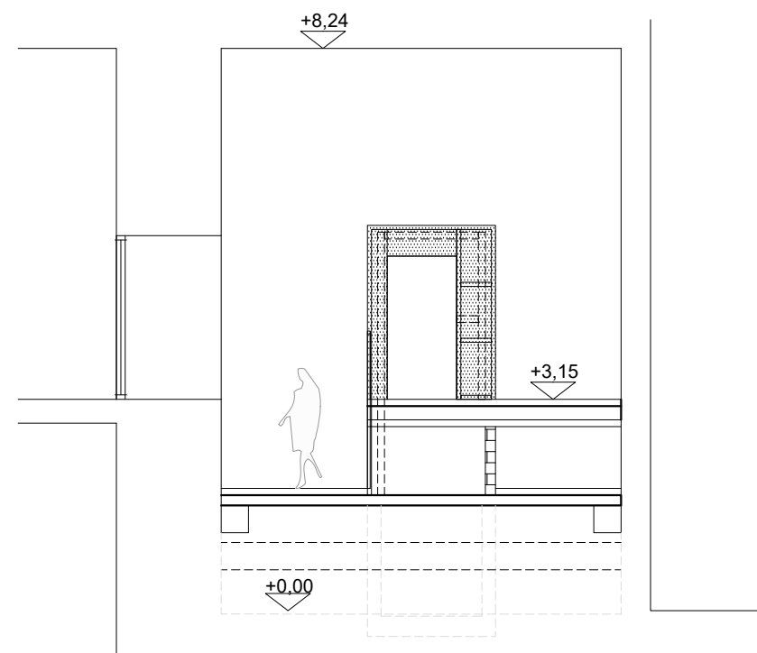
ALZADO TRASERO ESTADO REFORMADO
