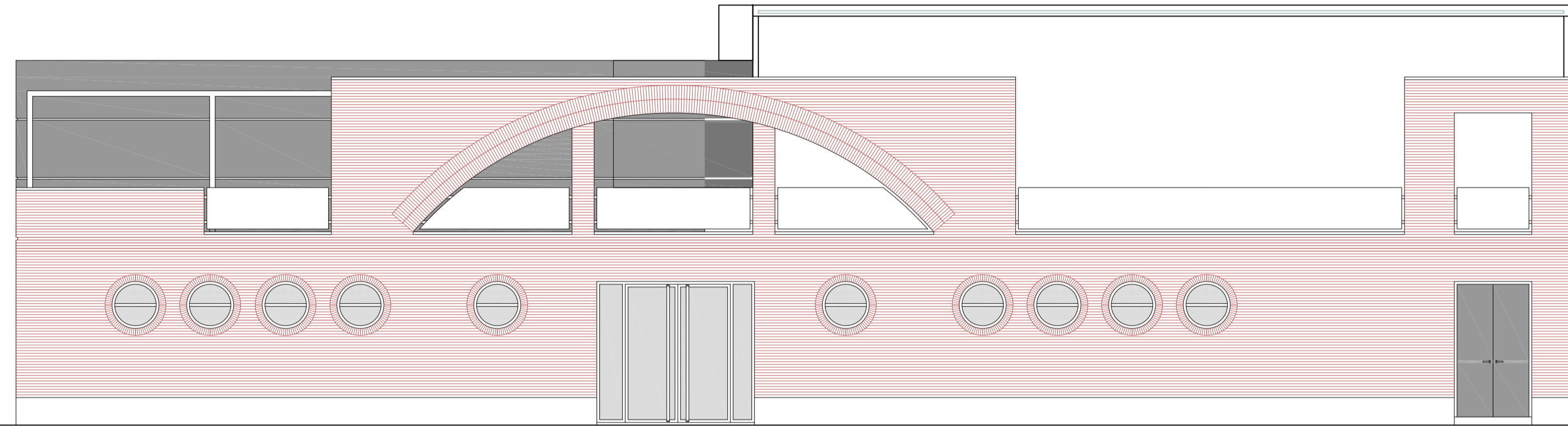
ALZADO C
