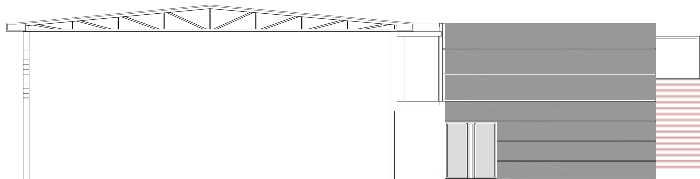
ALZADO D
